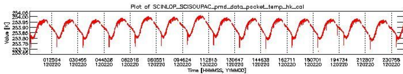
sciamachy_daily_report_level0_KSPT_L0_4504_N_20120220_3.PNG
