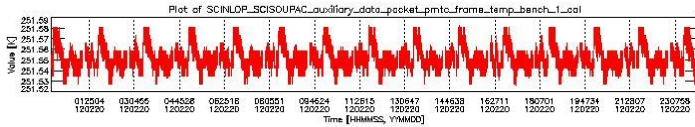
sciamachy_daily_report_level0_KSPT_L0_4504_N_20120220_0.PNG
