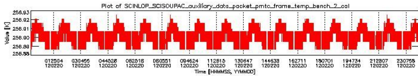
sciamachy_daily_report_level0_KSPT_L0_4504_N_20120220_1.PNG
