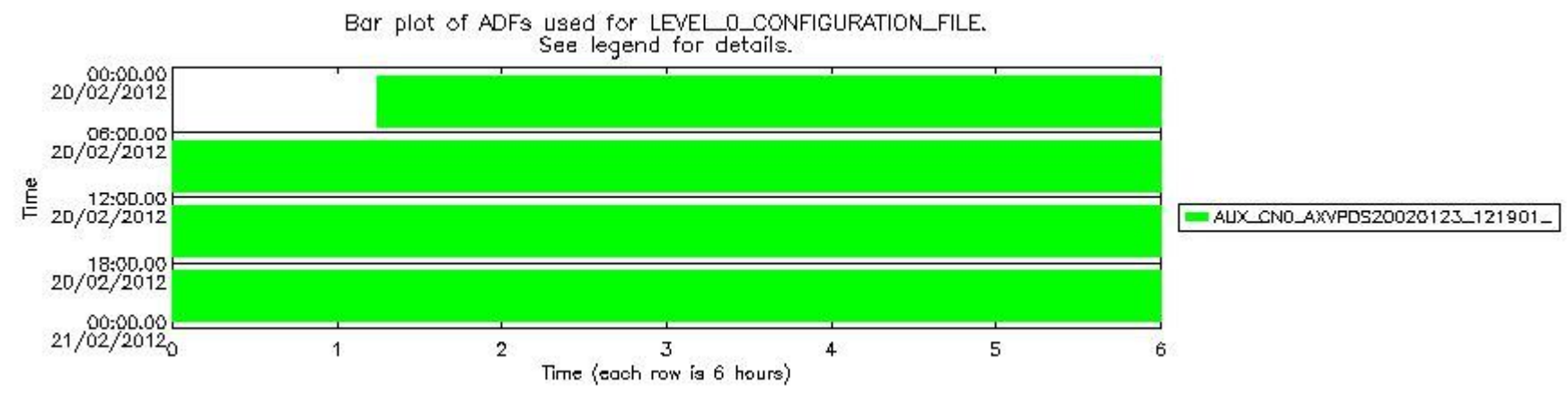
sciamachy_daily_report_level0_KSPT_L0_4504_N_20120220_6.PNG
