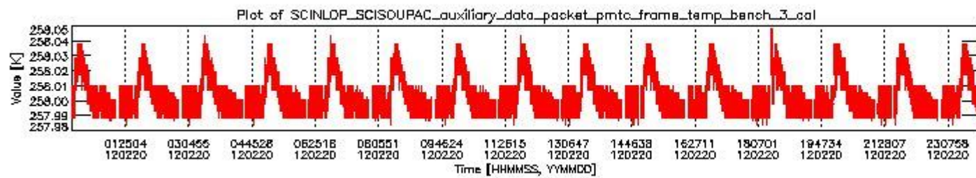
sciamachy_daily_report_level0_KSPT_L0_4504_N_20120220_2.PNG
