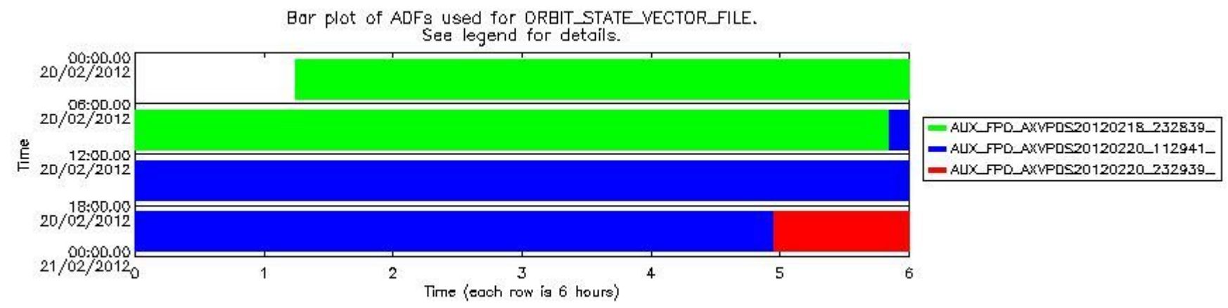
sciamachy_daily_report_level0_KSPT_L0_4504_N_20120220_7.PNG
