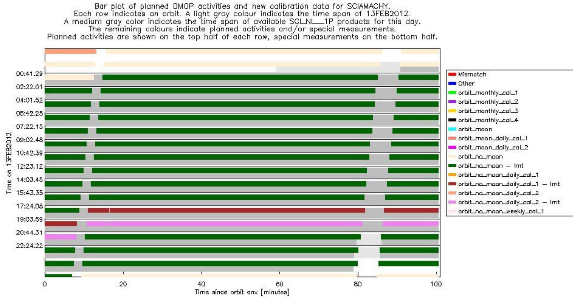
sciamachy_daily_report_level0_KSPT_L0_4504_N_20120213_5.PNG
