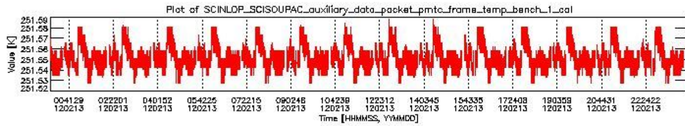
sciamachy_daily_report_level0_KSPT_L0_4504_N_20120213_0.PNG
