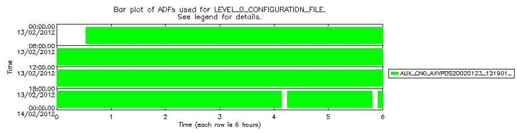
sciamachy_daily_report_level0_KSPT_L0_4504_N_20120213_6.PNG
