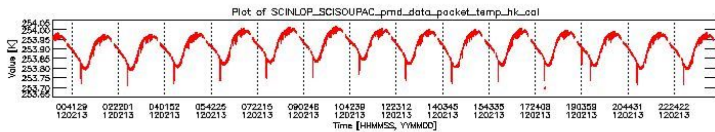
sciamachy_daily_report_level0_KSPT_L0_4504_N_20120213_3.PNG
