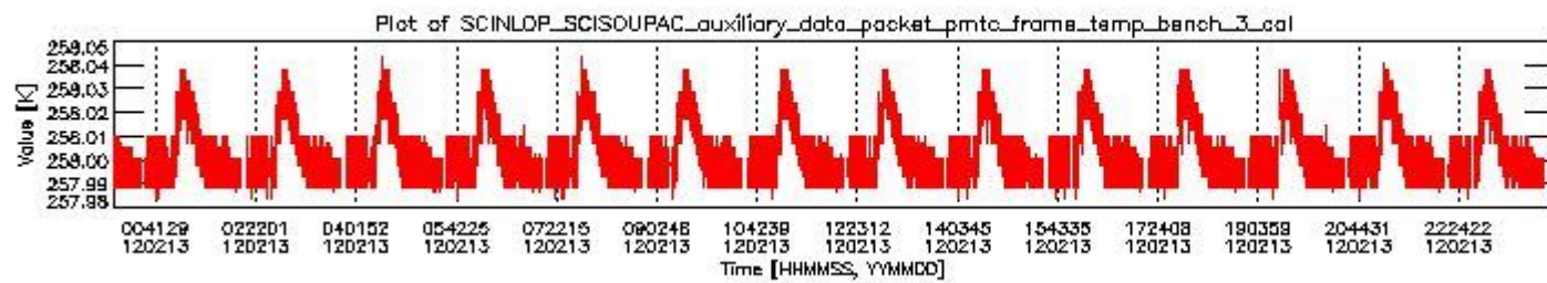
sciamachy_daily_report_level0_KSPT_L0_4504_N_20120213_2.PNG
