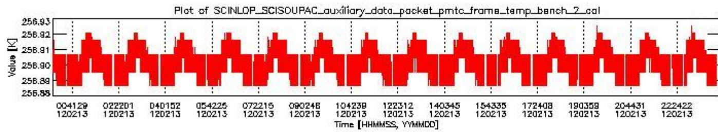
sciamachy_daily_report_level0_KSPT_L0_4504_N_20120213_1.PNG
