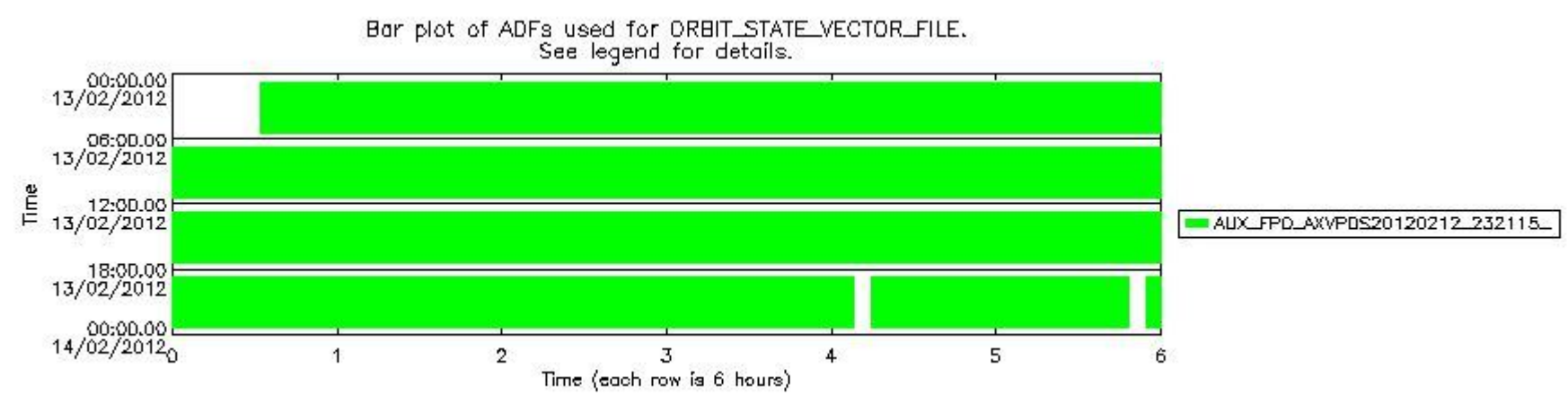
sciamachy_daily_report_level0_KSPT_L0_4504_N_20120213_7.PNG
