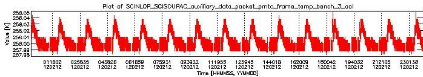
sciamachy_daily_report_level0_KSPT_L0_4504_N_20120212_2.PNG
