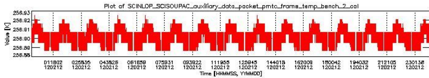
sciamachy_daily_report_level0_KSPT_L0_4504_N_20120212_1.PNG
