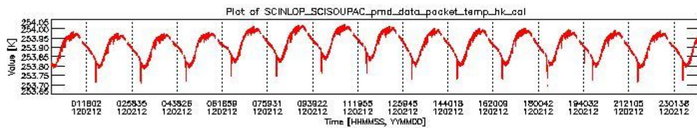
sciamachy_daily_report_level0_KSPT_L0_4504_N_20120212_3.PNG
