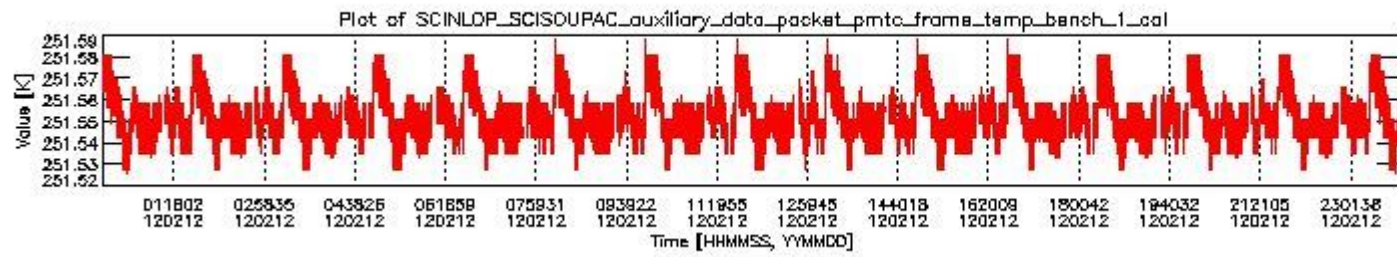
sciamachy_daily_report_level0_KSPT_L0_4504_N_20120212_0.PNG
