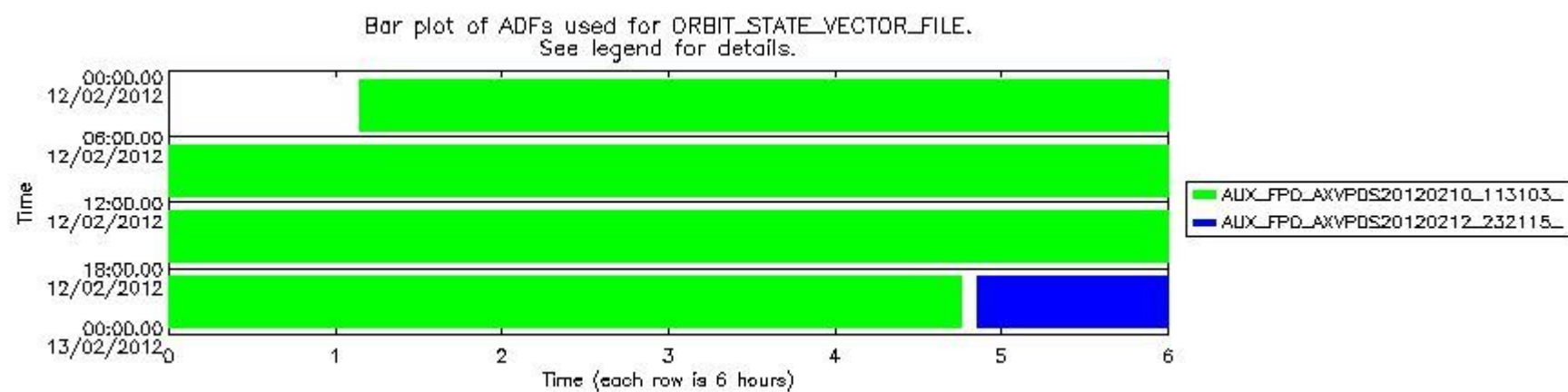
sciamachy_daily_report_level0_KSPT_L0_4504_N_20120212_7.PNG
