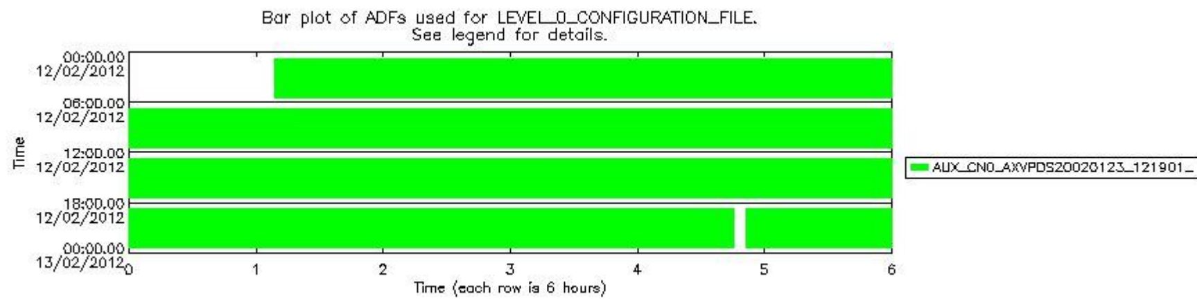
sciamachy_daily_report_level0_KSPT_L0_4504_N_20120212_6.PNG
