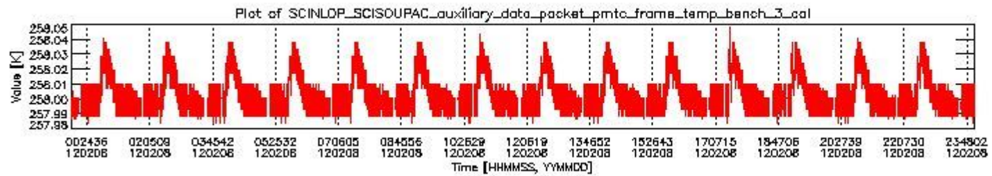
sciamachy_daily_report_level0_KSPT_L0_4504_N_20120208_2.PNG
