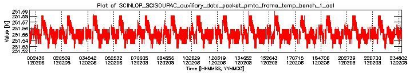
sciamachy_daily_report_level0_KSPT_L0_4504_N_20120208_0.PNG
