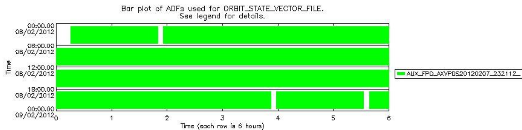
sciamachy_daily_report_level0_KSPT_L0_4504_N_20120208_7.PNG
