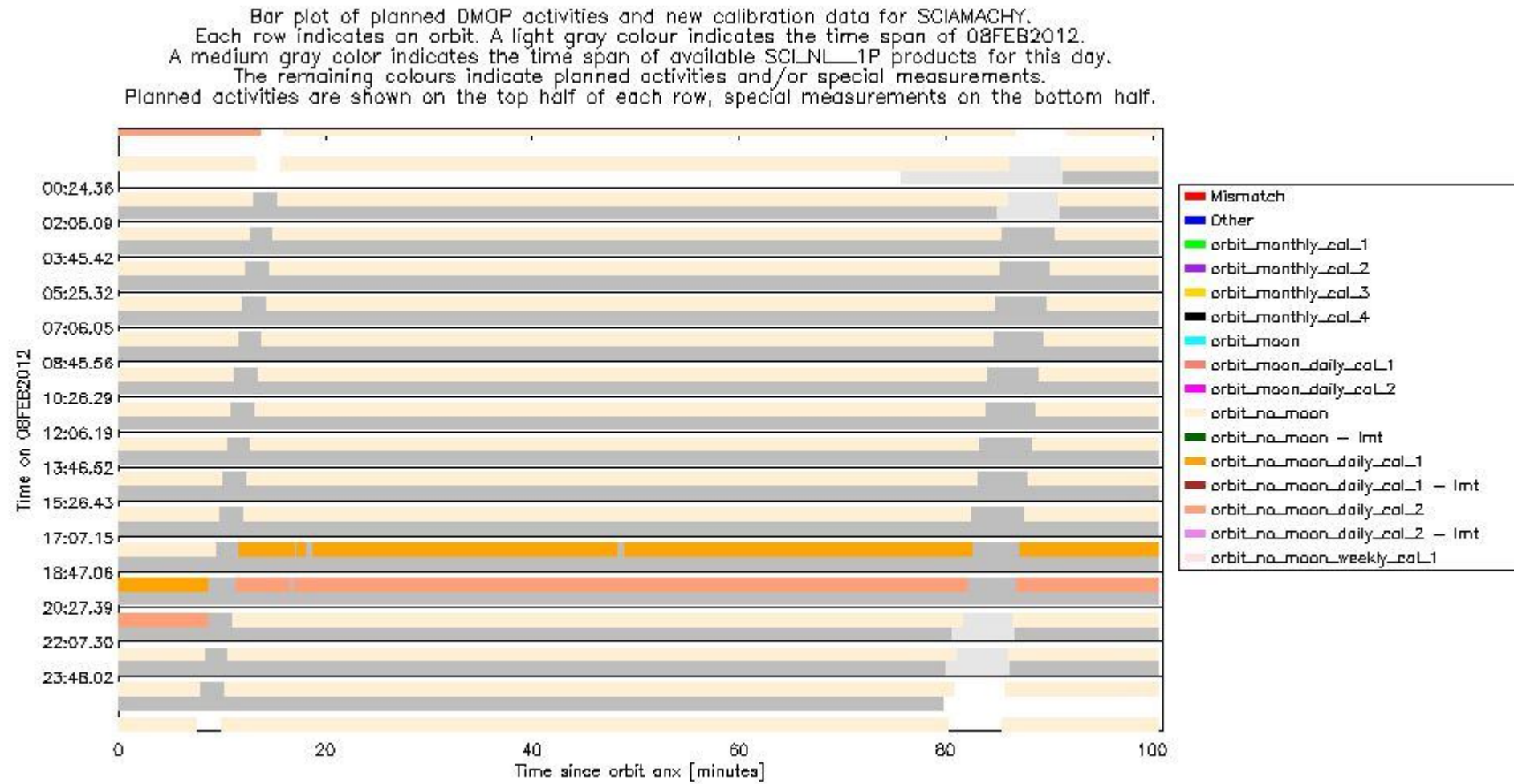
sciamachy_daily_report_level0_KSPT_L0_4504_N_20120208_5.PNG
