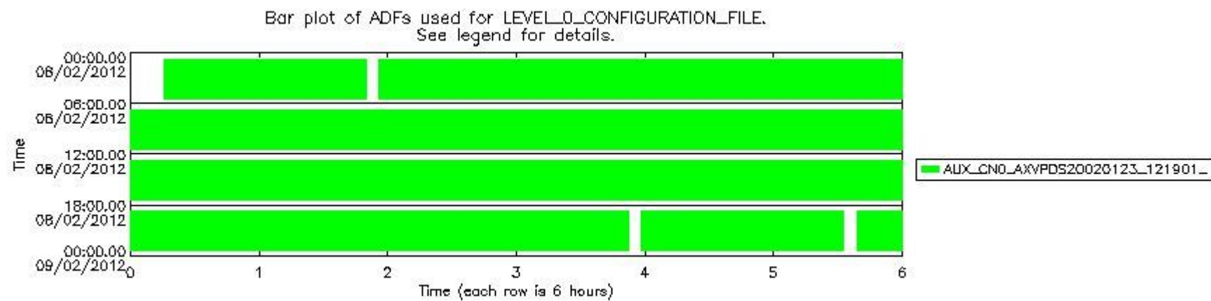
sciamachy_daily_report_level0_KSPT_L0_4504_N_20120208_6.PNG
