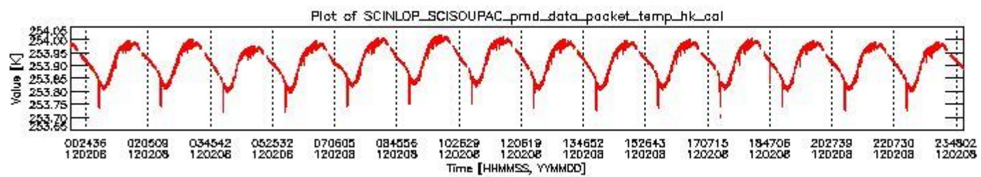
sciamachy_daily_report_level0_KSPT_L0_4504_N_20120208_3.PNG
