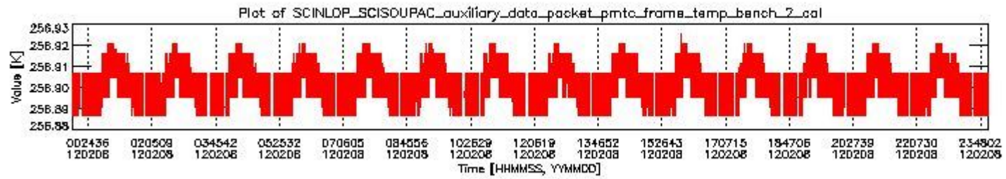
sciamachy_daily_report_level0_KSPT_L0_4504_N_20120208_1.PNG
