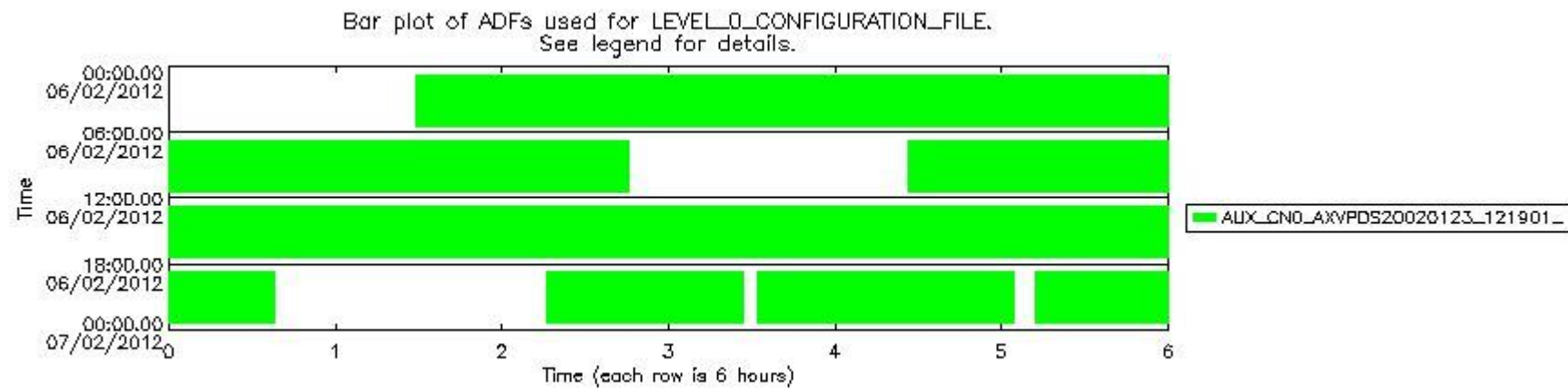
sciamachy_daily_report_level0_KSPT_L0_4504_N_20120206_6.PNG
