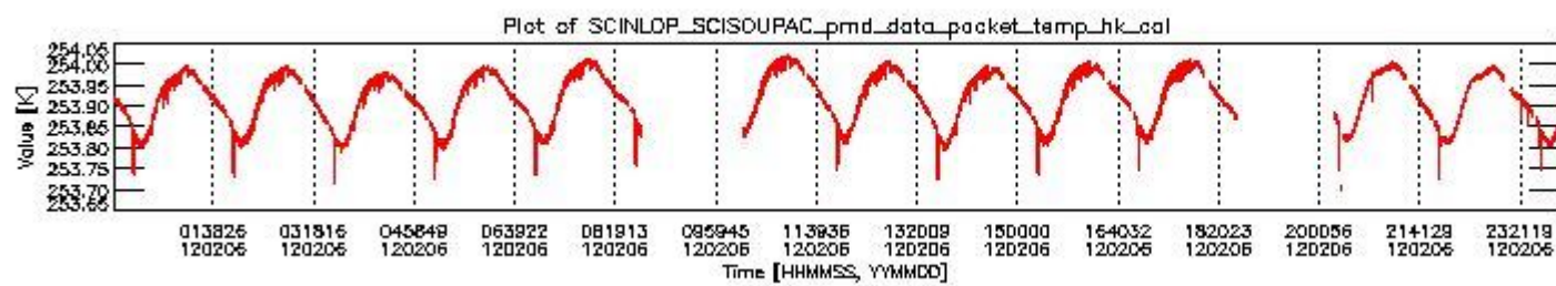
sciamachy_daily_report_level0_KSPT_L0_4504_N_20120206_3.PNG
