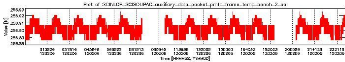
sciamachy_daily_report_level0_KSPT_L0_4504_N_20120206_1.PNG
