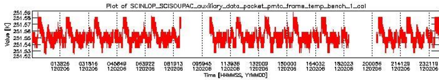
sciamachy_daily_report_level0_KSPT_L0_4504_N_20120206_0.PNG
