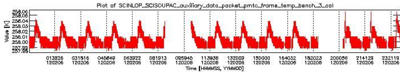
sciamachy_daily_report_level0_KSPT_L0_4504_N_20120206_2.PNG
