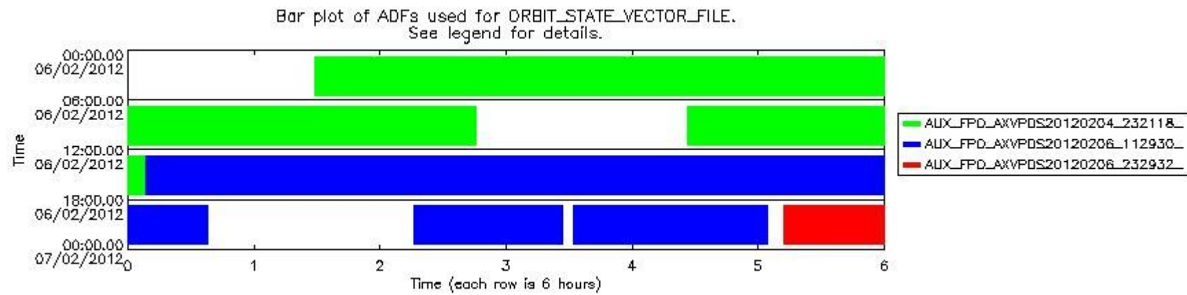
sciamachy_daily_report_level0_KSPT_L0_4504_N_20120206_7.PNG
