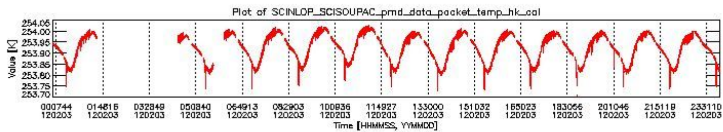
sciamachy_daily_report_level0_KSPT_L0_4504_N_20120203_3.PNG
