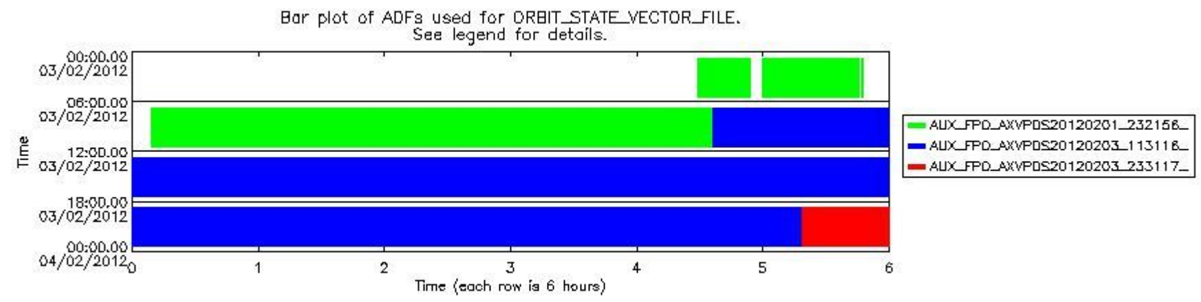
sciamachy_daily_report_level0_KSPT_L0_4504_N_20120203_7.PNG
