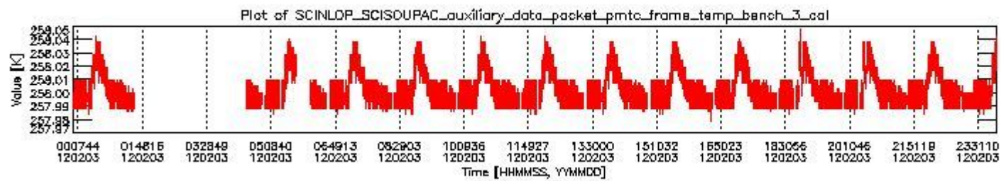
sciamachy_daily_report_level0_KSPT_L0_4504_N_20120203_2.PNG
