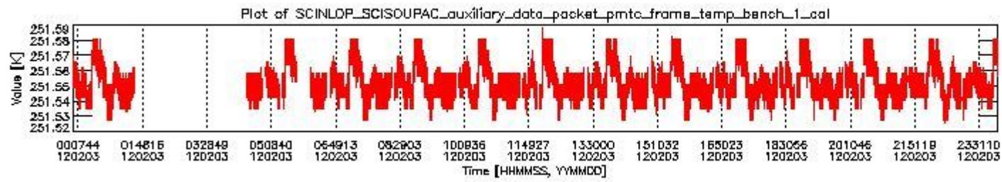
sciamachy_daily_report_level0_KSPT_L0_4504_N_20120203_0.PNG
