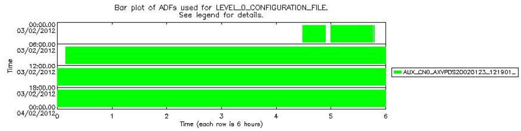
sciamachy_daily_report_level0_KSPT_L0_4504_N_20120203_6.PNG
