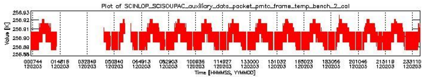
sciamachy_daily_report_level0_KSPT_L0_4504_N_20120203_1.PNG
