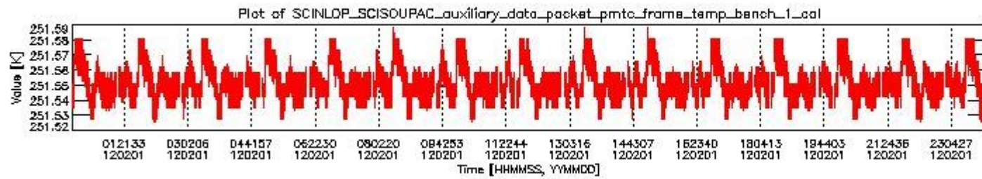
sciamachy_daily_report_level0_KSPT_L0_4504_N_20120201_0.PNG
