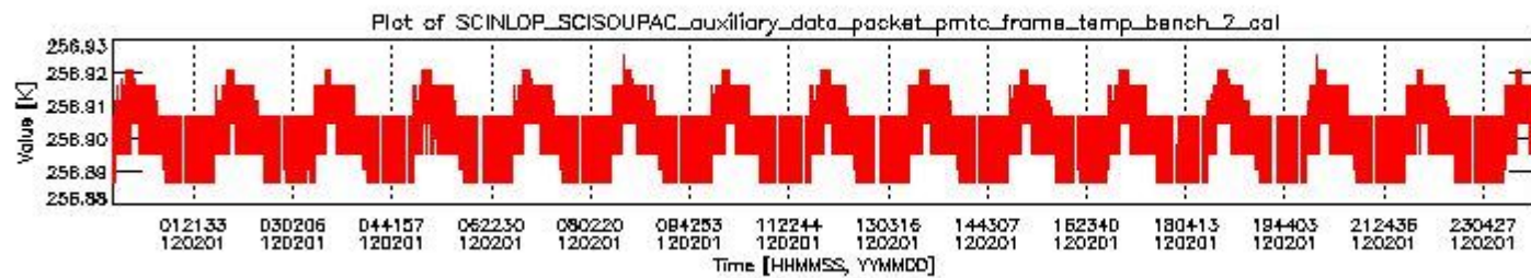
sciamachy_daily_report_level0_KSPT_L0_4504_N_20120201_1.PNG
