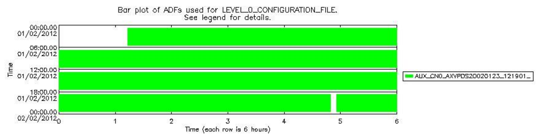
sciamachy_daily_report_level0_KSPT_L0_4504_N_20120201_6.PNG
