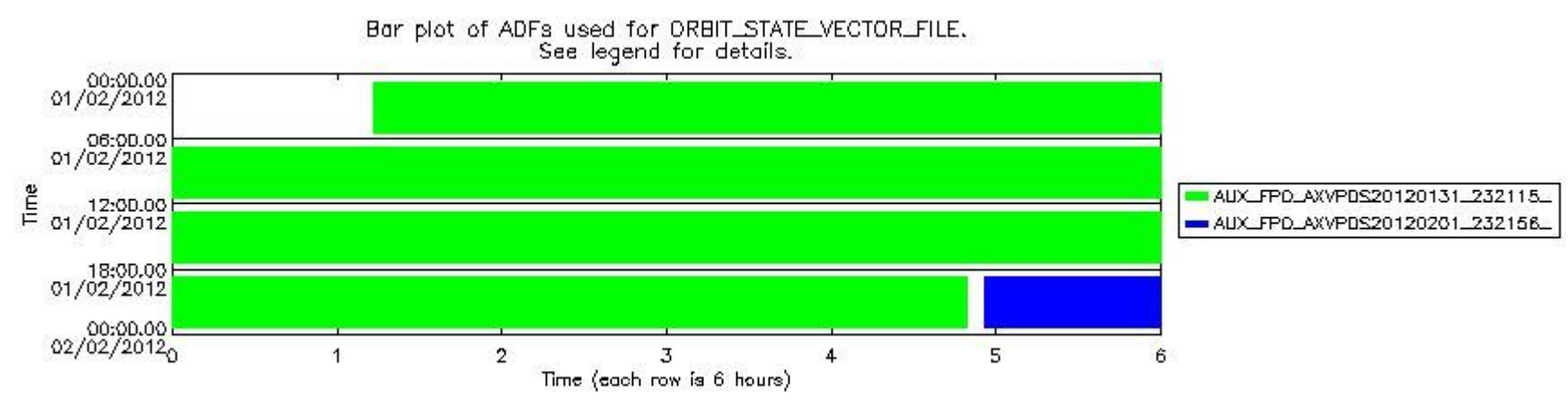
sciamachy_daily_report_level0_KSPT_L0_4504_N_20120201_7.PNG
