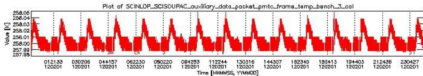
sciamachy_daily_report_level0_KSPT_L0_4504_N_20120201_2.PNG
