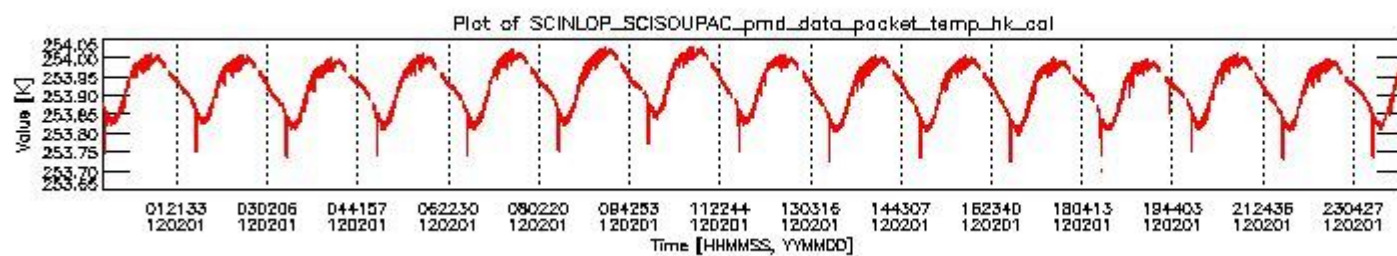
sciamachy_daily_report_level0_KSPT_L0_4504_N_20120201_3.PNG
