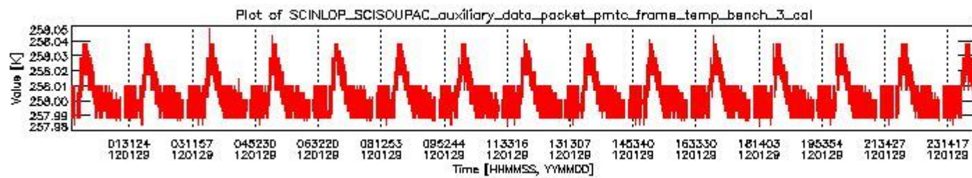
sciamachy_daily_report_level0_KSPT_L0_4504_N_20120129_2.PNG
