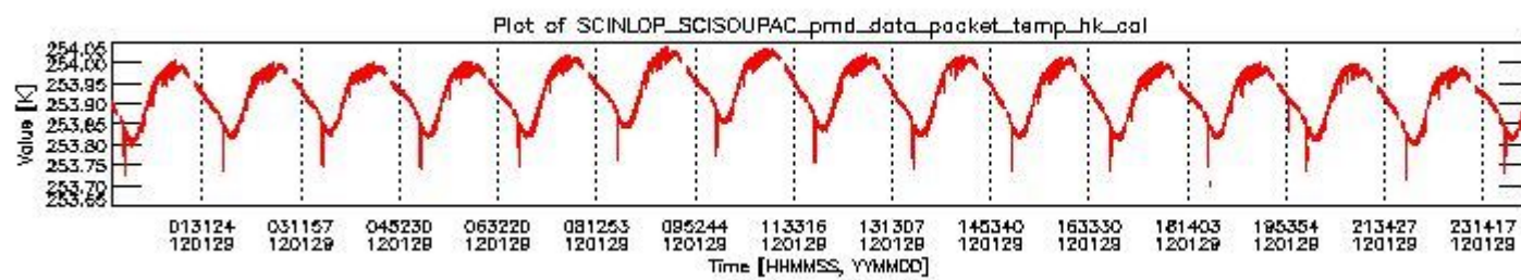
sciamachy_daily_report_level0_KSPT_L0_4504_N_20120129_3.PNG
