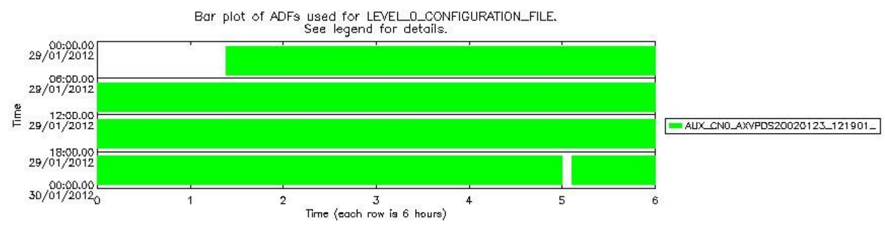
sciamachy_daily_report_level0_KSPT_L0_4504_N_20120129_6.PNG
