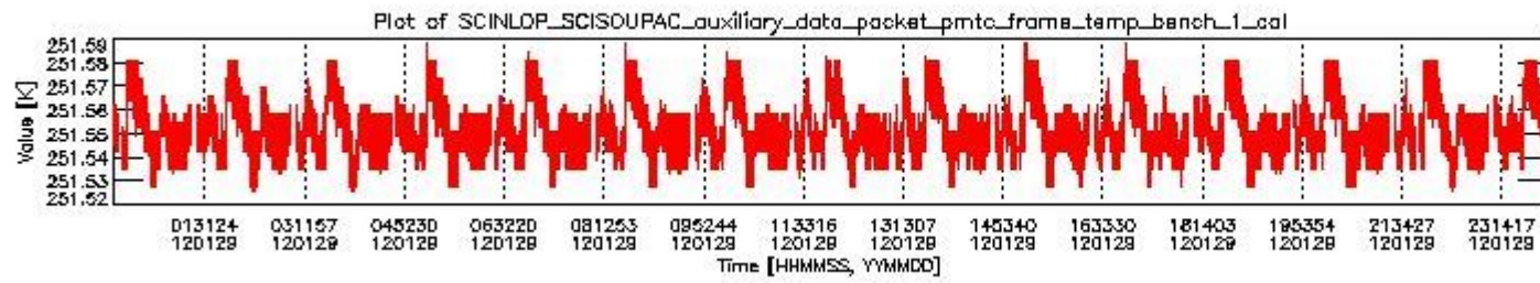
sciamachy_daily_report_level0_KSPT_L0_4504_N_20120129_0.PNG
