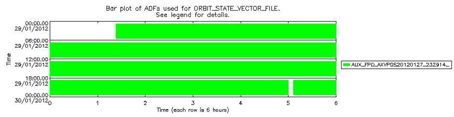
sciamachy_daily_report_level0_KSPT_L0_4504_N_20120129_7.PNG
