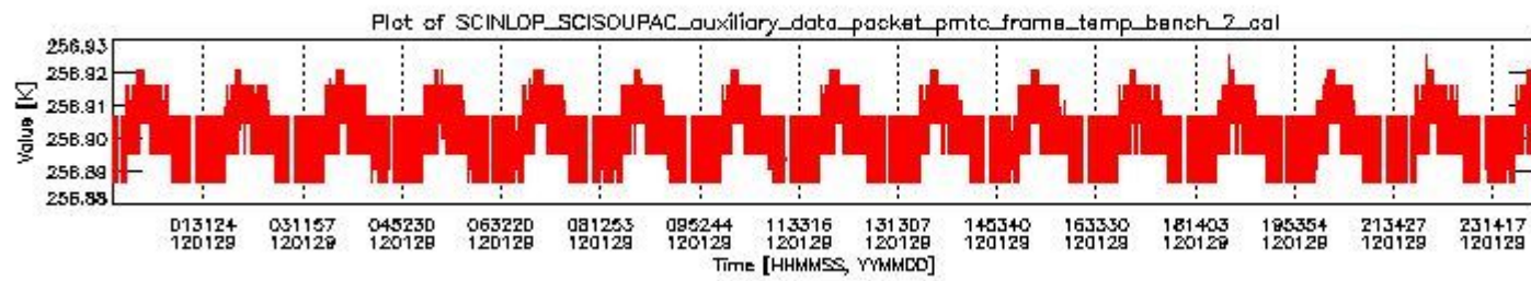
sciamachy_daily_report_level0_KSPT_L0_4504_N_20120129_1.PNG
