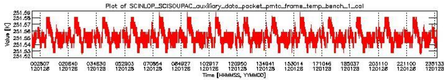
sciamachy_daily_report_level0_KSPT_L0_4504_N_20120128_0.PNG
