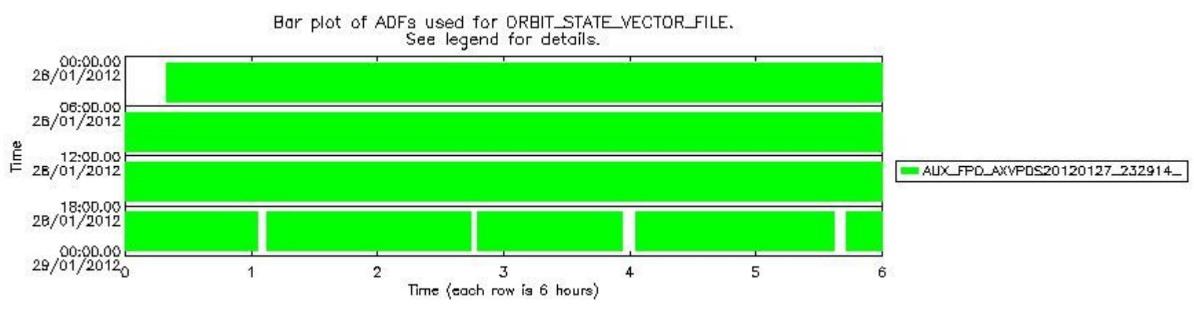
sciamachy_daily_report_level0_KSPT_L0_4504_N_20120128_7.PNG
