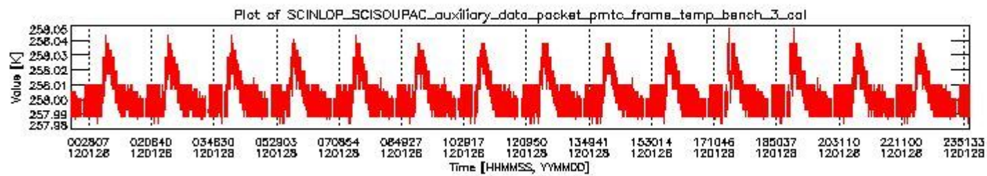
sciamachy_daily_report_level0_KSPT_L0_4504_N_20120128_2.PNG
