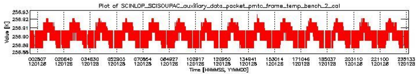
sciamachy_daily_report_level0_KSPT_L0_4504_N_20120128_1.PNG
