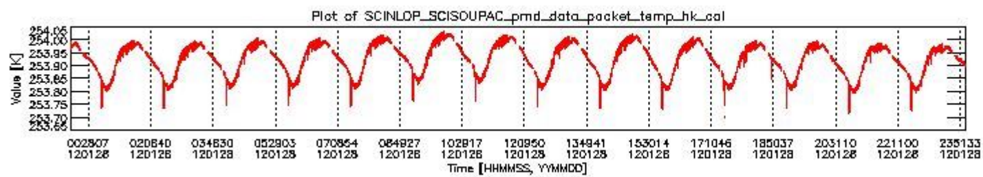
sciamachy_daily_report_level0_KSPT_L0_4504_N_20120128_3.PNG
