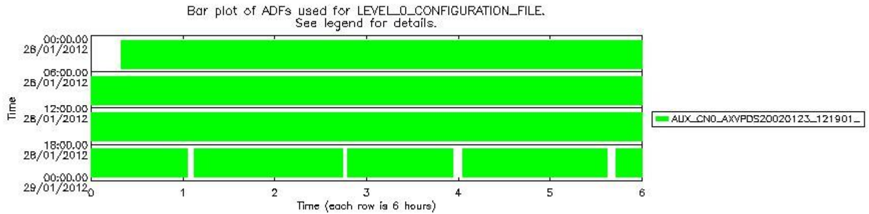
sciamachy_daily_report_level0_KSPT_L0_4504_N_20120128_6.PNG
