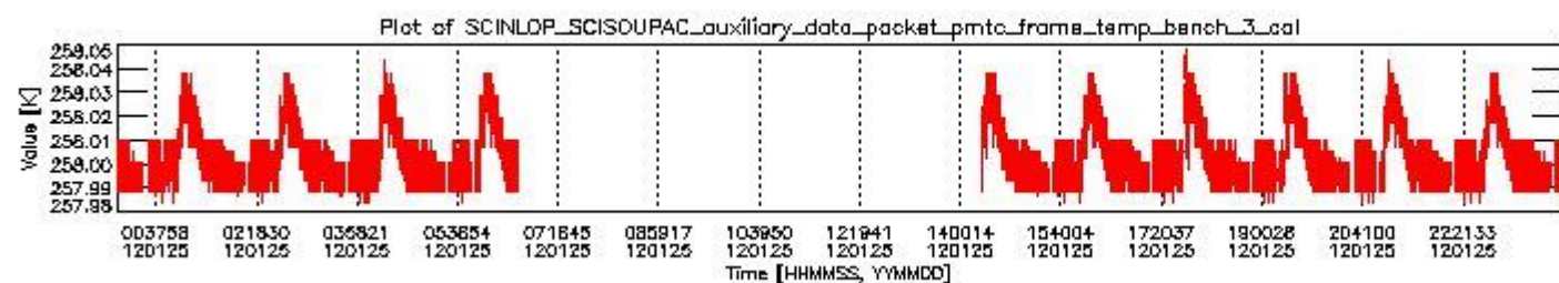
sciamachy_daily_report_level0_KSPT_L0_4504_N_20120125_2.PNG
