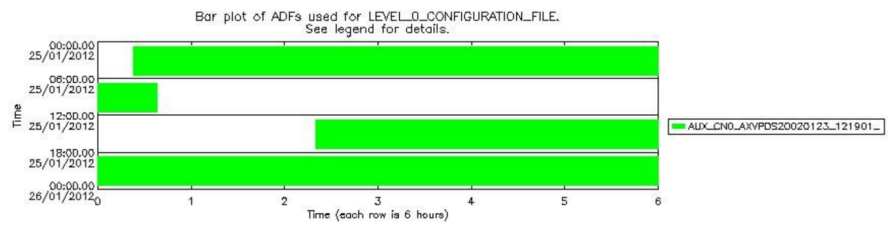
sciamachy_daily_report_level0_KSPT_L0_4504_N_20120125_6.PNG
