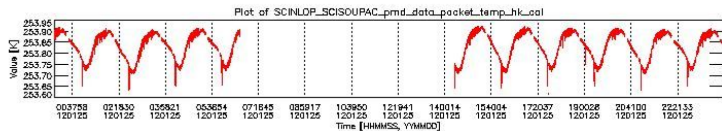
sciamachy_daily_report_level0_KSPT_L0_4504_N_20120125_3.PNG
