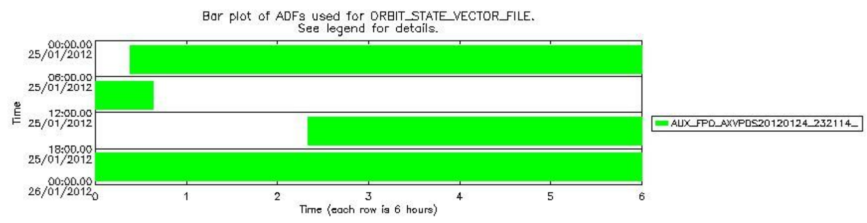
sciamachy_daily_report_level0_KSPT_L0_4504_N_20120125_7.PNG
