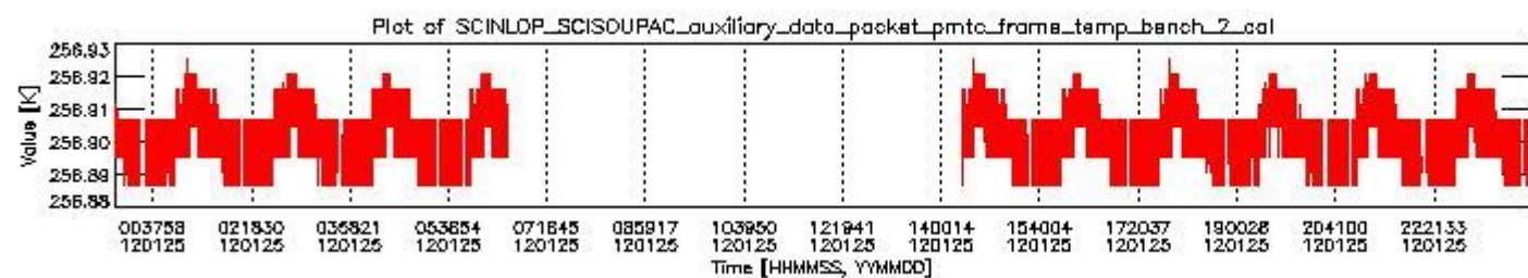
sciamachy_daily_report_level0_KSPT_L0_4504_N_20120125_1.PNG
