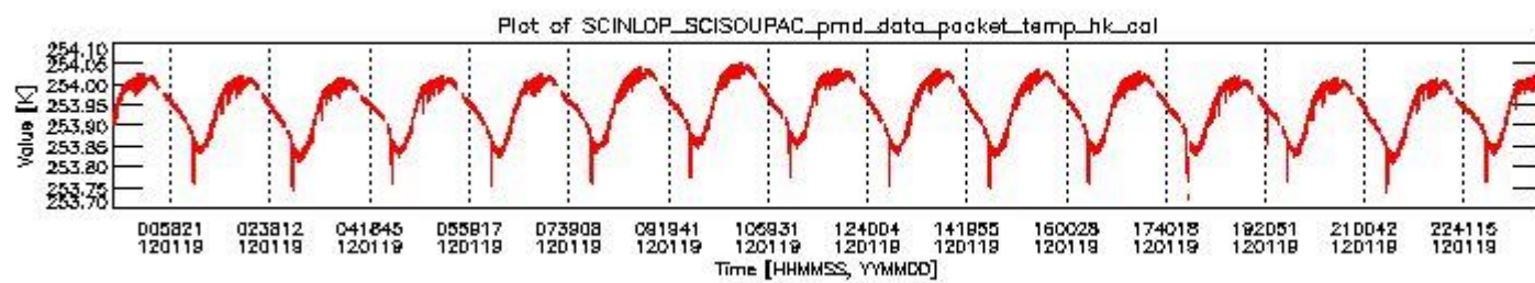
sciamachy_daily_report_level0_KSPT_L0_4504_N_20120119_3.PNG
