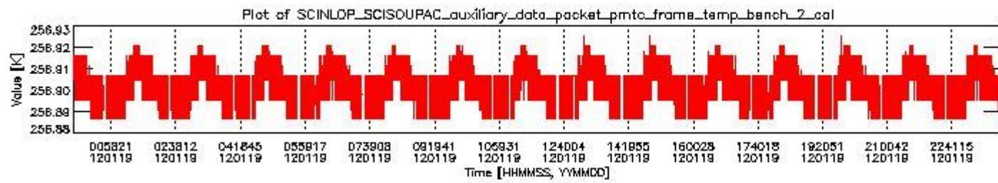
sciamachy_daily_report_level0_KSPT_L0_4504_N_20120119_1.PNG
