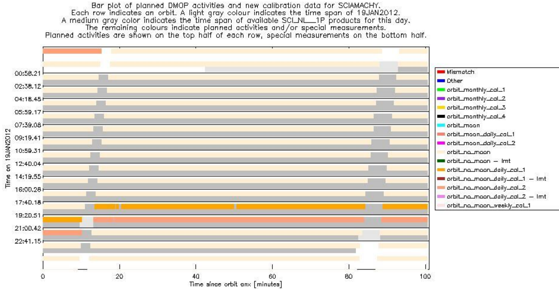
sciamachy_daily_report_level0_KSPT_L0_4504_N_20120119_5.PNG
