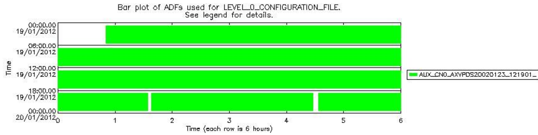
sciamachy_daily_report_level0_KSPT_L0_4504_N_20120119_6.PNG
