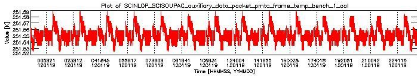
sciamachy_daily_report_level0_KSPT_L0_4504_N_20120119_0.PNG
