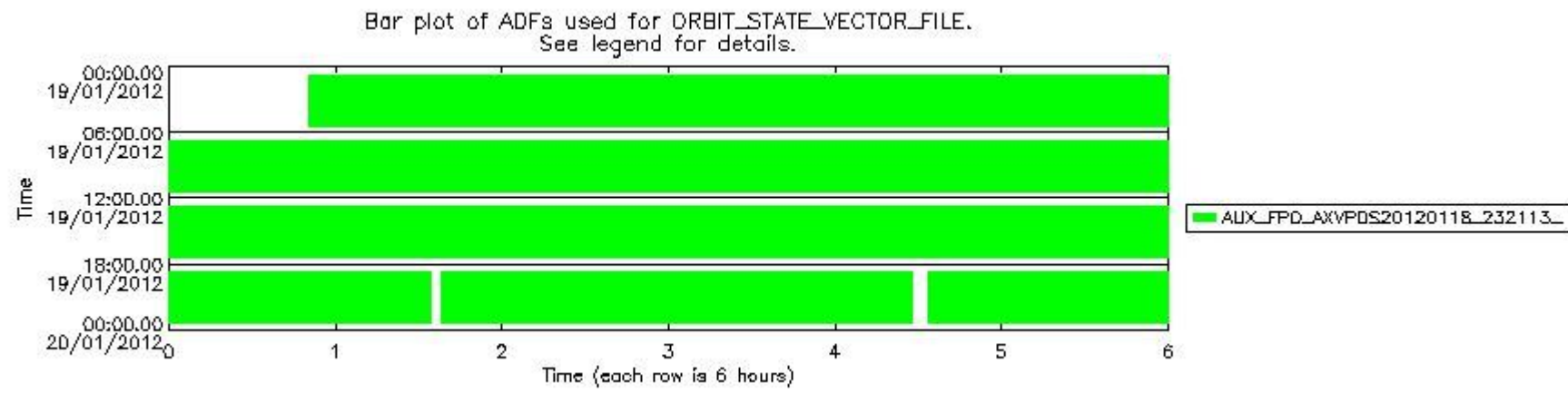
sciamachy_daily_report_level0_KSPT_L0_4504_N_20120119_7.PNG
