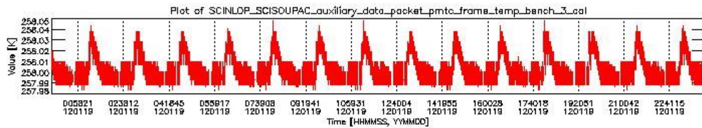
sciamachy_daily_report_level0_KSPT_L0_4504_N_20120119_2.PNG
