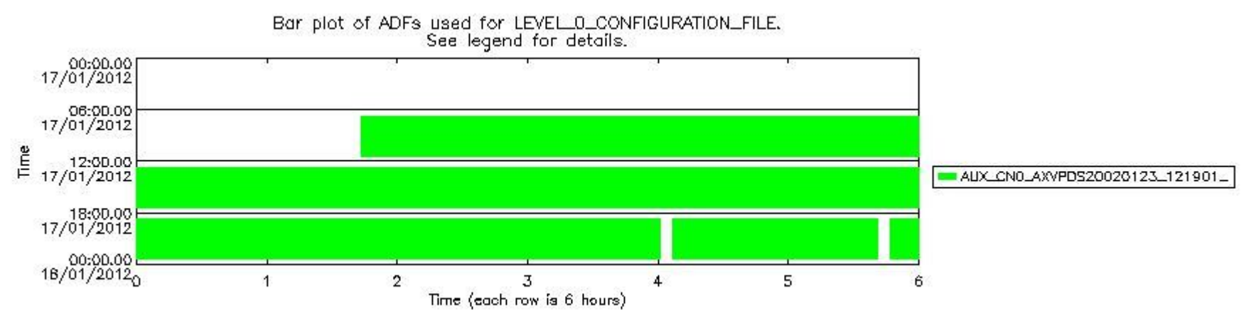
sciamachy_daily_report_level0_KSPT_L0_4504_N_20120117_6.PNG
