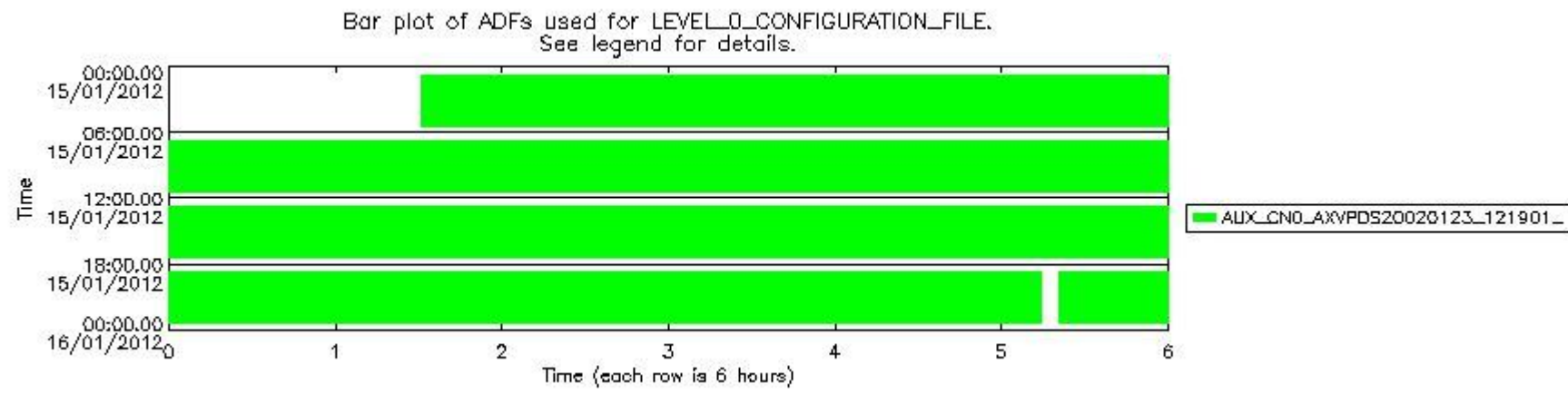
sciamachy_daily_report_level0_KSPT_L0_4504_N_20120115_6.PNG
