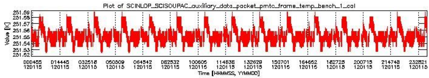
sciamachy_daily_report_level0_KSPT_L0_4504_N_20120115_0.PNG
