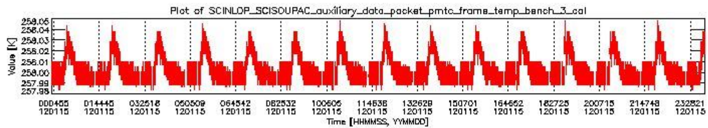
sciamachy_daily_report_level0_KSPT_L0_4504_N_20120115_2.PNG
