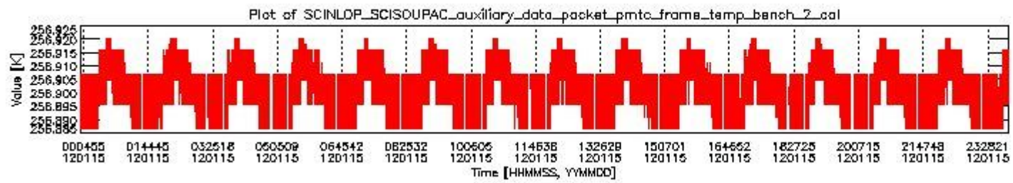
sciamachy_daily_report_level0_KSPT_L0_4504_N_20120115_1.PNG
