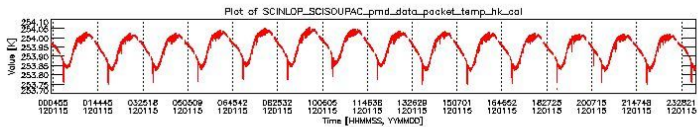
sciamachy_daily_report_level0_KSPT_L0_4504_N_20120115_3.PNG
