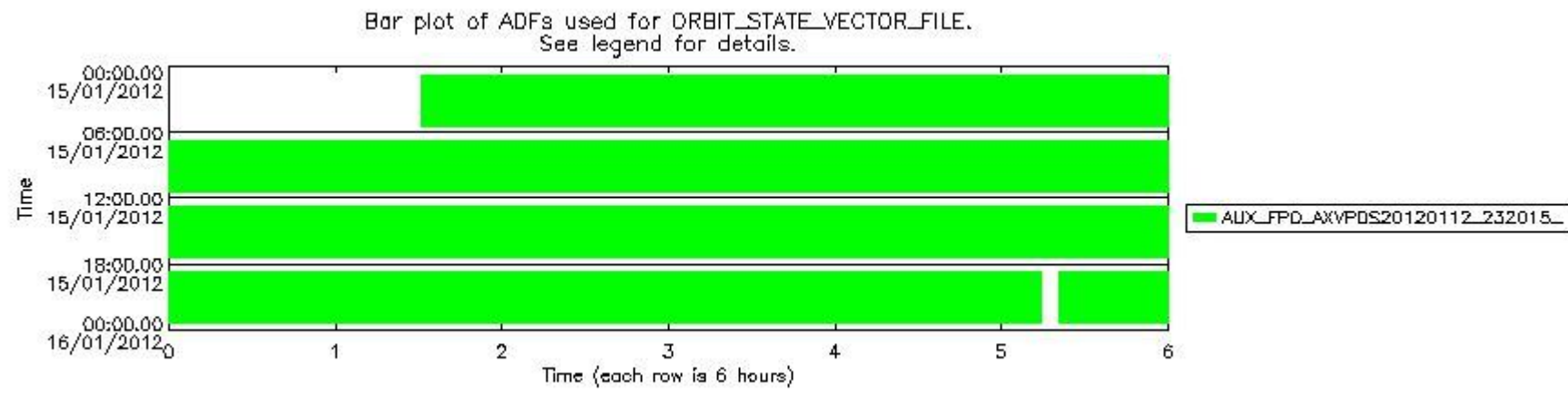
sciamachy_daily_report_level0_KSPT_L0_4504_N_20120115_7.PNG
