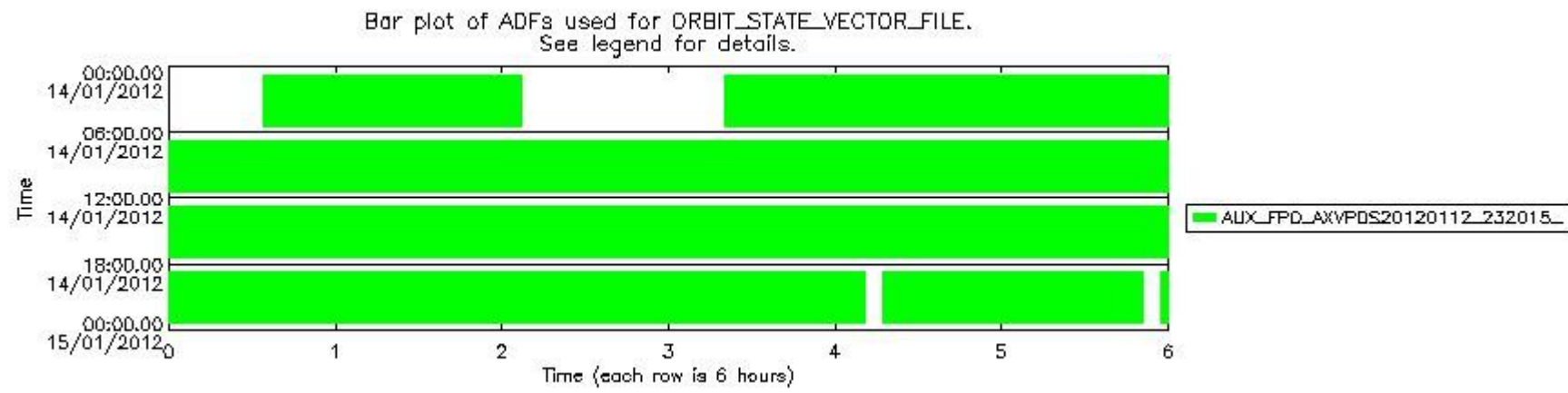
sciamachy_daily_report_level0_KSPT_L0_4504_N_20120114_7.PNG
