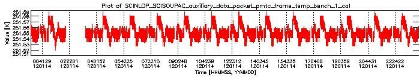
sciamachy_daily_report_level0_KSPT_L0_4504_N_20120114_0.PNG
