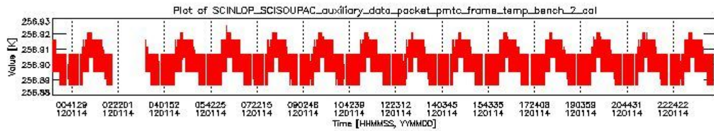
sciamachy_daily_report_level0_KSPT_L0_4504_N_20120114_1.PNG
