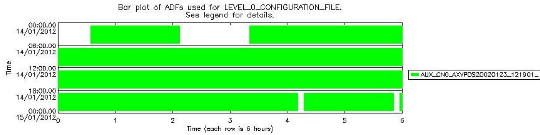
sciamachy_daily_report_level0_KSPT_L0_4504_N_20120114_6.PNG
