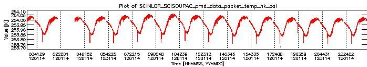
sciamachy_daily_report_level0_KSPT_L0_4504_N_20120114_3.PNG
