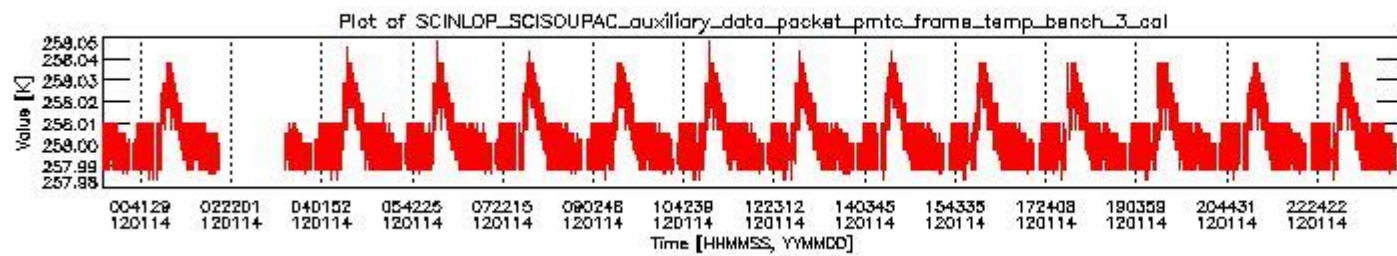
sciamachy_daily_report_level0_KSPT_L0_4504_N_20120114_2.PNG
