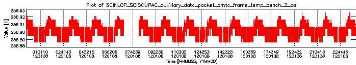
sciamachy_daily_report_level0_KSPT_L0_4504_N_20120108_1.PNG
