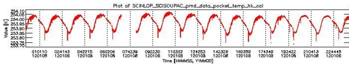
sciamachy_daily_report_level0_KSPT_L0_4504_N_20120108_3.PNG
