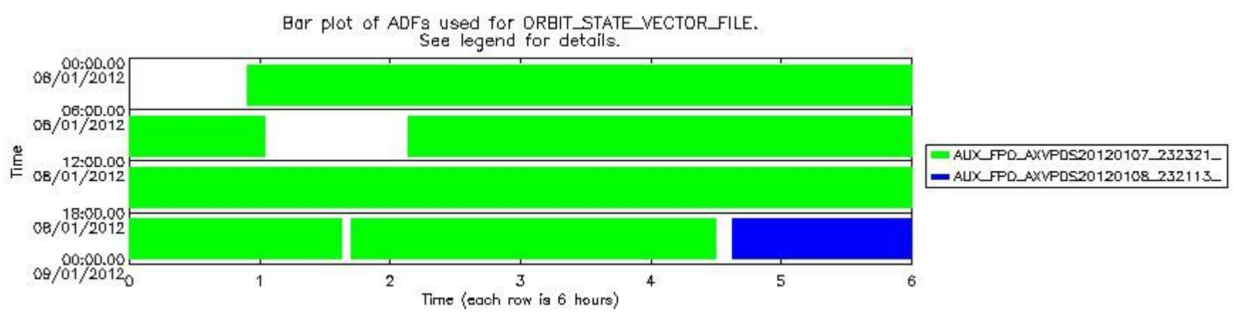
sciamachy_daily_report_level0_KSPT_L0_4504_N_20120108_7.PNG
