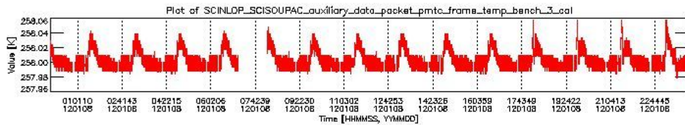
sciamachy_daily_report_level0_KSPT_L0_4504_N_20120108_2.PNG
