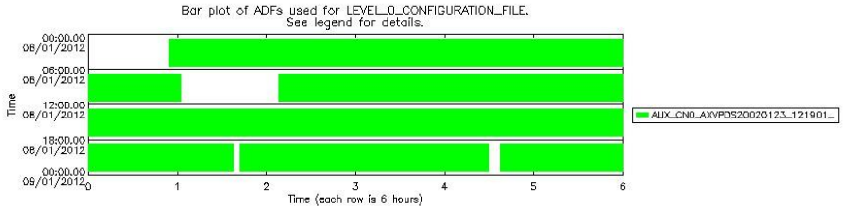
sciamachy_daily_report_level0_KSPT_L0_4504_N_20120108_6.PNG
