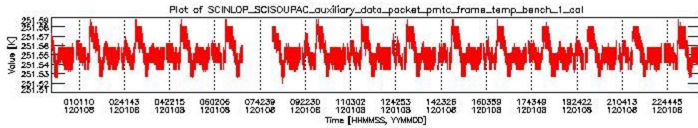
sciamachy_daily_report_level0_KSPT_L0_4504_N_20120108_0.PNG
