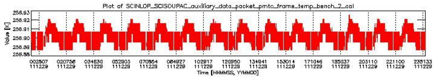
sciamachy_daily_report_level0_KSPT_L0_4504_N_2011229_1.PNG
