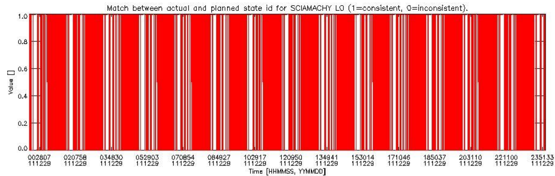
sciamachy_daily_report_level0_KSPT_L0_4504_N_20111229_5.PNG
