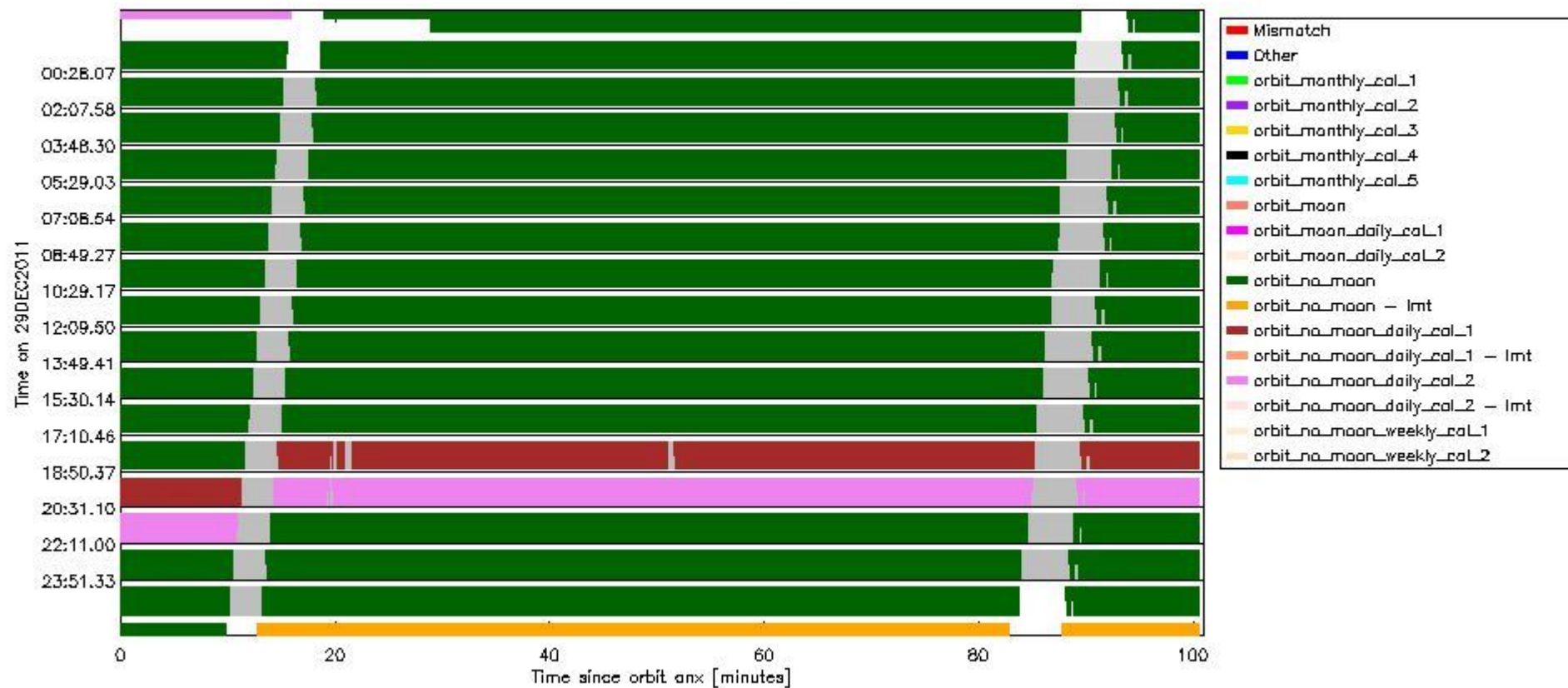
sciamachy_daily_report_level0_KSPT_L0_4504_N_20111229_6.PNG
