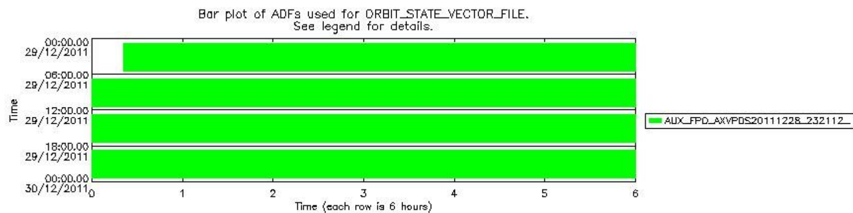
sciamachy_daily_report_level0_KSPT_L0_4504_N_20111229_8.PNG
