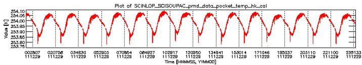
sciamachy_daily_report_level0_KSPT_L0_4504_N_2011229_3.PNG
