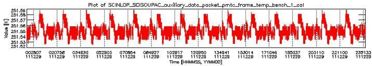
sciamachy_daily_report_level0_KSPT_L0_4504_N_2011229_0.PNG
