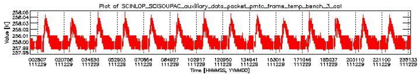
sciamachy_daily_report_level0_KSPT_L0_4504_N_2011229_2.PNG
