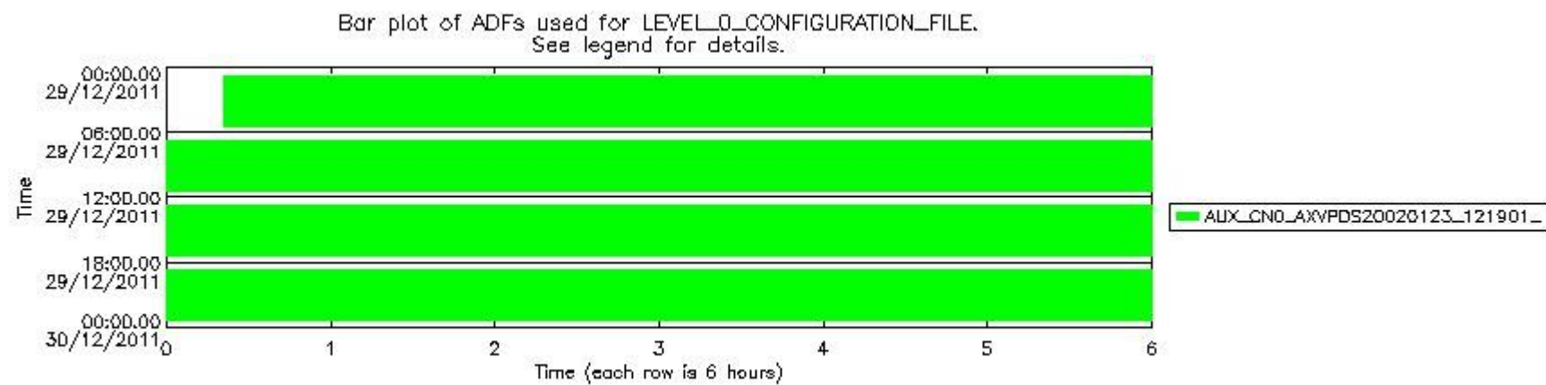
sciamachy_daily_report_level0_KSPT_L0_4504_N_20111229_7.PNG
