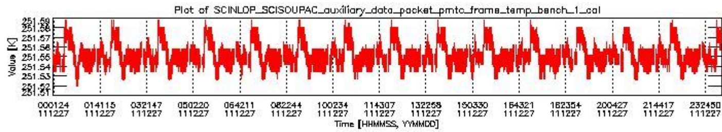
sciamachy_daily_report_level0_KSPT_L0_4504_N_20111227_0.PNG
