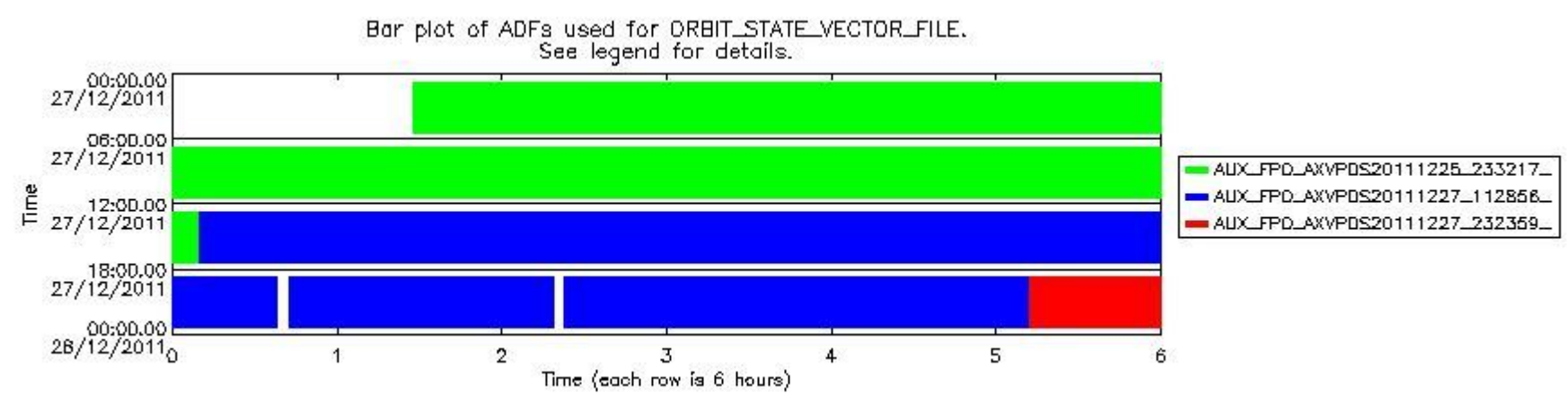
sciamachy_daily_report_level0_KSPT_L0_4504_N_20111227_8.PNG
