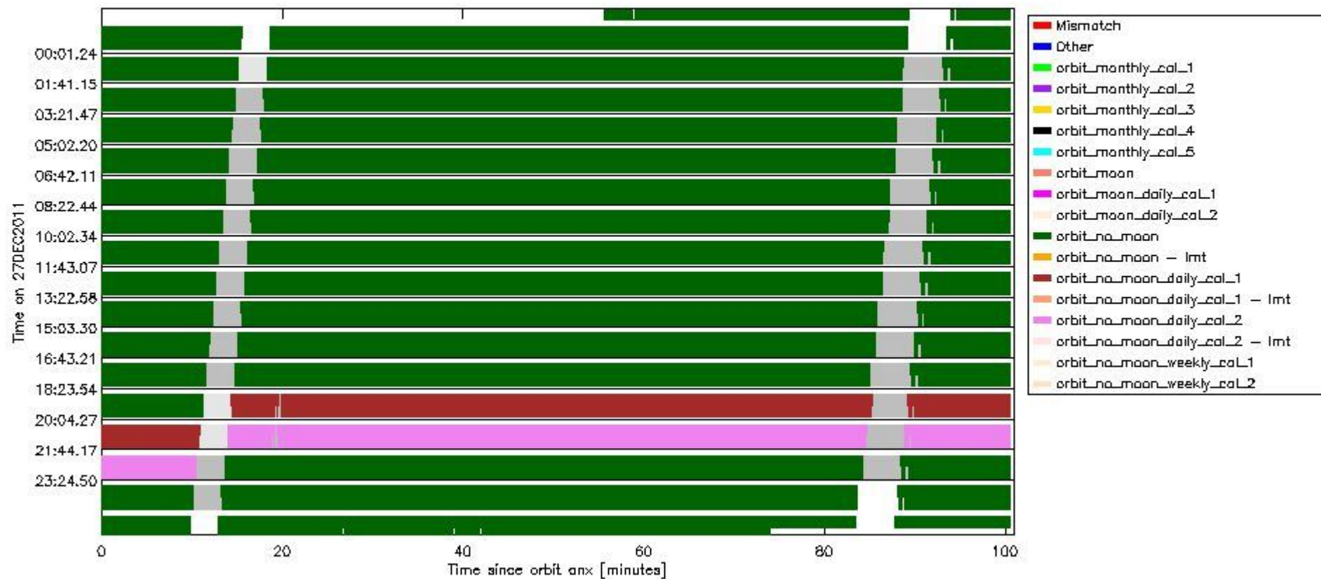
sciamachy_daily_report_level0_KSPT_L0_4504_N_20111227_6.PNG
