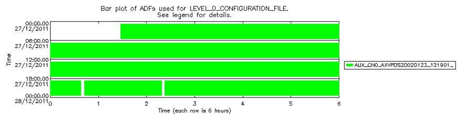
sciamachy_daily_report_level0_KSPT_L0_4504_N_20111227_7.PNG
