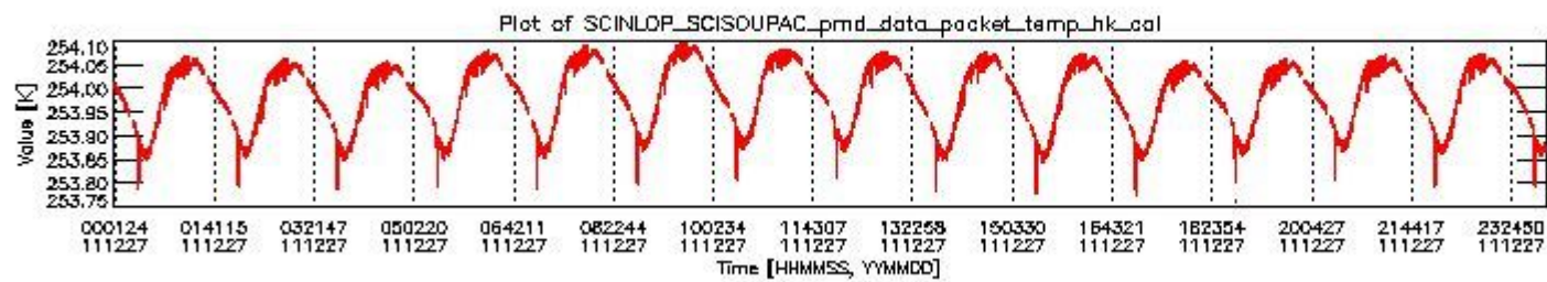
sciamachy_daily_report_level0_KSPT_L0_4504_N_20111227_3.PNG
