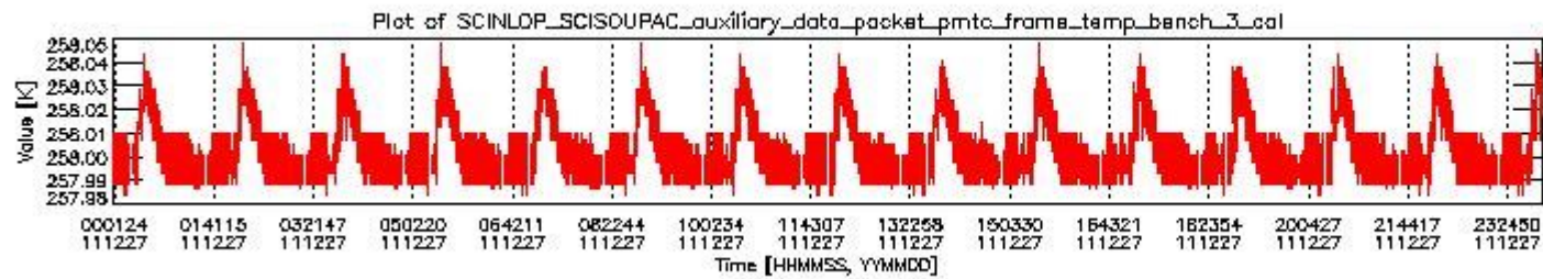
sciamachy_daily_report_level0_KSPT_L0_4504_N_20111227_2.PNG
