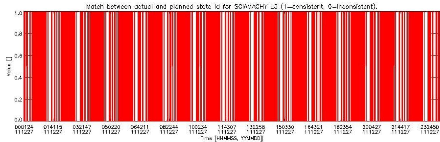
sciamachy_daily_report_level0_KSPT_L0_4504_N_20111227_5.PNG
