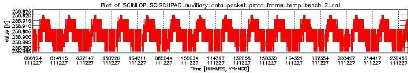
sciamachy_daily_report_level0_KSPT_L0_4504_N_20111227_1.PNG
