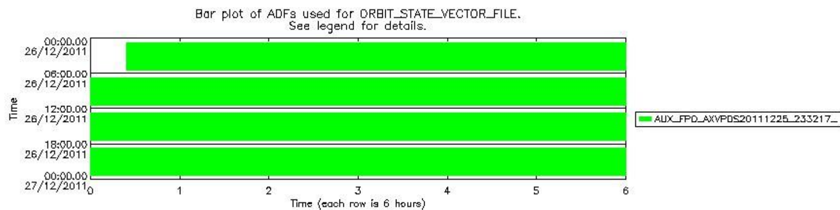
sciamachy_daily_report_level0_KSPT_L0_4504_N_20111226_8.PNG
