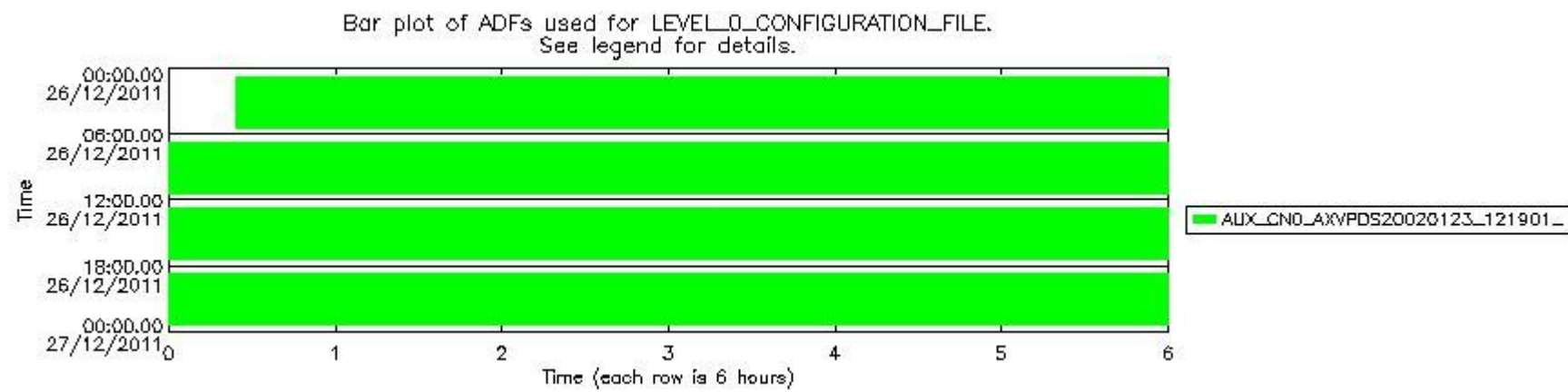
sciamachy_daily_report_level0_KSPT_L0_4504_N_20111226_7.PNG
