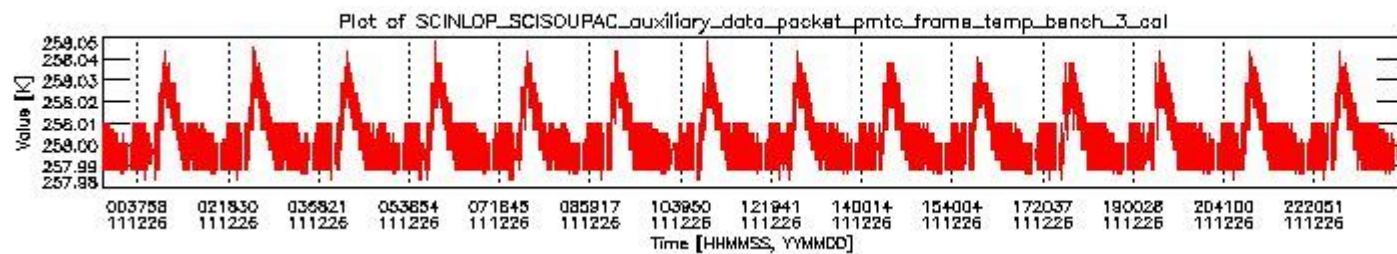
sciamachy_daily_report_level0_KSPT_L0_4504_N_20111226_2.PNG
