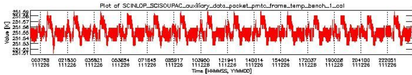
sciamachy_daily_report_level0_KSPT_L0_4504_N_20111226_0.PNG
