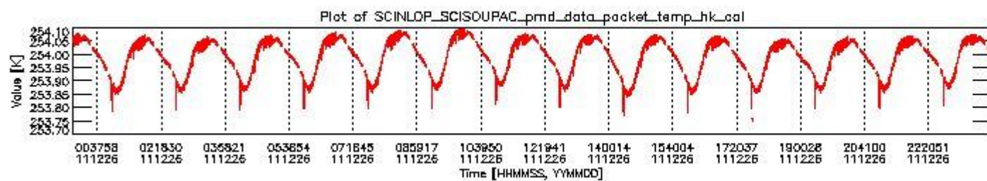
sciamachy_daily_report_level0_KSPT_L0_4504_N_20111226_3.PNG
