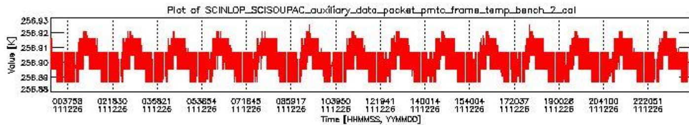
sciamachy_daily_report_level0_KSPT_L0_4504_N_20111226_1.PNG
