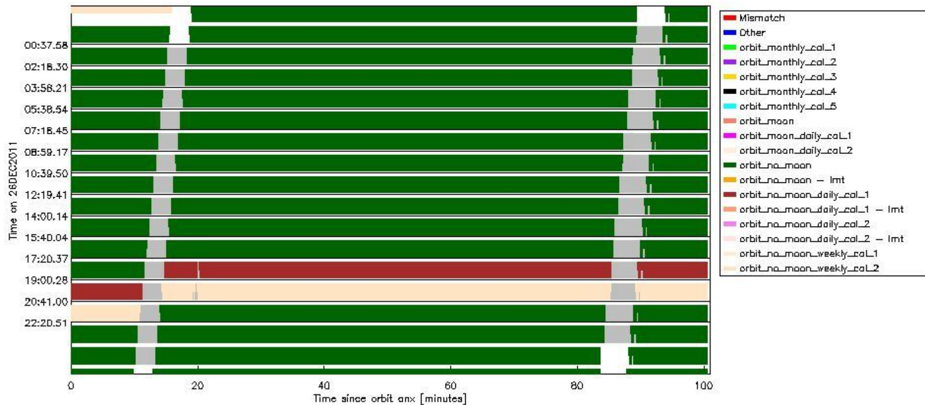
sciamachy_daily_report_level0_KSPT_L0_4504_N_20111226_6.PNG
