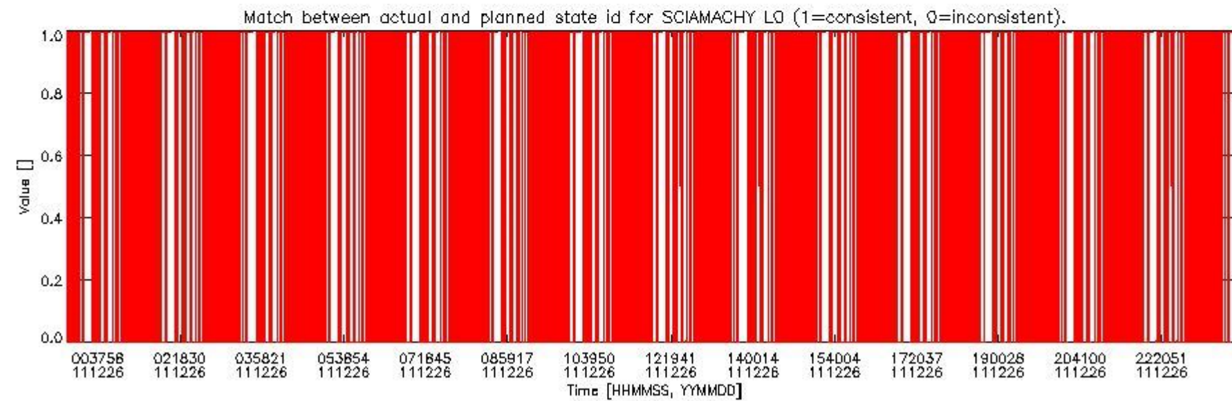
sciamachy_daily_report_level0_KSPT_L0_4504_N_20111226_5.PNG
