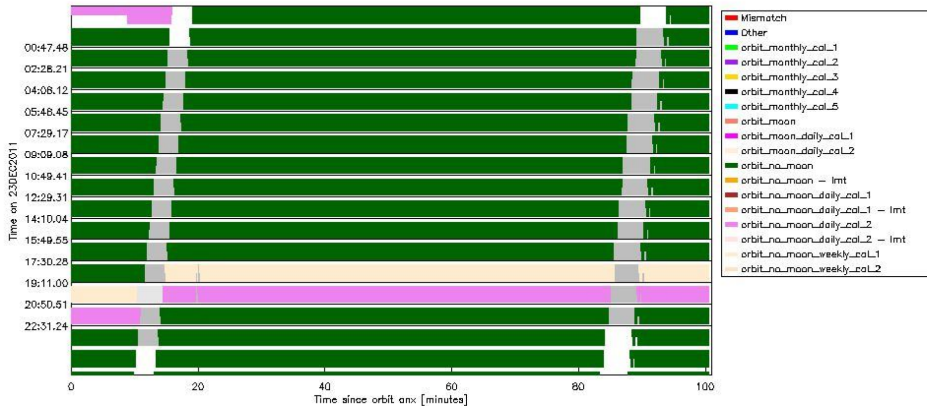
sciamachy_daily_report_level0_KSPT_L0_4504_N_20111223_6.PNG
