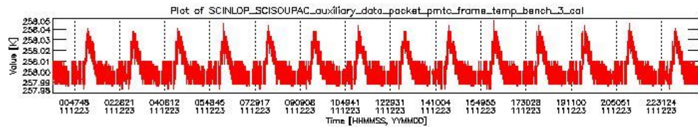
sciamachy_daily_report_level0_KSPT_L0_4504_N_20111223_2.PNG
