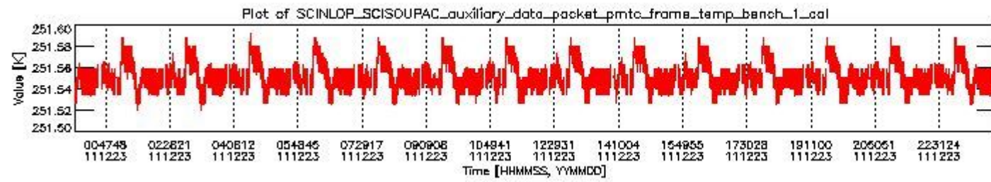
sciamachy_daily_report_level0_KSPT_L0_4504_N_20111223_0.PNG
