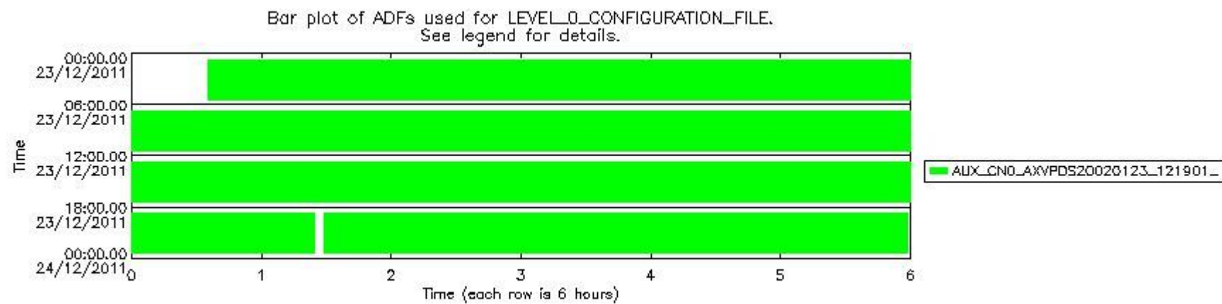
sciamachy_daily_report_level0_KSPT_L0_4504_N_20111223_7.PNG
