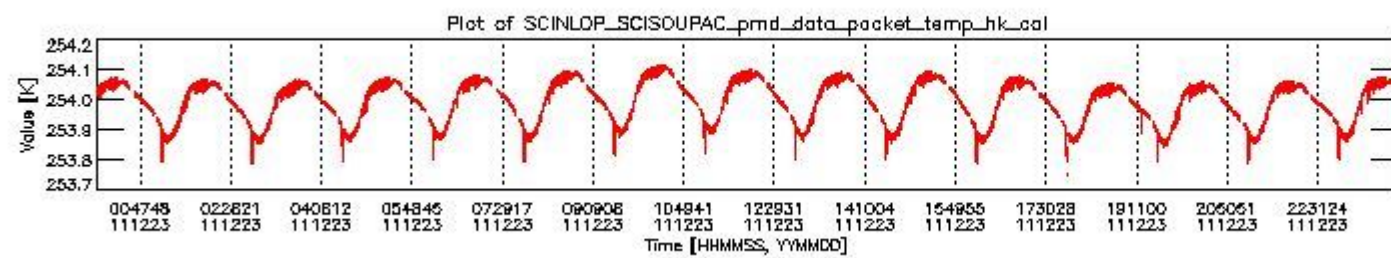
sciamachy_daily_report_level0_KSPT_L0_4504_N_20111223_3.PNG
