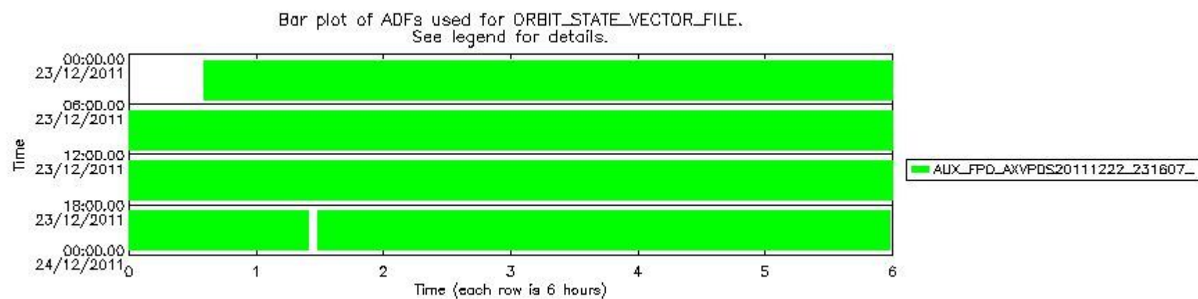
sciamachy_daily_report_level0_KSPT_L0_4504_N_20111223_8.PNG
