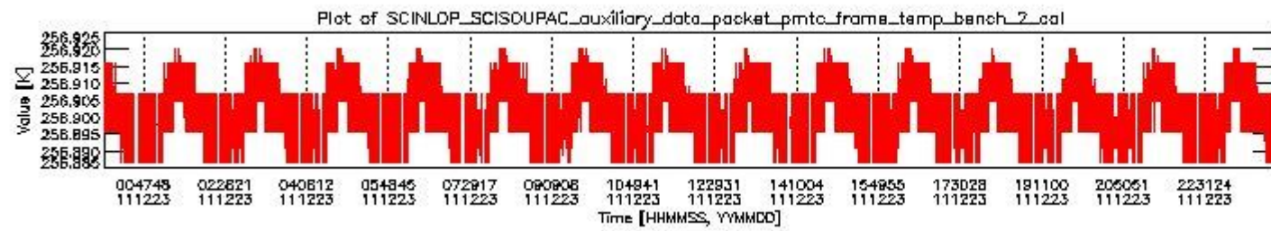
sciamachy_daily_report_level0_KSPT_L0_4504_N_20111223_1.PNG
