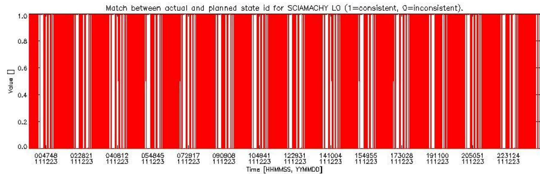
sciamachy_daily_report_level0_KSPT_L0_4504_N_20111223_5.PNG
