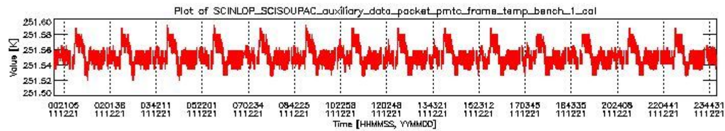
sciamachy_daily_report_level0_KSPT_L0_4504_N_2011221_0.PNG
