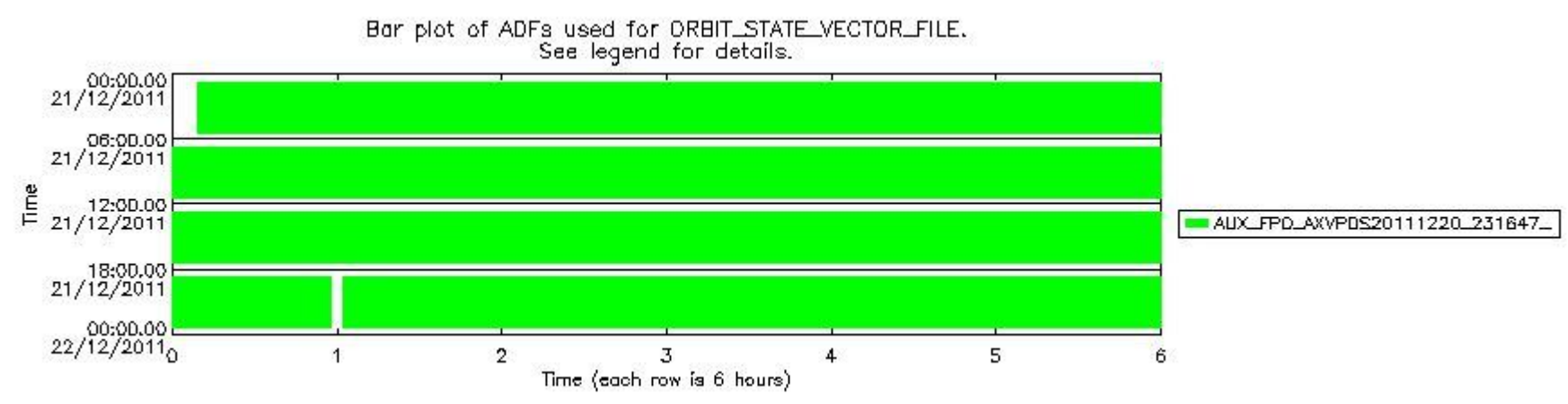
sciamachy_daily_report_level0_KSPT_L0_4504_N_20111221_8.PNG
