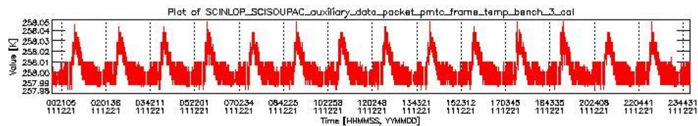
sciamachy_daily_report_level0_KSPT_L0_4504_N_2011221_2.PNG
