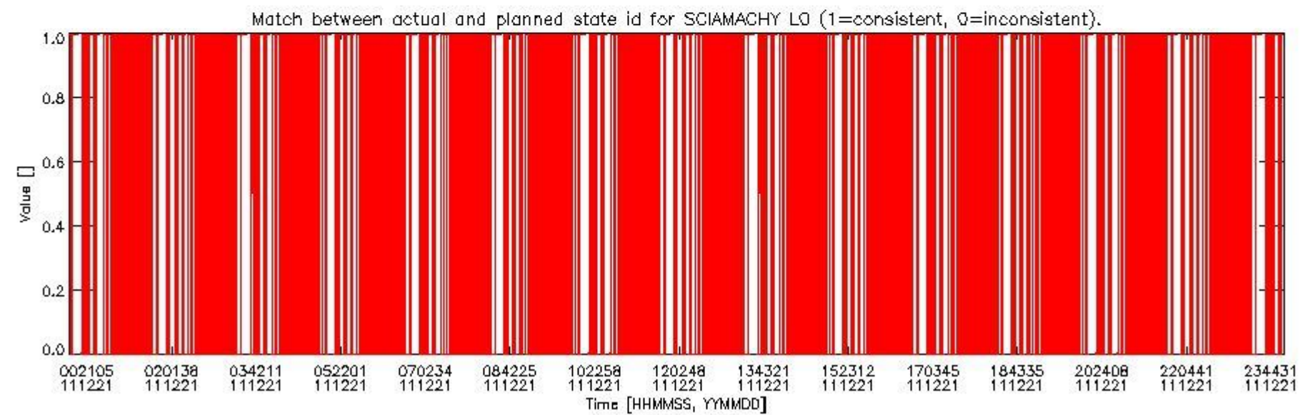
sciamachy_daily_report_level0_KSPT_L0_4504_N_20111221_5.PNG
