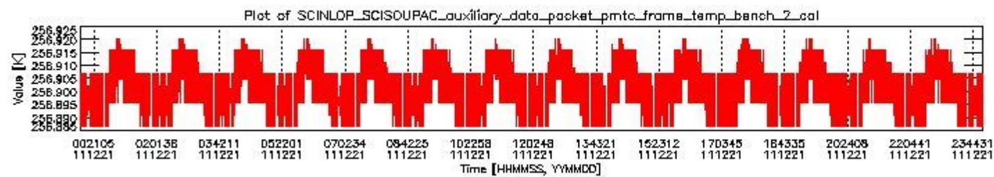
sciamachy_daily_report_level0_KSPT_L0_4504_N_2011221_1.PNG
