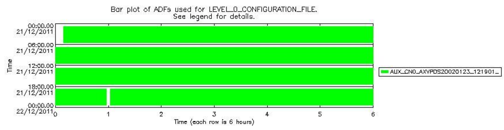
sciamachy_daily_report_level0_KSPT_L0_4504_N_20111221_7.PNG
