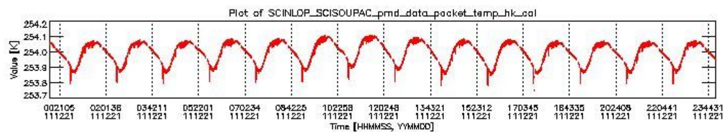
sciamachy_daily_report_level0_KSPT_L0_4504_N_2011221_3.PNG
