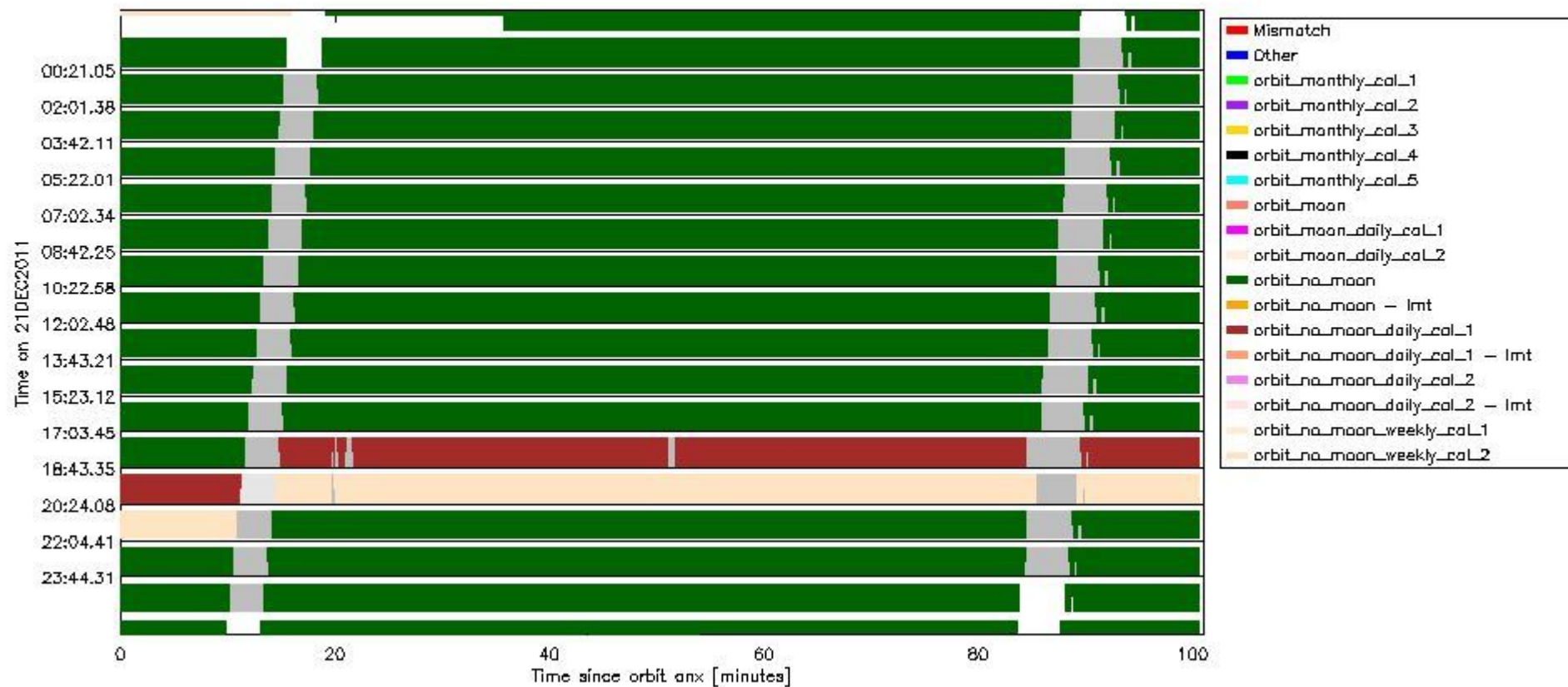
sciamachy_daily_report_level0_KSPT_L0_4504_N_20111221_6.PNG
