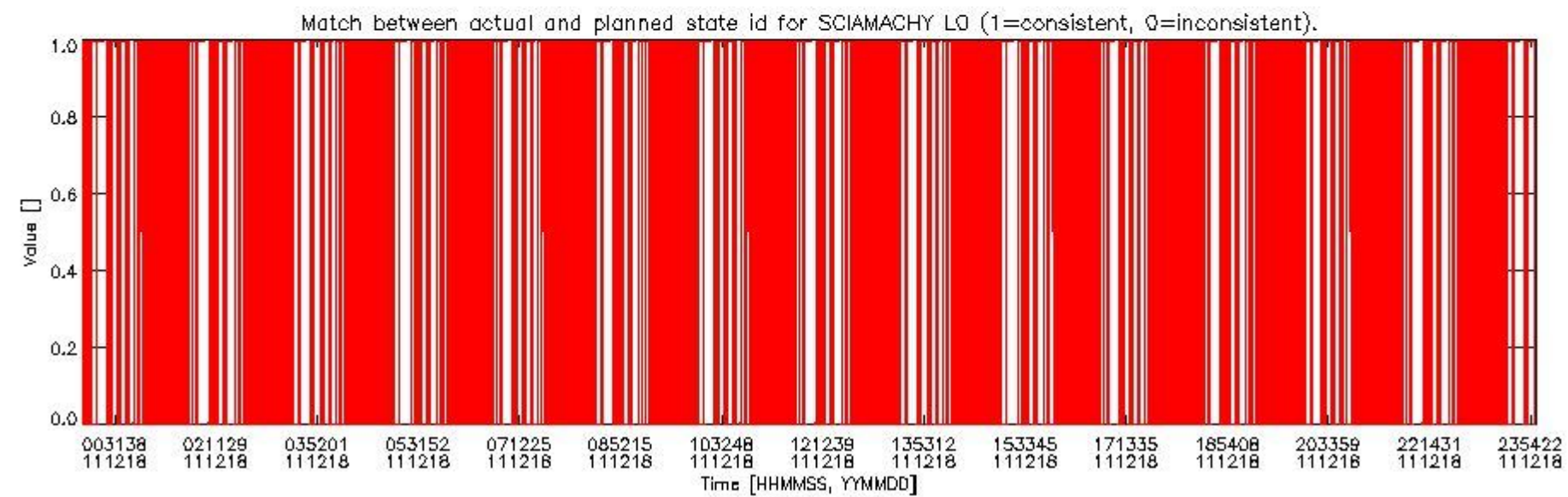
sciamachy_daily_report_level0_KSPT_L0_4504_N_20111218_5.PNG
