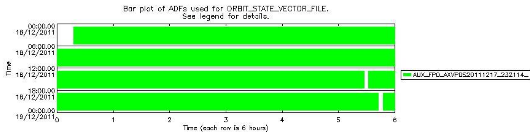
sciamachy_daily_report_level0_KSPT_L0_4504_N_20111218_8.PNG
