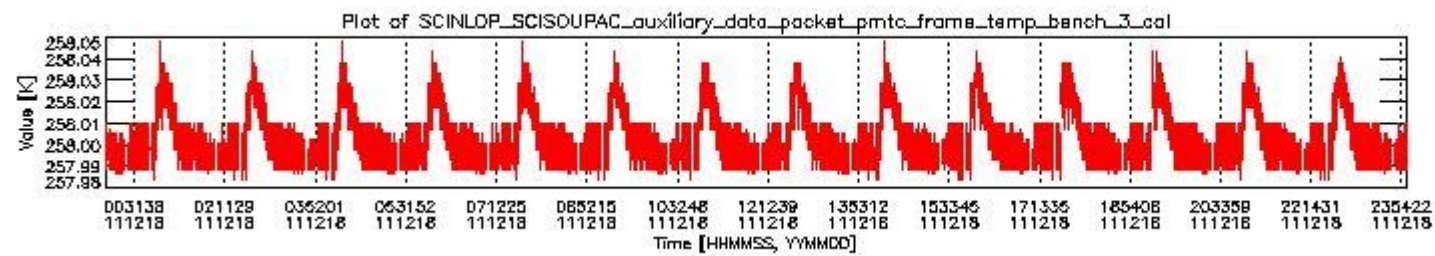
sciamachy_daily_report_level0_KSPT_L0_4504_N_20111218_2.PNG
