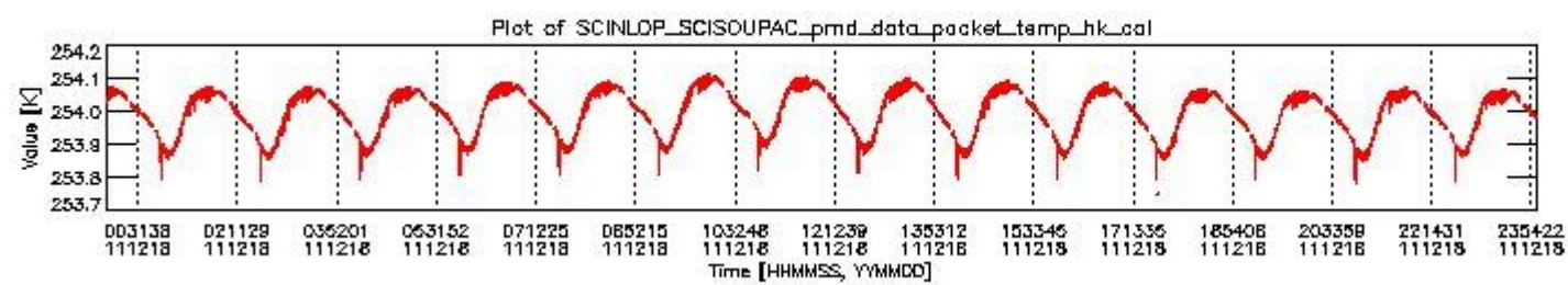
sciamachy_daily_report_level0_KSPT_L0_4504_N_20111218_3.PNG
