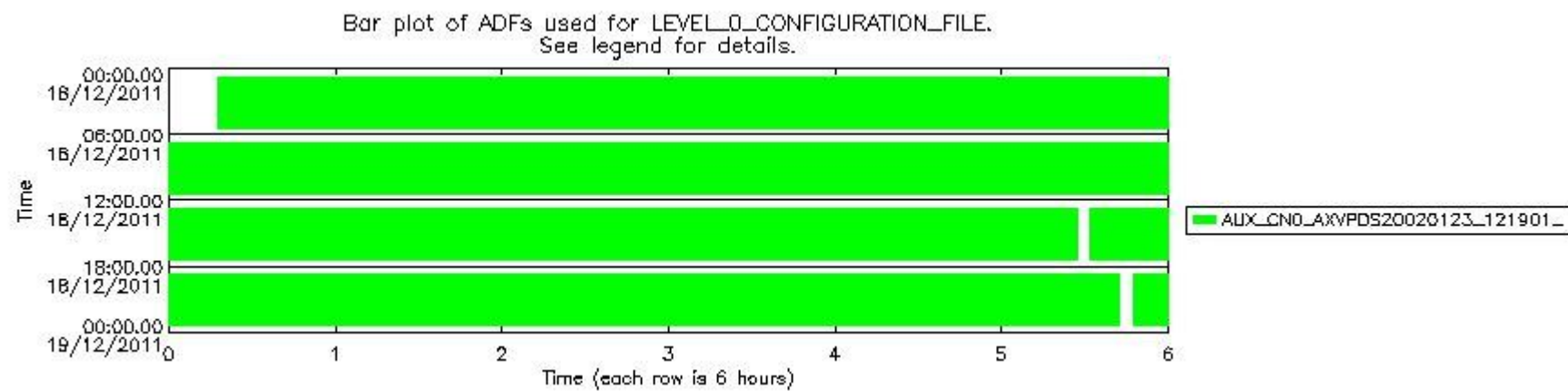
sciamachy_daily_report_level0_KSPT_L0_4504_N_20111218_7.PNG
