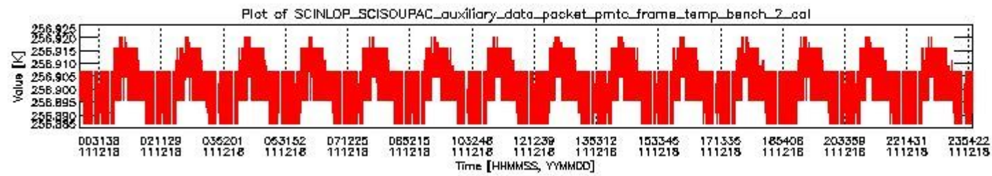
sciamachy_daily_report_level0_KSPT_L0_4504_N_20111218_1.PNG
