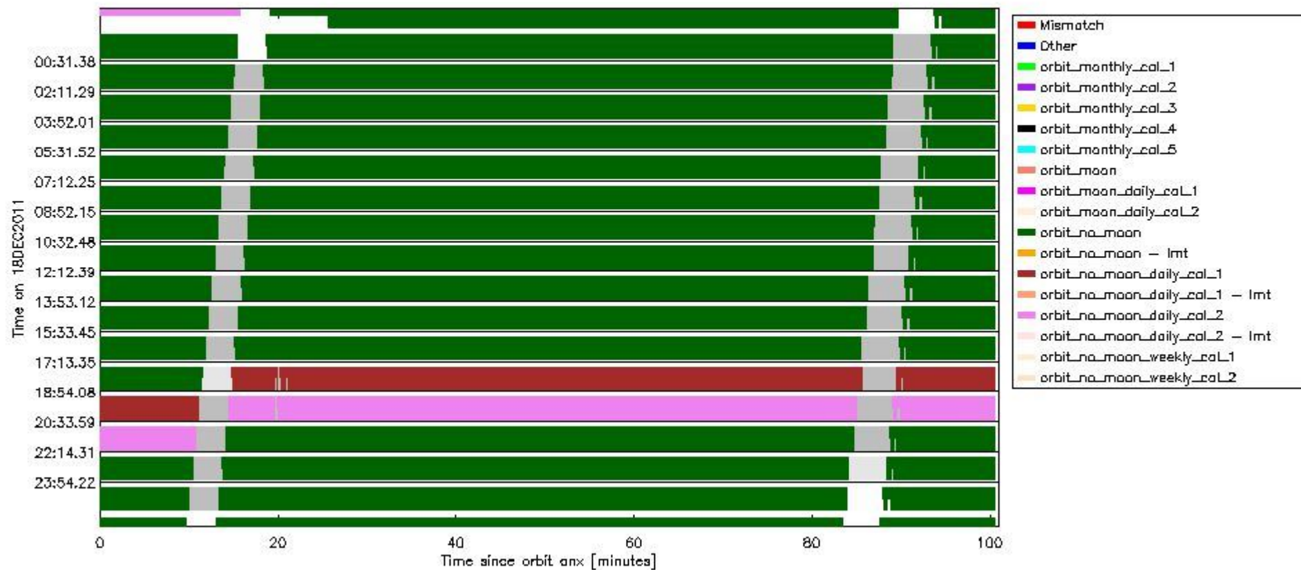
sciamachy_daily_report_level0_KSPT_L0_4504_N_20111218_6.PNG
