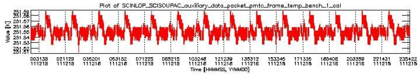
sciamachy_daily_report_level0_KSPT_L0_4504_N_20111218_0.PNG
