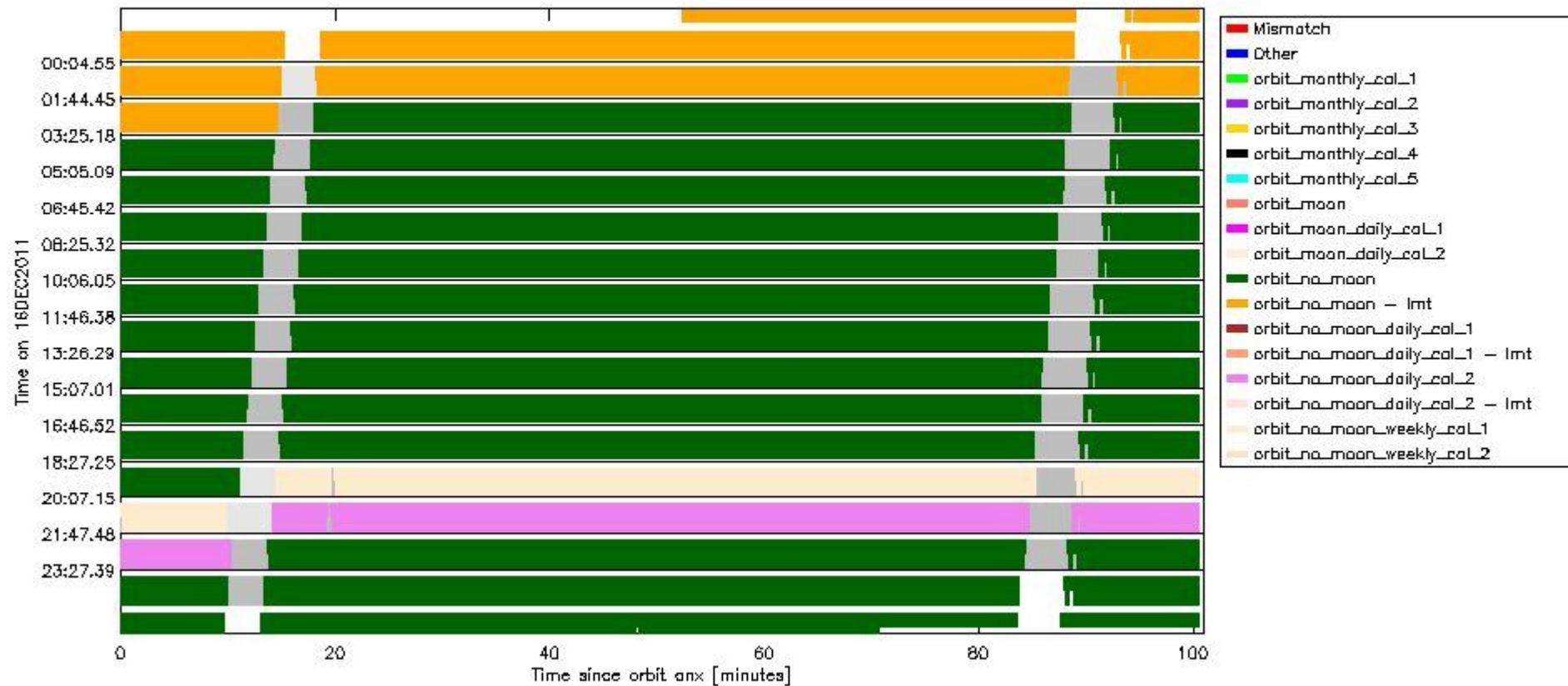
sciamachy_daily_report_level0_KSPT_L0_4504_N_20111216_6.PNG
