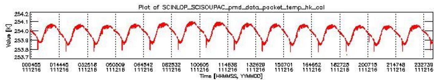
sciamachy_daily_report_level0_KSPT_L0_4504_N_20111216_3.PNG
