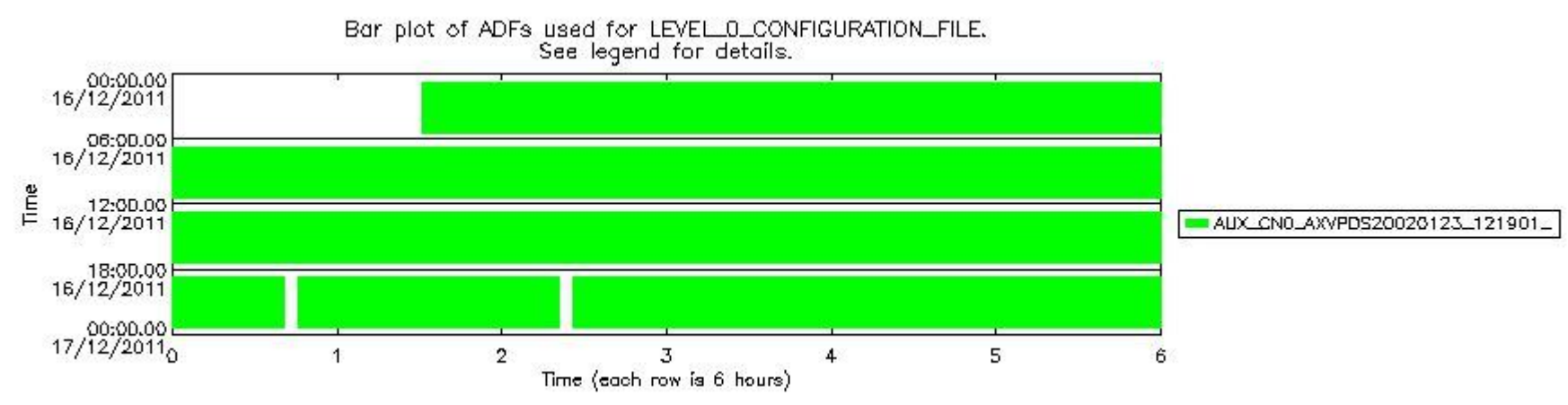
sciamachy_daily_report_level0_KSPT_L0_4504_N_20111216_7.PNG
