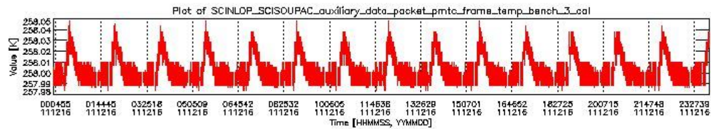
sciamachy_daily_report_level0_KSPT_L0_4504_N_20111216_2.PNG
