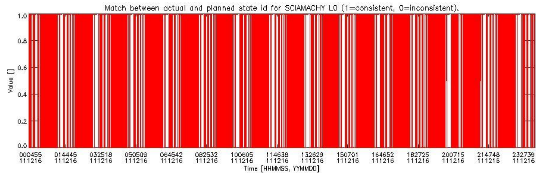
sciamachy_daily_report_level0_KSPT_L0_4504_N_20111216_5.PNG
