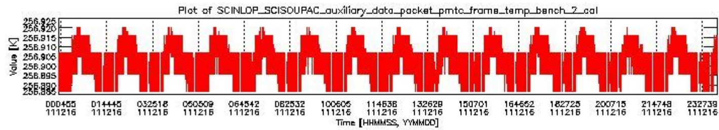
sciamachy_daily_report_level0_KSPT_L0_4504_N_20111216_1.PNG
