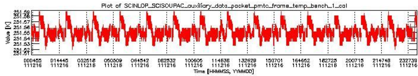
sciamachy_daily_report_level0_KSPT_L0_4504_N_20111216_0.PNG
