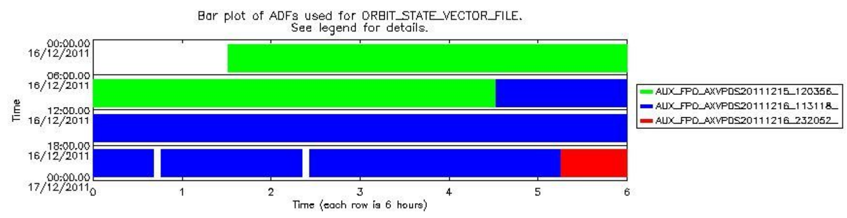
sciamachy_daily_report_level0_KSPT_L0_4504_N_20111216_8.PNG
