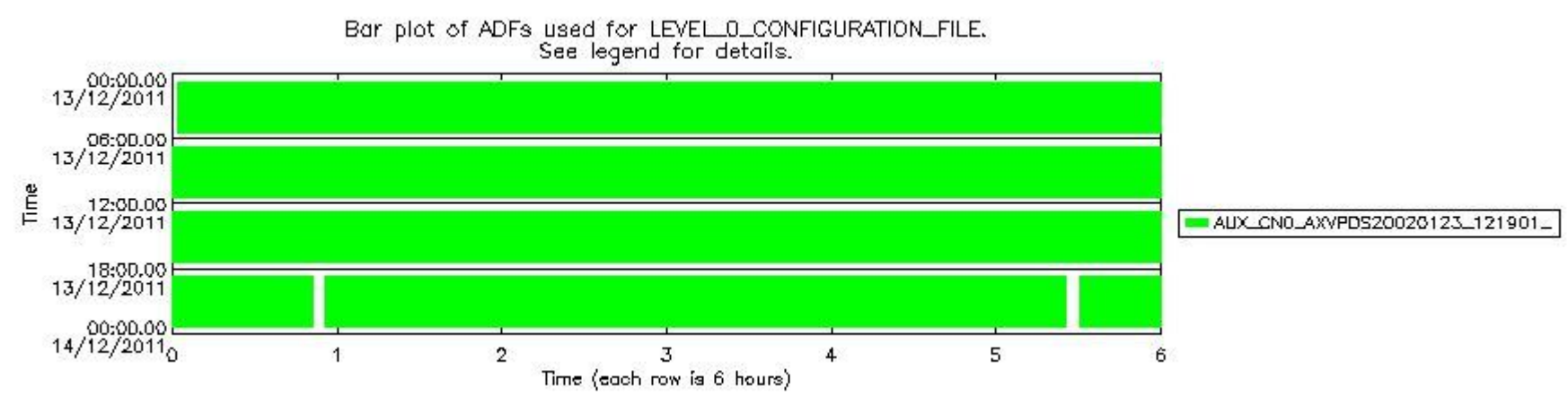
sciamachy_daily_report_level0_KSPT_L0_4504_N_20111213_7.PNG
