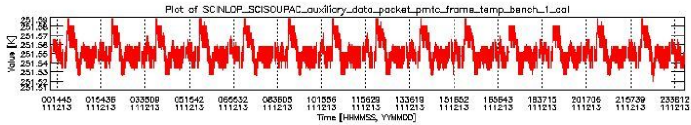
sciamachy_daily_report_level0_KSPT_L0_4504_N_20111213_0.PNG
