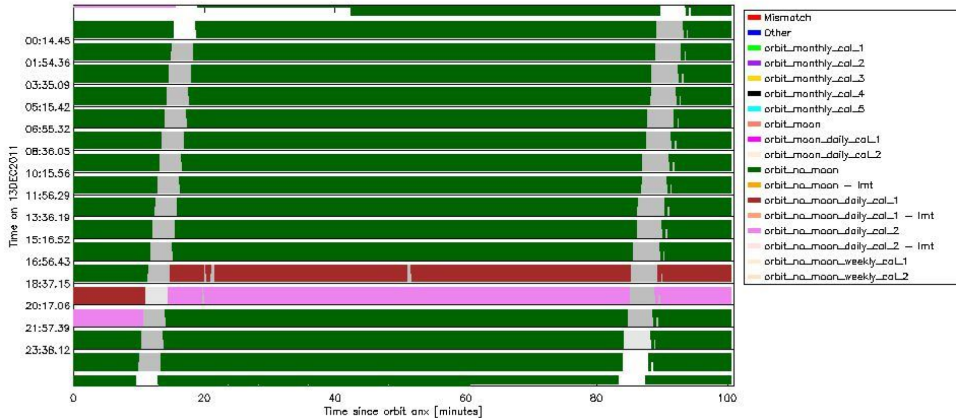
sciamachy_daily_report_level0_KSPT_L0_4504_N_20111213_6.PNG
