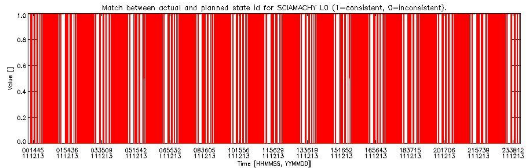
sciamachy_daily_report_level0_KSPT_L0_4504_N_20111213_5.PNG
