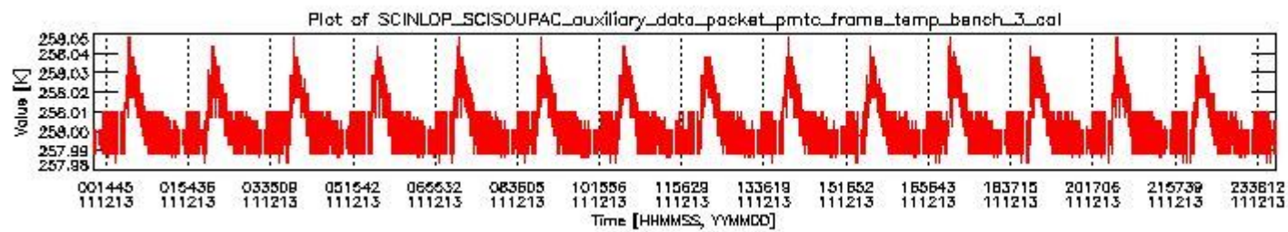
sciamachy_daily_report_level0_KSPT_L0_4504_N_20111213_2.PNG
