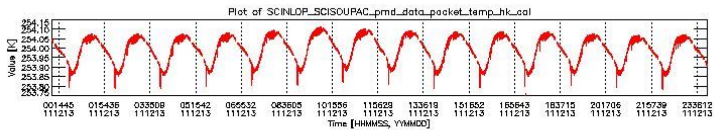
sciamachy_daily_report_level0_KSPT_L0_4504_N_20111213_3.PNG
