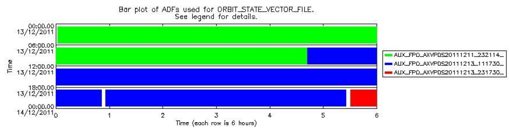
sciamachy_daily_report_level0_KSPT_L0_4504_N_20111213_8.PNG
