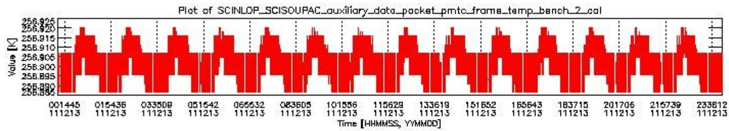
sciamachy_daily_report_level0_KSPT_L0_4504_N_20111213_1.PNG
