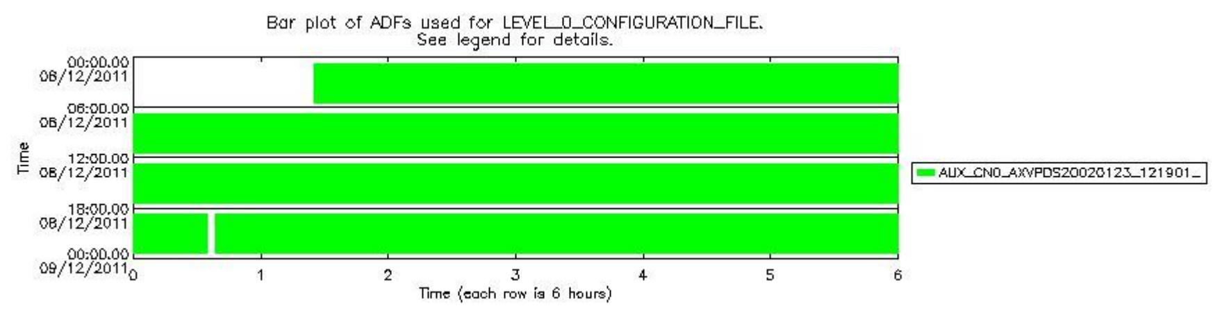
sciamachy_daily_report_level0_KSPT_L0_4504_N_20111208_7.PNG
