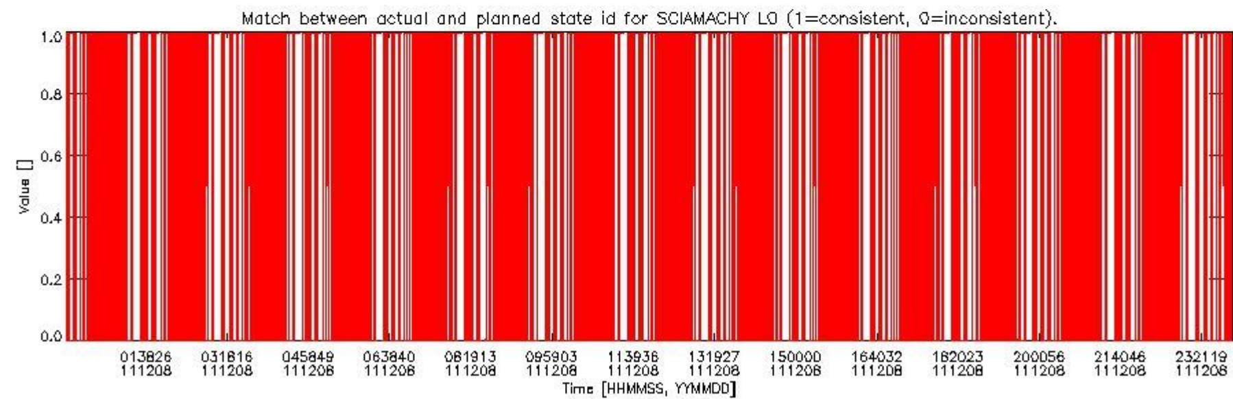
sciamachy_daily_report_level0_KSPT_L0_4504_N_2011208_5.PNG
