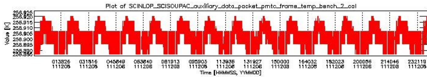
sciamachy_daily_report_level0_KSPT_L0_4504_N_20111208_1.PNG
