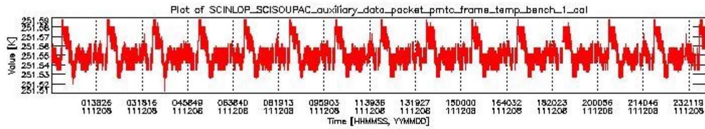
sciamachy_daily_report_level0_KSPT_L0_4504_N_20111208_0.PNG
