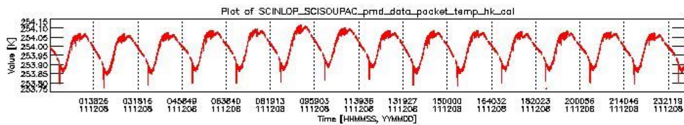
sciamachy_daily_report_level0_KSPT_L0_4504_N_20111208_3.PNG
