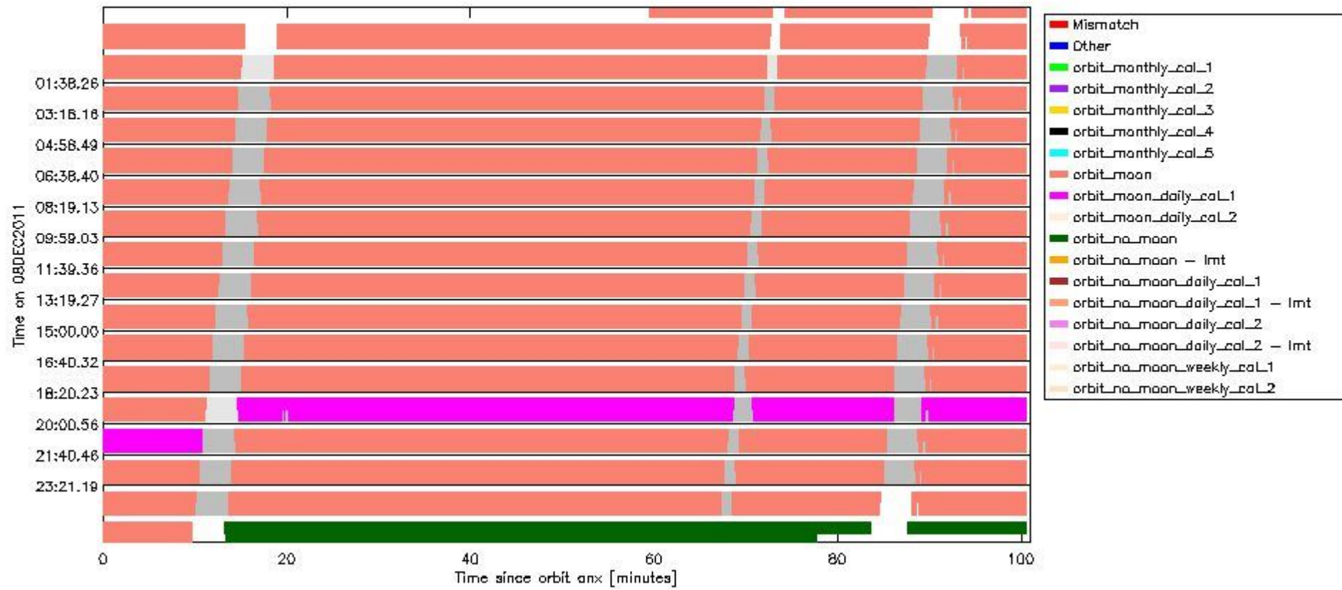
sciamachy_daily_report_level0_KSPT_L0_4504_N_20111208_6.PNG
