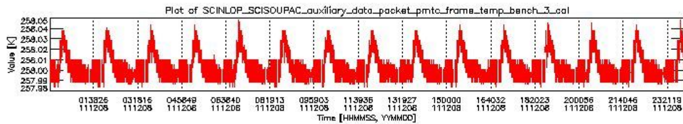
sciamachy_daily_report_level0_KSPT_L0_4504_N_20111208_2.PNG
