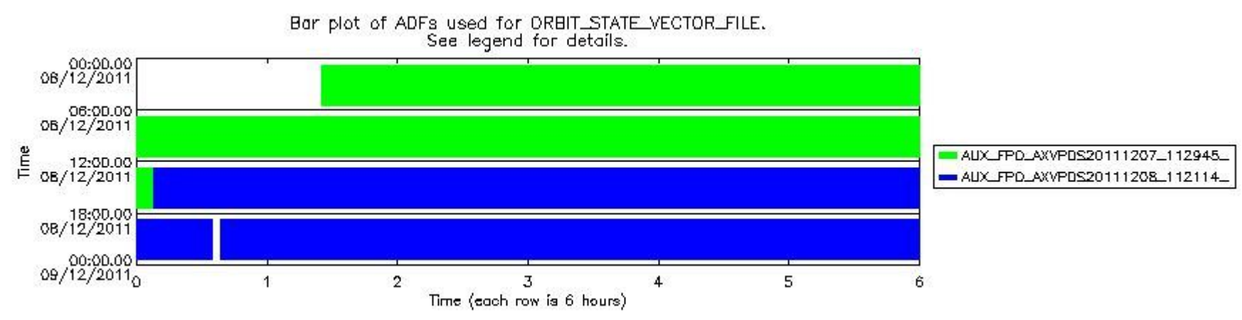
sciamachy_daily_report_level0_KSPT_L0_4504_N_20111208_8.PNG
