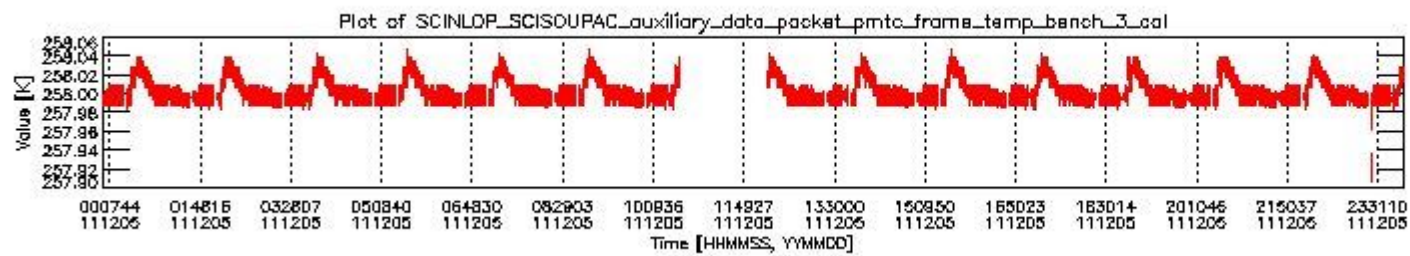
sciamachy_daily_report_level0_KSPT_L0_4504_N_20111205_2.PNG
