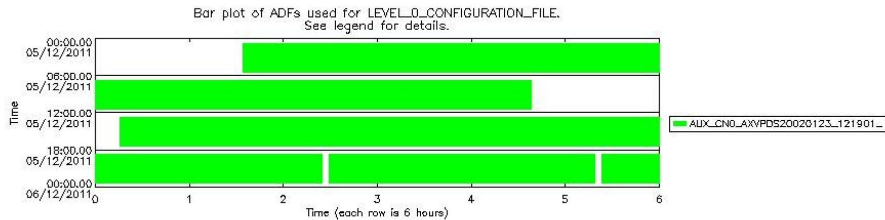
sciamachy_daily_report_level0_KSPT_L0_4504_N_20111205_7.PNG
