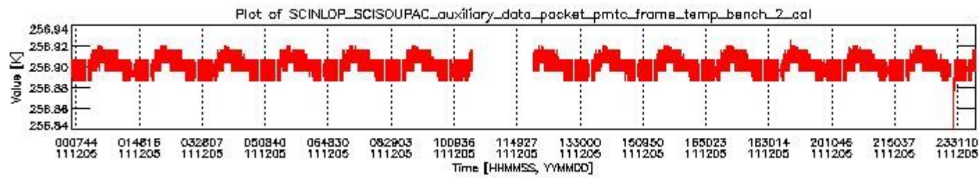
sciamachy_daily_report_level0_KSPT_L0_4504_N_20111205_1.PNG
