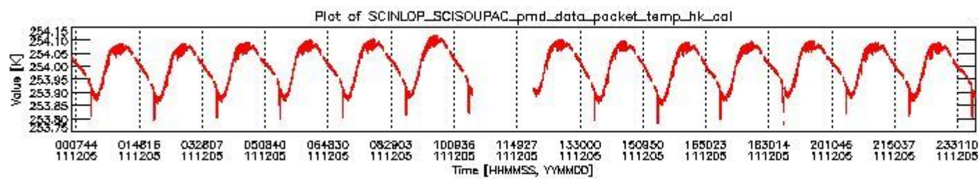
sciamachy_daily_report_level0_KSPT_L0_4504_N_20111205_3.PNG
