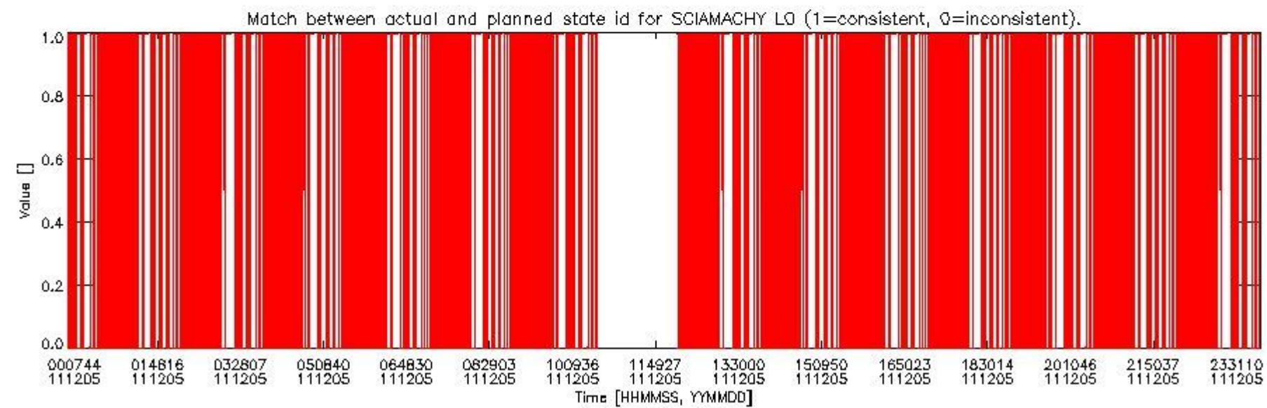
sciamachy_daily_report_level0_KSPT_L0_4504_N_20111205_5.PNG
