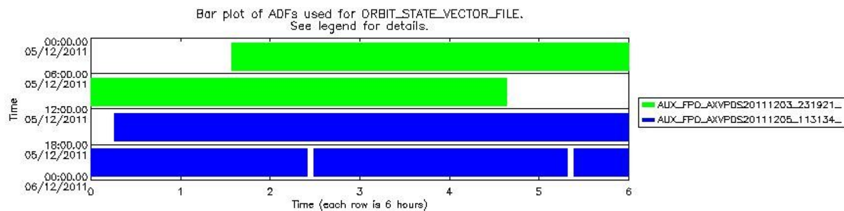
sciamachy_daily_report_level0_KSPT_L0_4504_N_20111205_8.PNG
