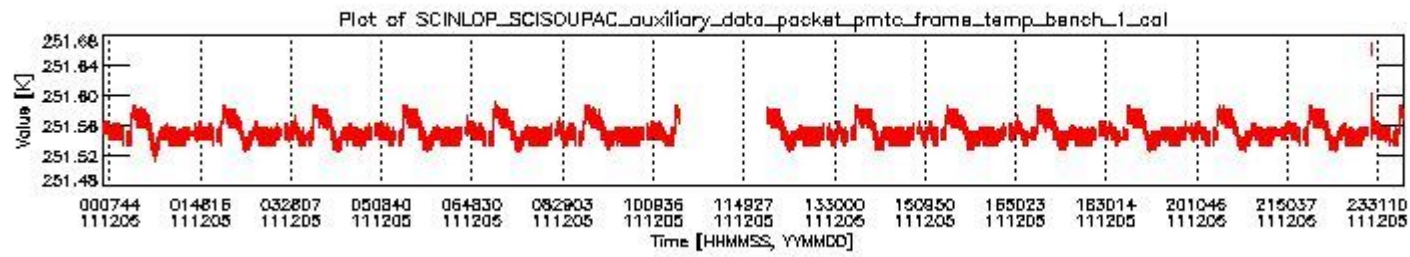
sciamachy_daily_report_level0_KSPT_L0_4504_N_20111205_0.PNG
