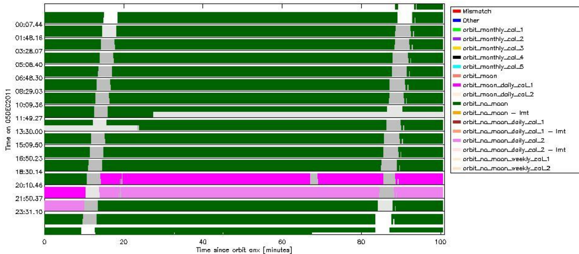
sciamachy_daily_report_level0_KSPT_L0_4504_N_20111205_6.PNG
