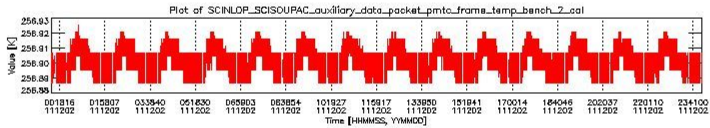
sciamachy_daily_report_level0_KSPT_L0_4504_N_20111202_1.PNG
