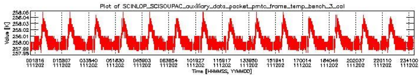
sciamachy_daily_report_level0_KSPT_L0_4504_N_20111202_2.PNG
