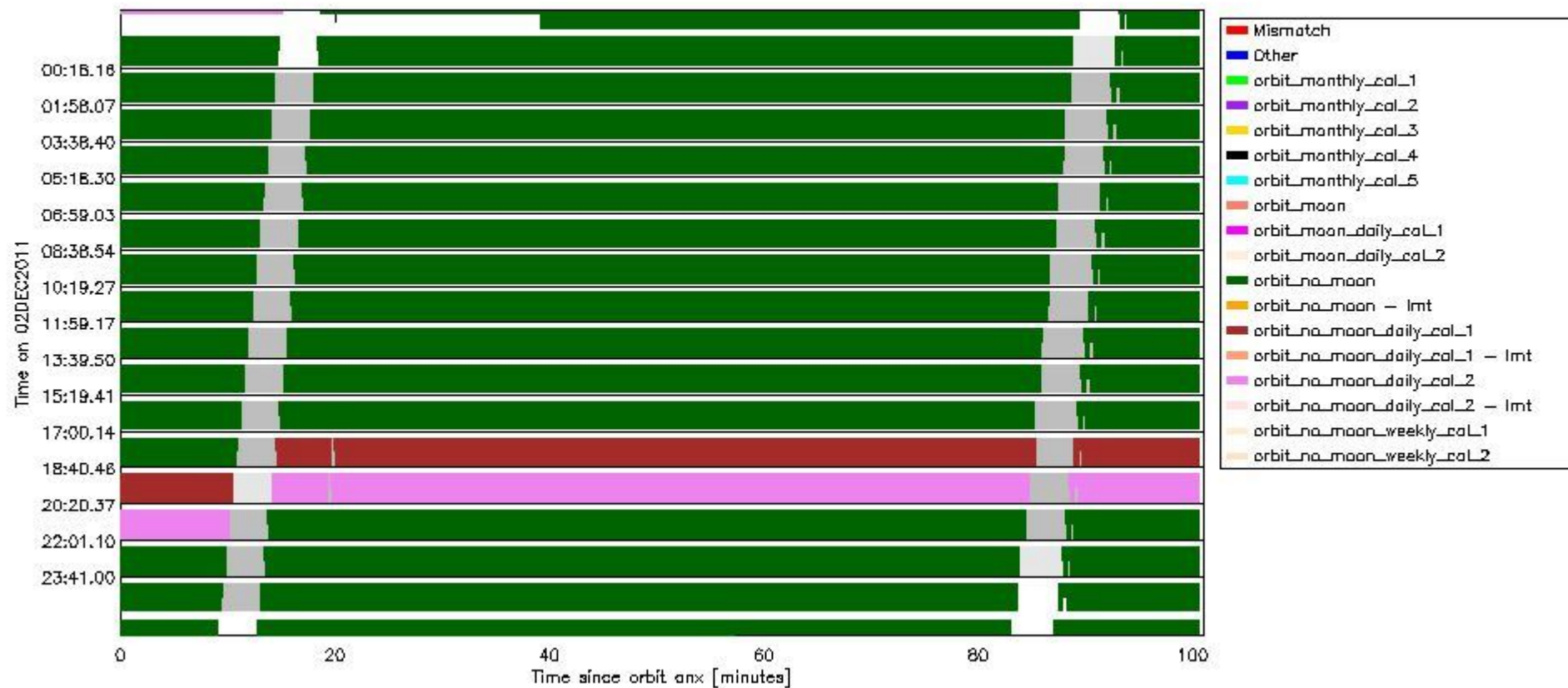
sciamachy_daily_report_level0_KSPT_L0_4504_N_20111202_6.PNG
