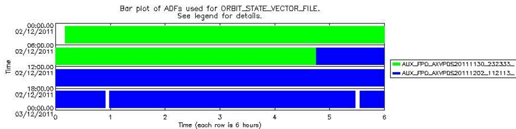
sciamachy_daily_report_level0_KSPT_L0_4504_N_20111202_8.PNG
