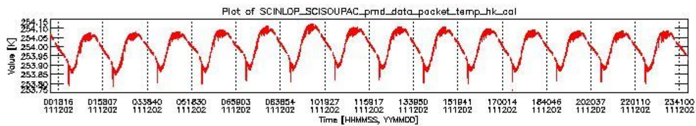
sciamachy_daily_report_level0_KSPT_L0_4504_N_20111202_3.PNG
