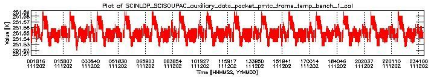
sciamachy_daily_report_level0_KSPT_L0_4504_N_20111202_0.PNG
