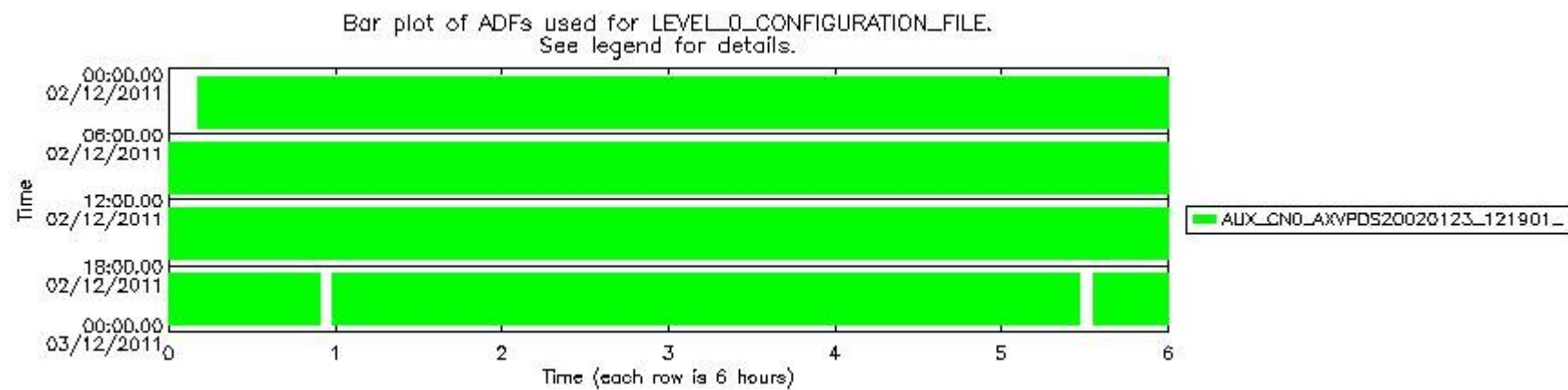
sciamachy_daily_report_level0_KSPT_L0_4504_N_20111202_7.PNG
