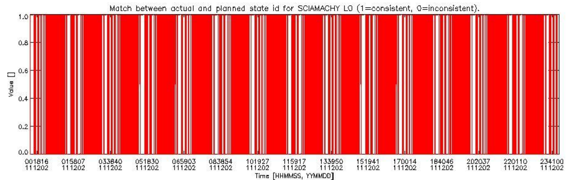
sciamachy_daily_report_level0_KSPT_L0_4504_N_20111202_5.PNG
