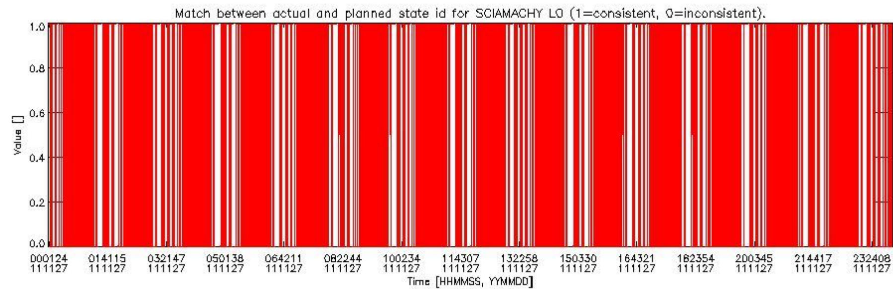
sciamachy_daily_report_level0_KSPT_L0_4504_N_20111127_5.PNG
