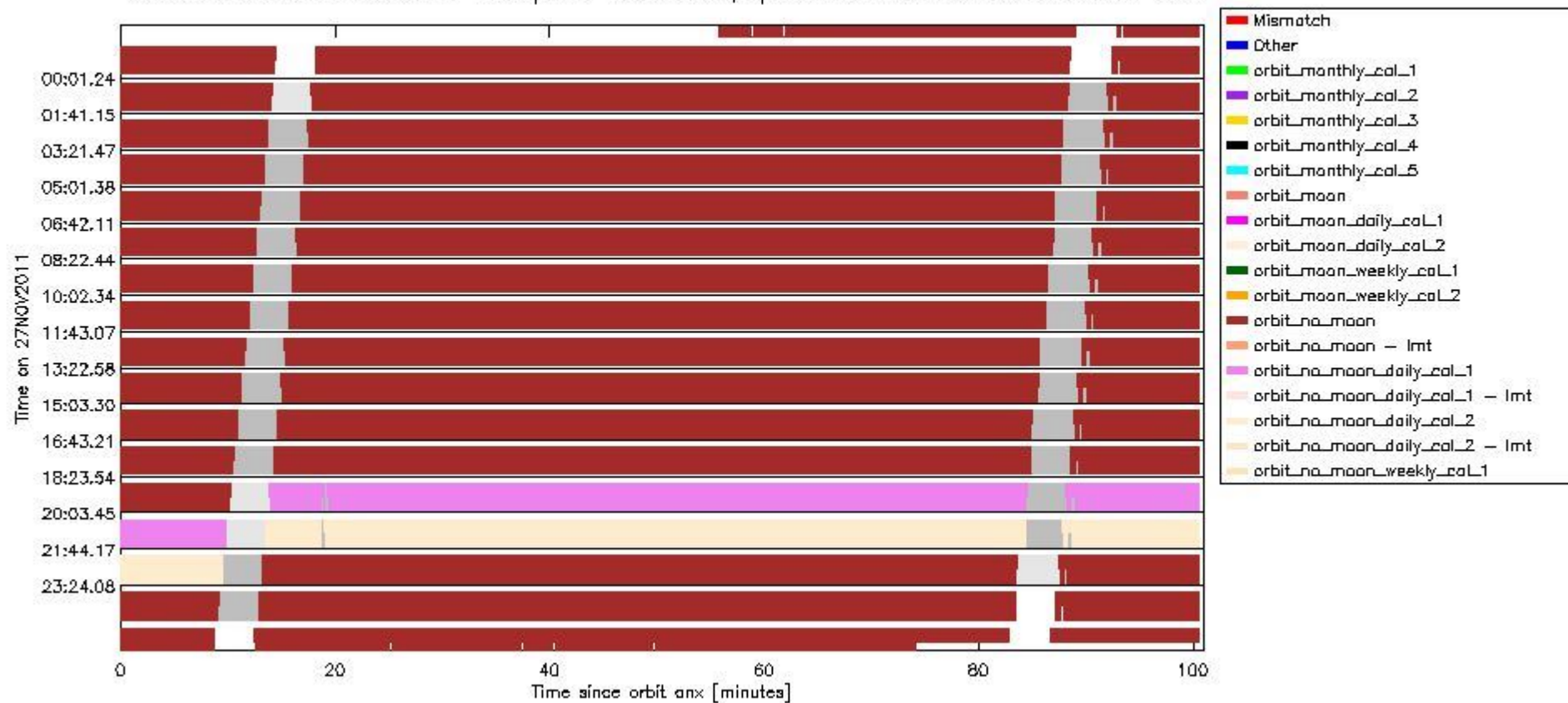
sciamachy_daily_report_level0_KSPT_L0_4504_N_20111127_6.PNG
