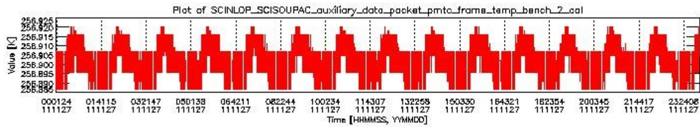
sciamachy_daily_report_level0_KSPT_L0_4504_N_20111127_1.PNG
