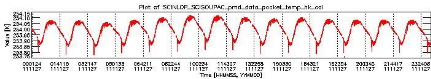
sciamachy_daily_report_level0_KSPT_L0_4504_N_20111127_3.PNG
