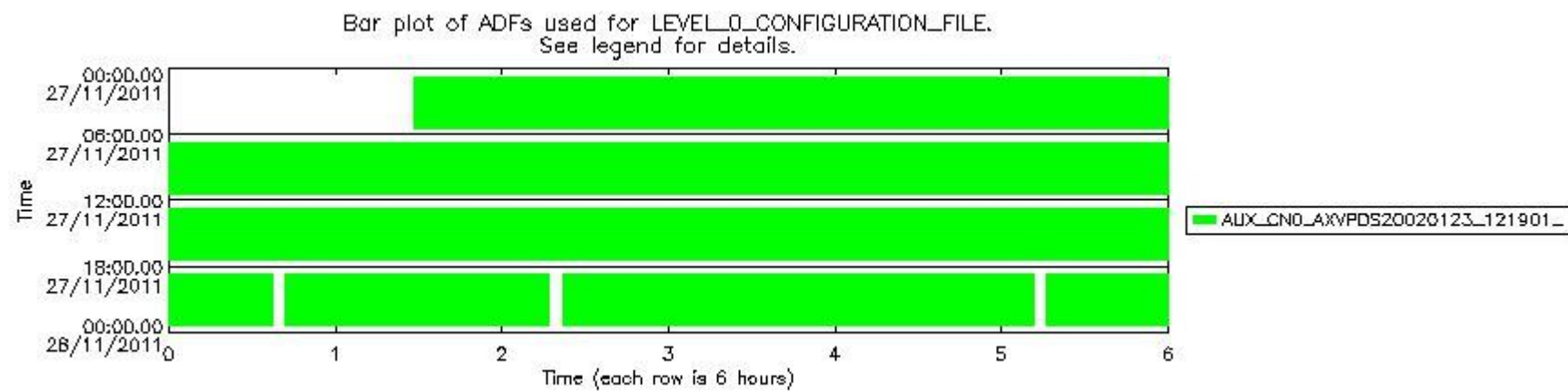
sciamachy_daily_report_level0_KSPT_L0_4504_N_20111127_7.PNG
