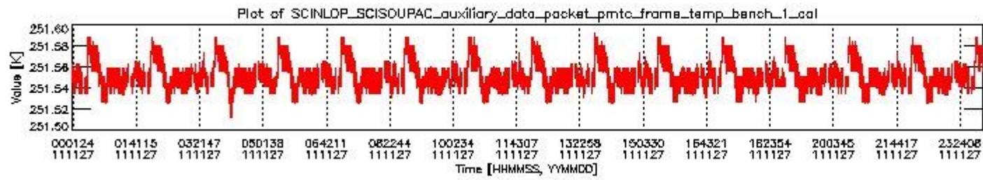
sciamachy_daily_report_level0_KSPT_L0_4504_N_20111127_0.PNG
