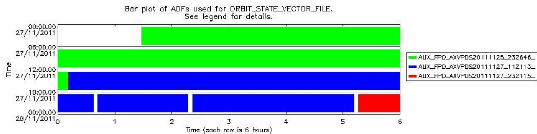
sciamachy_daily_report_level0_KSPT_L0_4504_N_20111127_8.PNG
