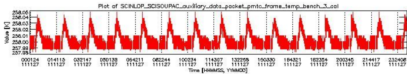
sciamachy_daily_report_level0_KSPT_L0_4504_N_20111127_2.PNG
