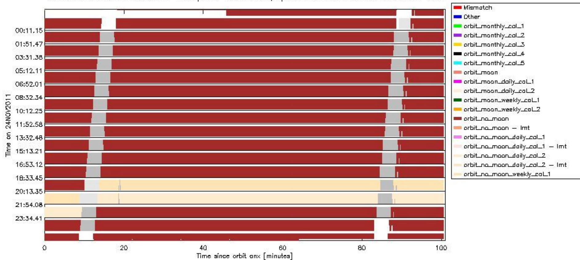
sciamachy_daily_report_level0_KSPT_L0_4504_N_20111124_6.PNG
