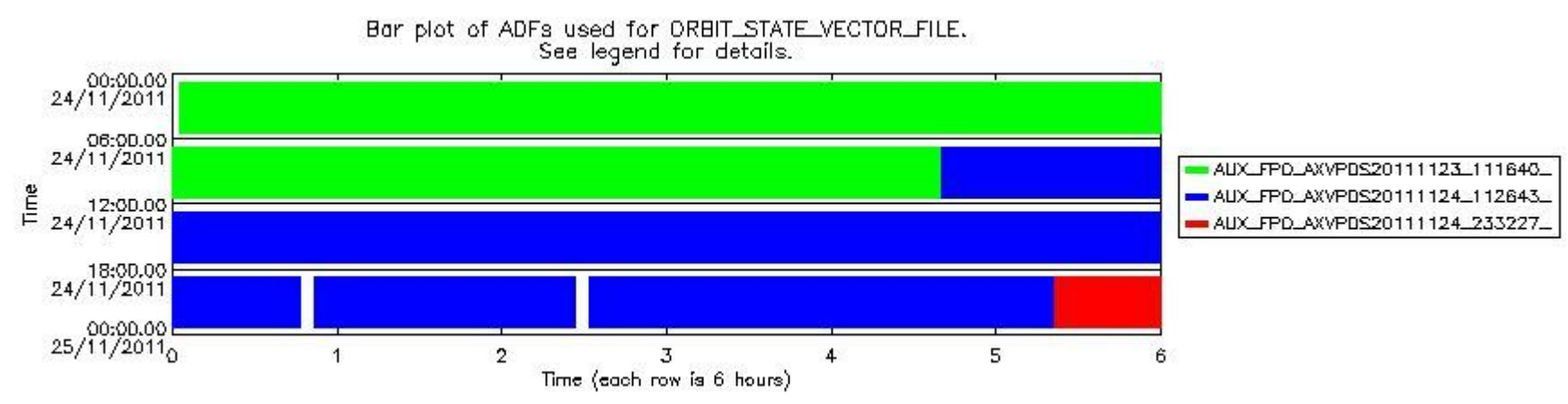
sciamachy_daily_report_level0_KSPT_L0_4504_N_20111124_8.PNG
