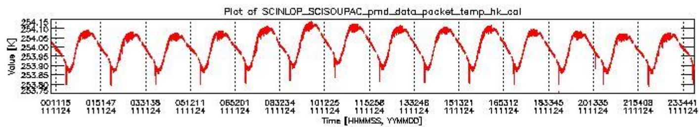
sciamachy_daily_report_level0_KSPT_L0_4504_N_20111124_3.PNG
