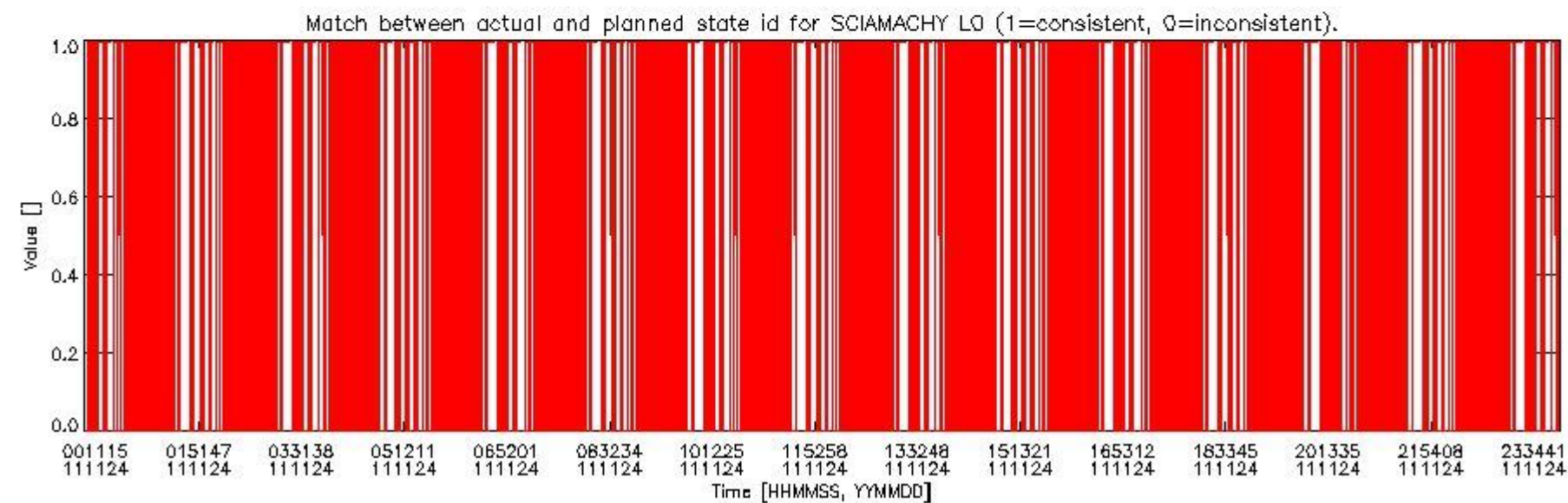
sciamachy_daily_report_level0_KSPT_L0_4504_N_20111124_5.PNG
