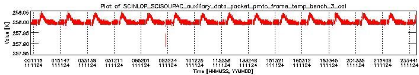
sciamachy_daily_report_level0_KSPT_L0_4504_N_20111124_2.PNG
