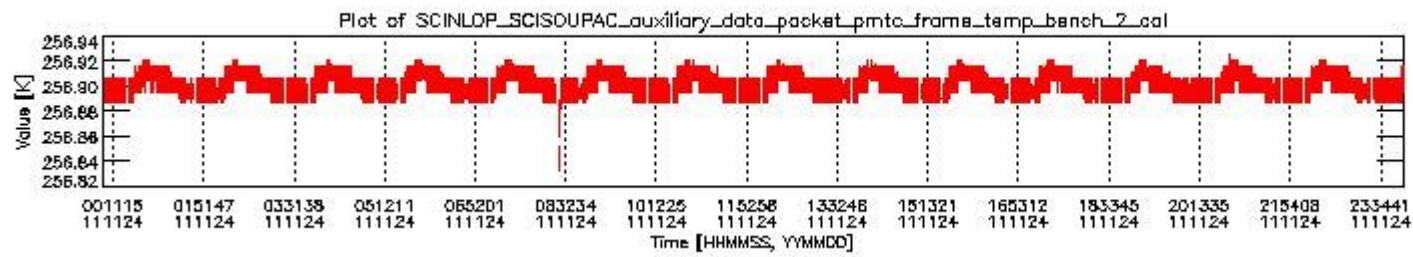
sciamachy_daily_report_level0_KSPT_L0_4504_N_20111124_1.PNG
