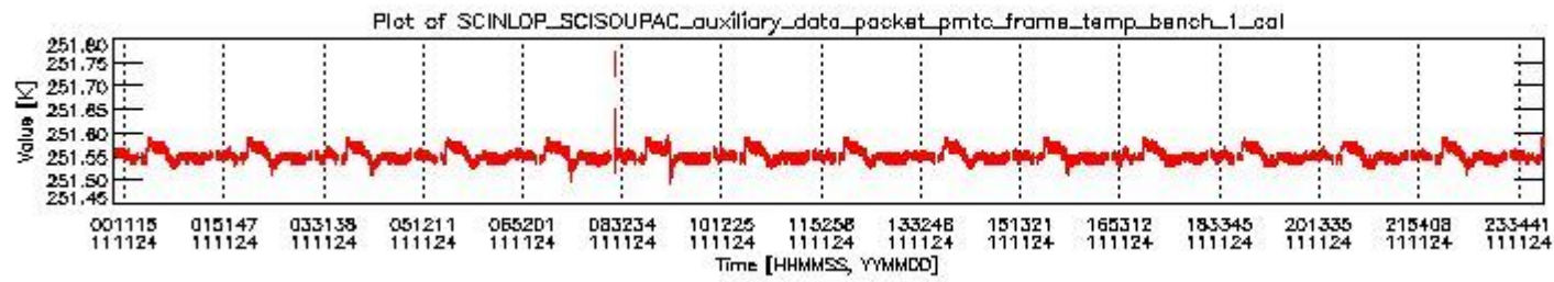
sciamachy_daily_report_level0_KSPT_L0_4504_N_20111124_0.PNG
