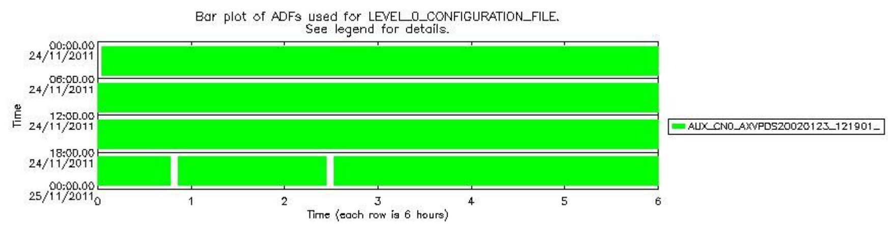
sciamachy_daily_report_level0_KSPT_L0_4504_N_20111124_7.PNG
