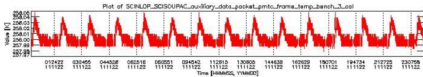
sciamachy_daily_report_level0_KSPT_L0_4504_N_20111122_2.PNG
