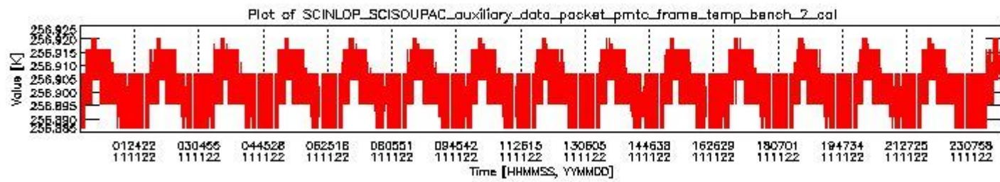
sciamachy_daily_report_level0_KSPT_L0_4504_N_20111122_1.PNG
