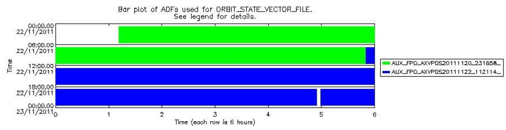
sciamachy_daily_report_level0_KSPT_L0_4504_N_20111122_8.PNG
