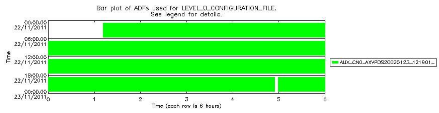
sciamachy_daily_report_level0_KSPT_L0_4504_N_20111122_7.PNG
