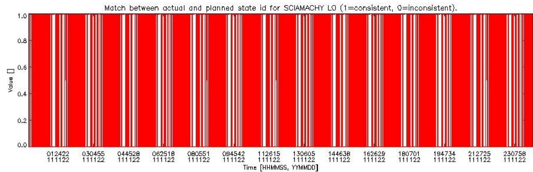
sciamachy_daily_report_level0_KSPT_L0_4504_N_20111122_5.PNG
