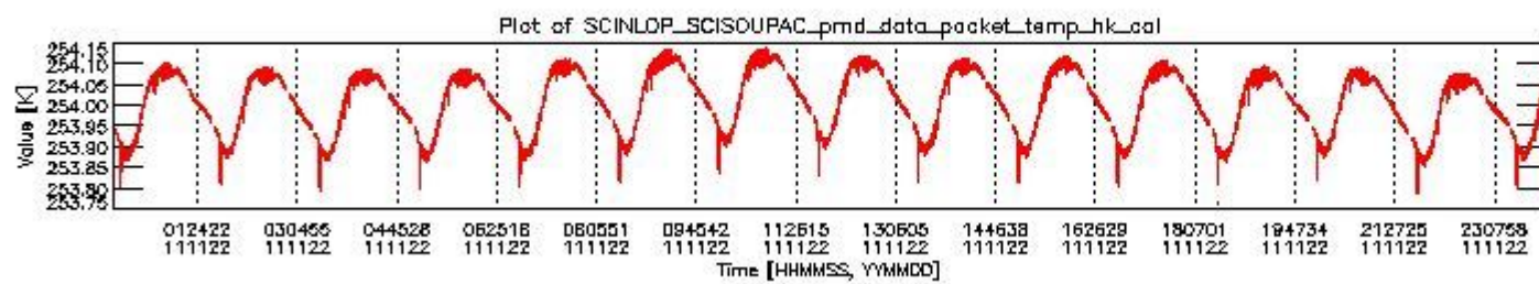
sciamachy_daily_report_level0_KSPT_L0_4504_N_20111122_3.PNG
