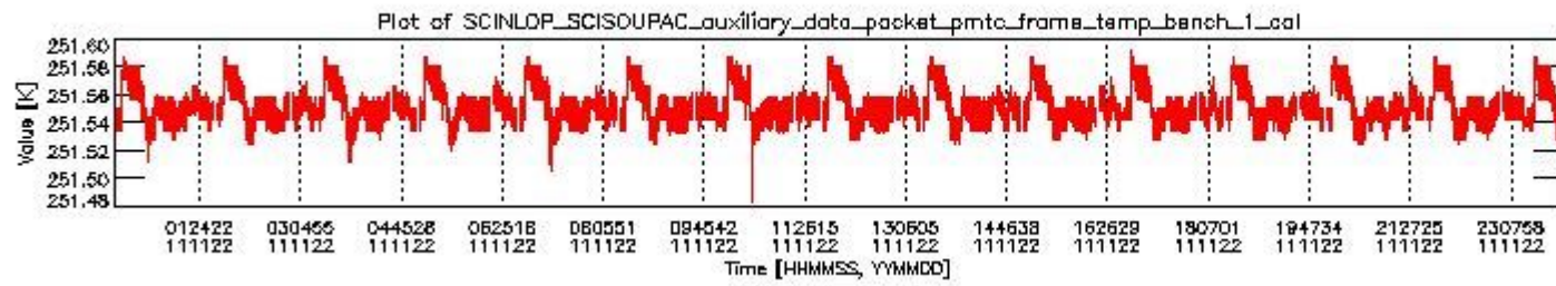
sciamachy_daily_report_level0_KSPT_L0_4504_N_20111122_0.PNG
