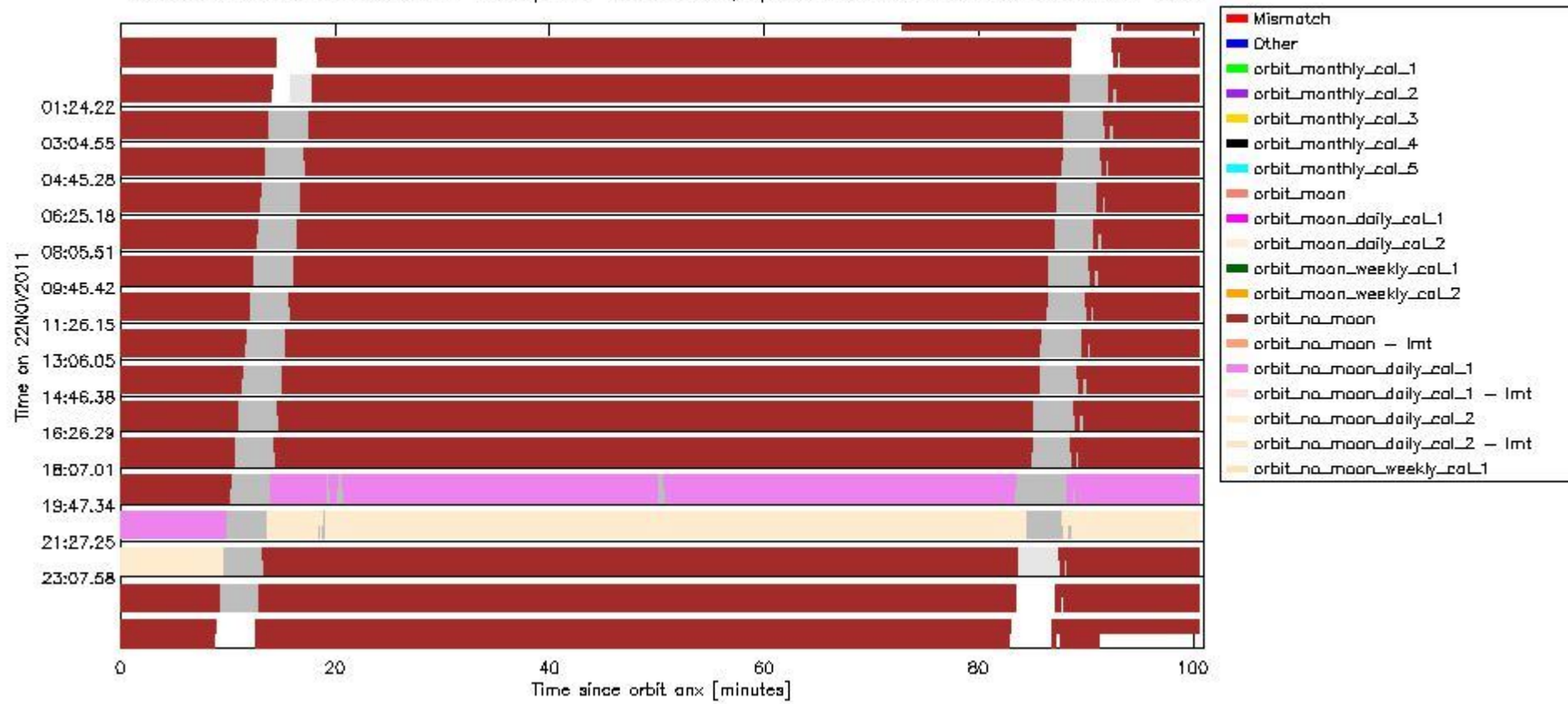
sciamachy_daily_report_level0_KSPT_L0_4504_N_20111122_6.PNG
