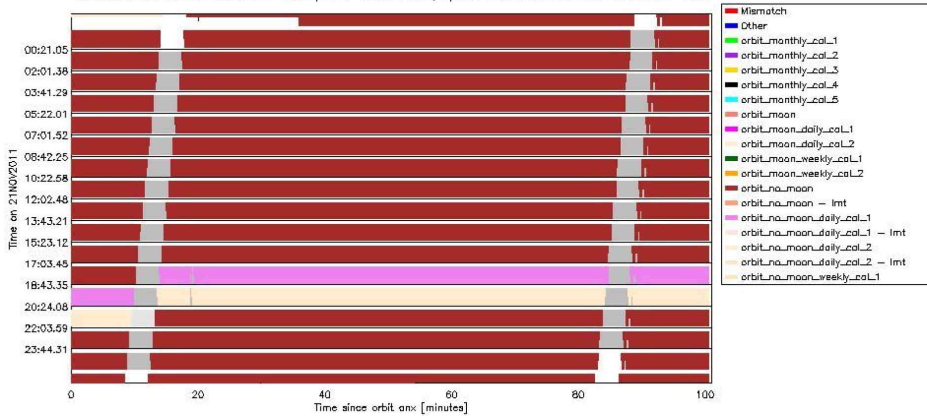
sciamachy_daily_report_level0_KSPT_L0_4504_N_20111121_6.PNG
