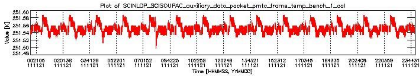
sciamachy_daily_report_level0_KSPT_L0_4504_N_20111121_0.PNG
