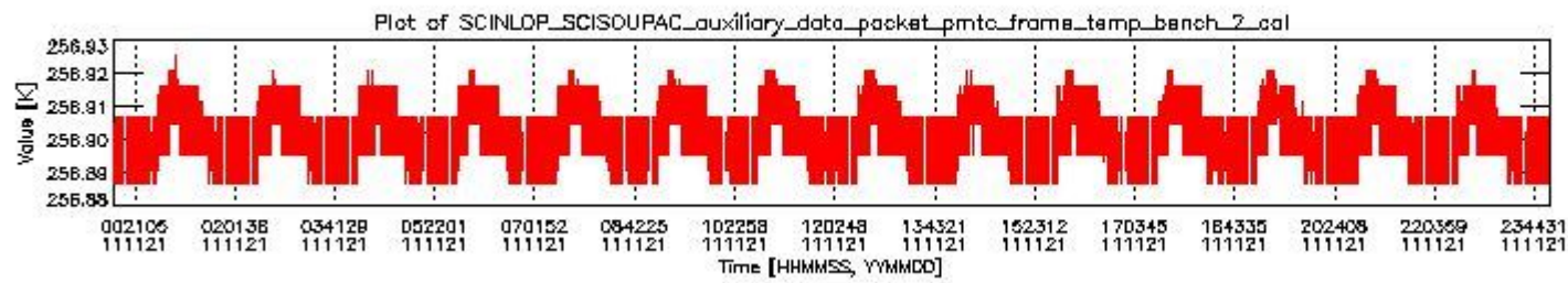
sciamachy_daily_report_level0_KSPT_L0_4504_N_20111121_1.PNG
