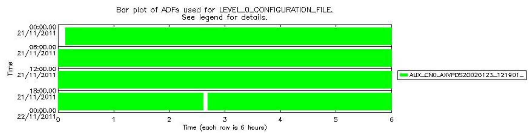
sciamachy_daily_report_level0_KSPT_L0_4504_N_20111121_7.PNG
