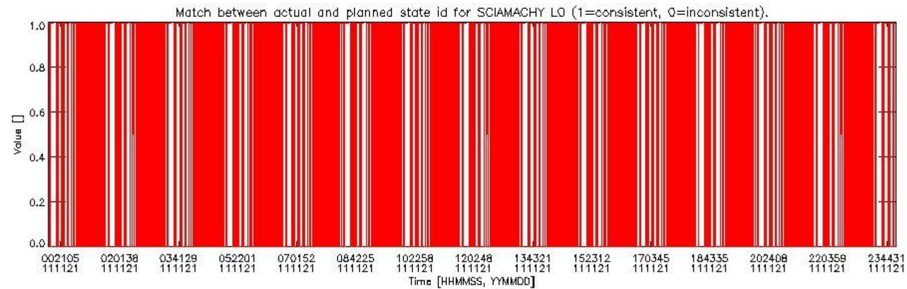
sciamachy_daily_report_level0_KSPT_L0_4504_N_20111121_5.PNG
