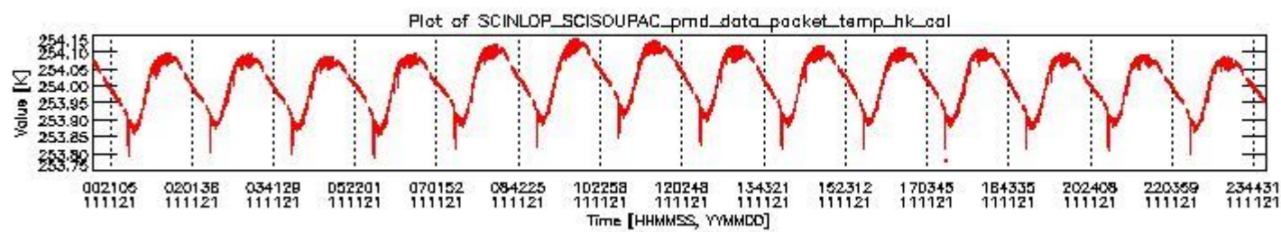
sciamachy_daily_report_level0_KSPT_L0_4504_N_20111121_3.PNG
