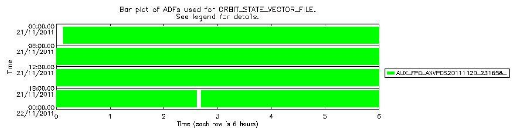
sciamachy_daily_report_level0_KSPT_L0_4504_N_20111121_8.PNG
