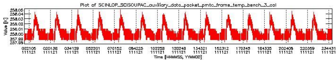
sciamachy_daily_report_level0_KSPT_L0_4504_N_20111121_2.PNG
