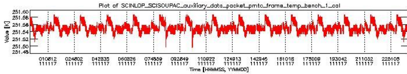
sciamachy_daily_report_level0_KSPT_L0_4504_N_20111117_0.PNG
