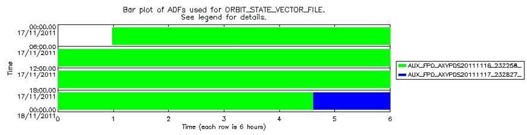
sciamachy_daily_report_level0_KSPT_L0_4504_N_20111117_8.PNG
