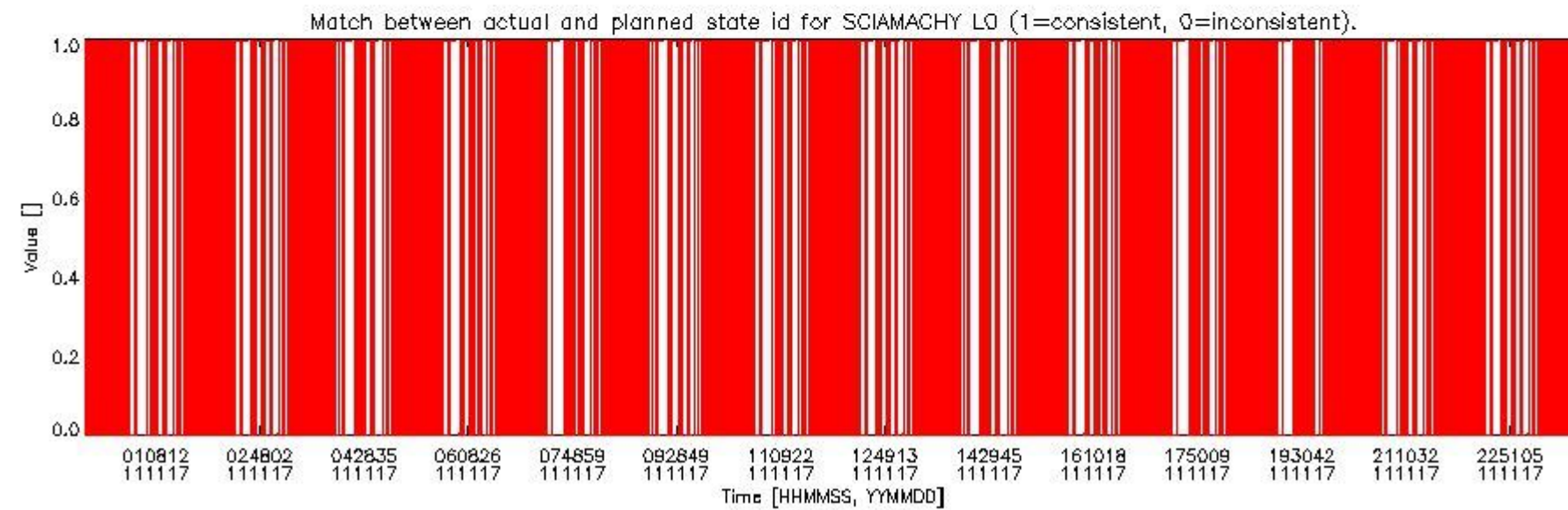
sciamachy_daily_report_level0_KSPT_L0_4504_N_20111117_5.PNG
