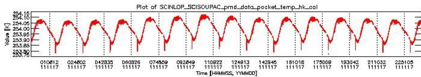
sciamachy_daily_report_level0_KSPT_L0_4504_N_20111117_3.PNG
