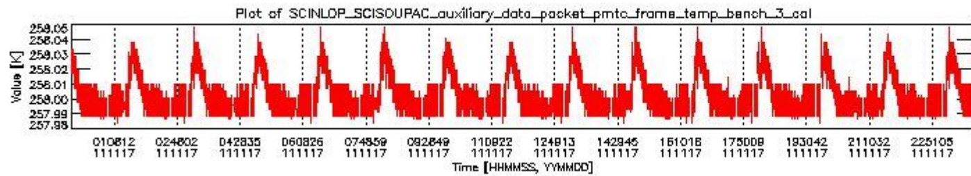
sciamachy_daily_report_level0_KSPT_L0_4504_N_20111117_2.PNG
