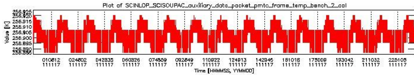
sciamachy_daily_report_level0_KSPT_L0_4504_N_20111117_1.PNG
