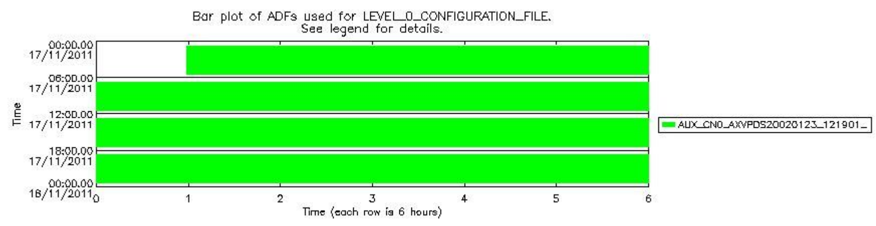
sciamachy_daily_report_level0_KSPT_L0_4504_N_20111117_7.PNG
