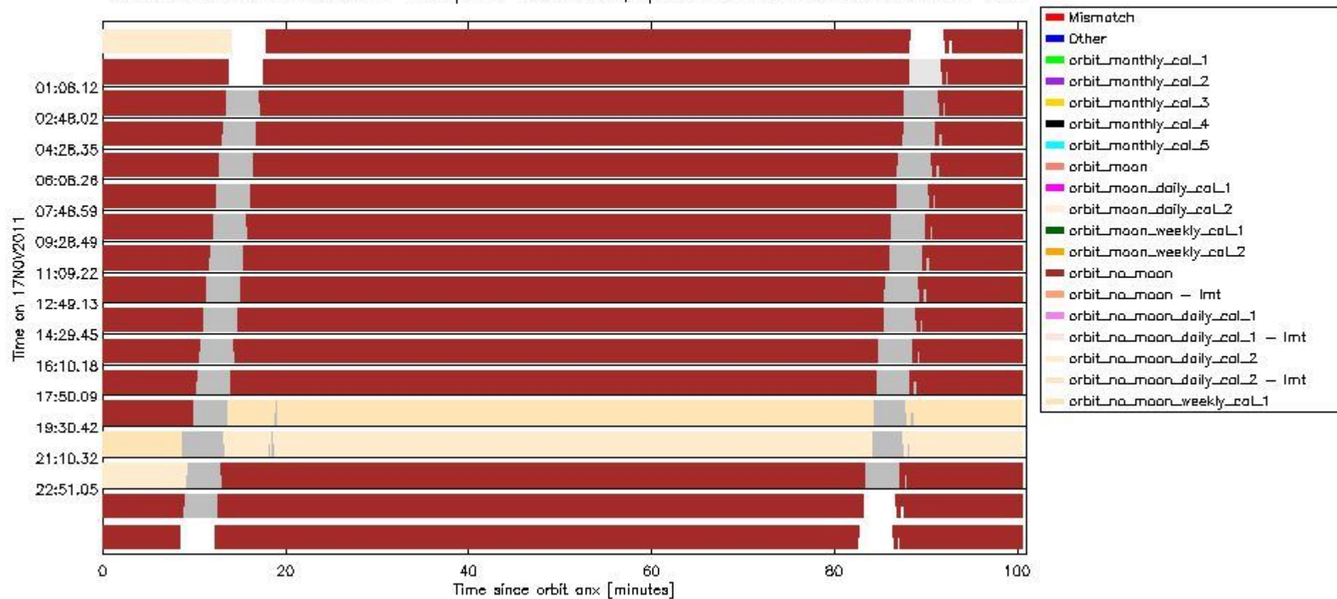
sciamachy_daily_report_level0_KSPT_L0_4504_N_20111117_6.PNG
