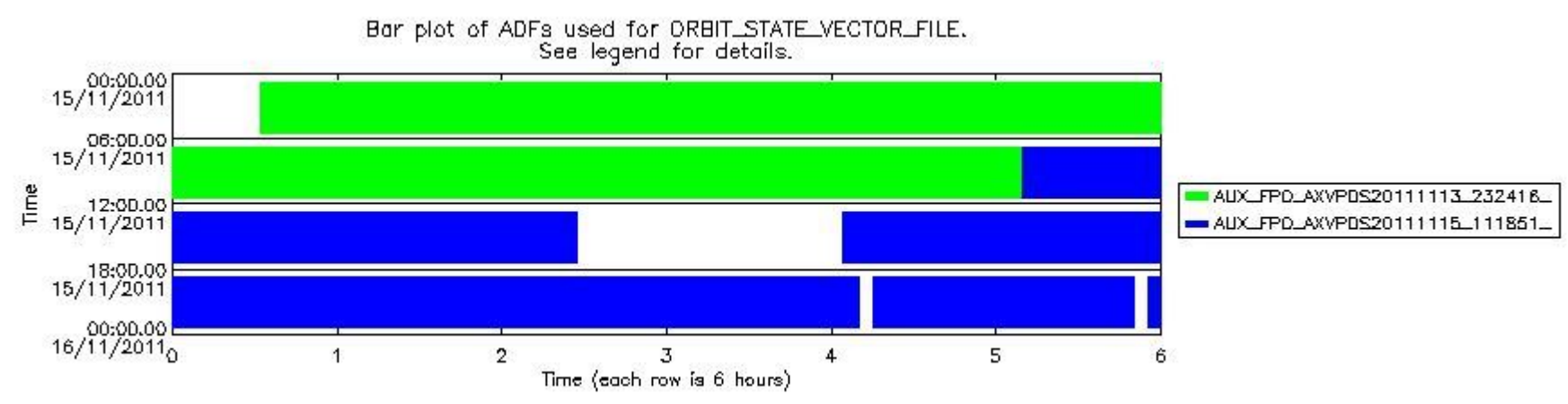
sciamachy_daily_report_level0_KSPT_L0_4504_N_20111115_8.PNG
