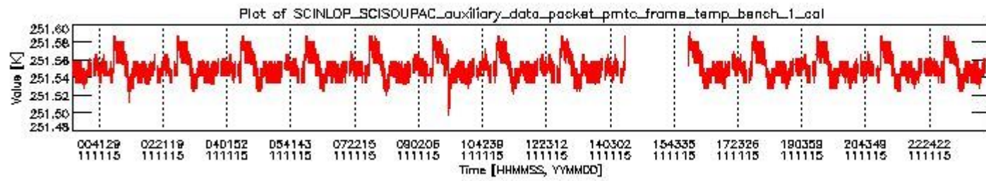
sciamachy_daily_report_level0_KSPT_L0_4504_N_20111115_0.PNG
