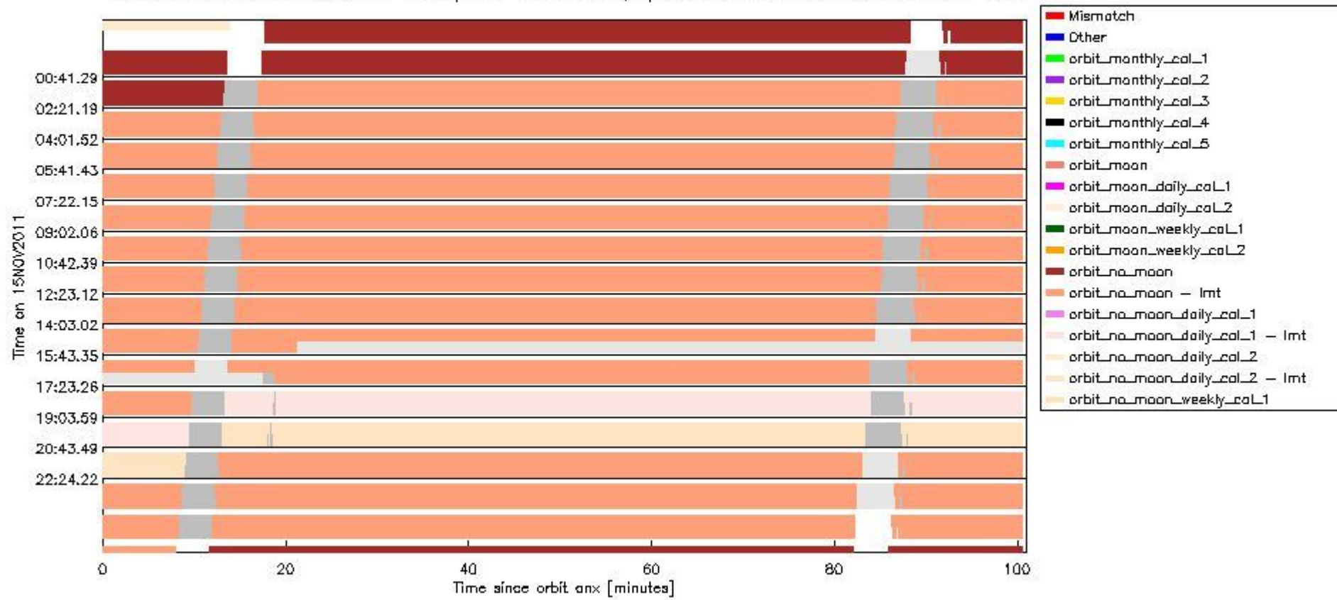
sciamachy_daily_report_level0_KSPT_L0_4504_N_20111115_6.PNG
