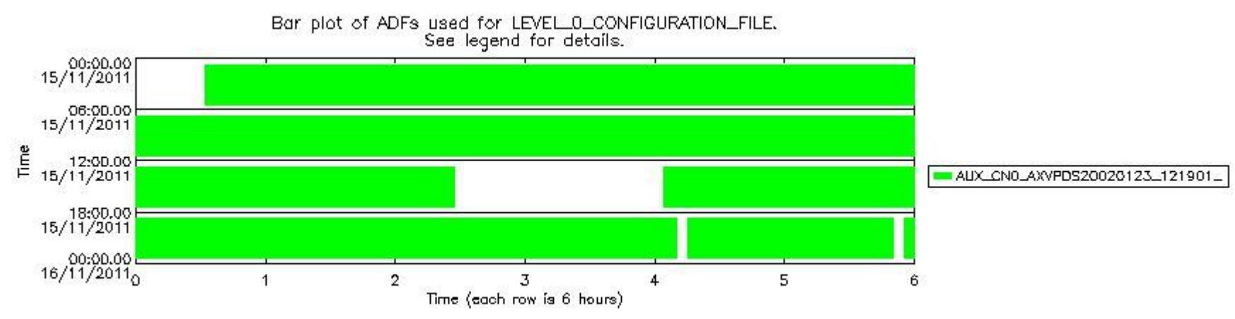
sciamachy_daily_report_level0_KSPT_L0_4504_N_20111115_7.PNG
