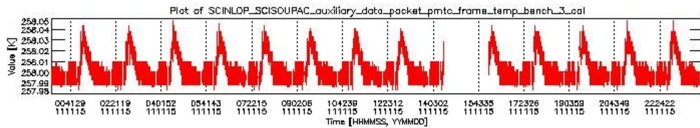
sciamachy_daily_report_level0_KSPT_L0_4504_N_20111115_2.PNG
