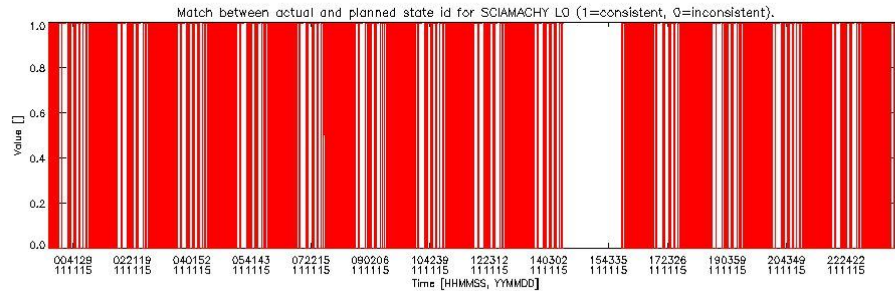
sciamachy_daily_report_level0_KSPT_L0_4504_N_20111115_5.PNG
