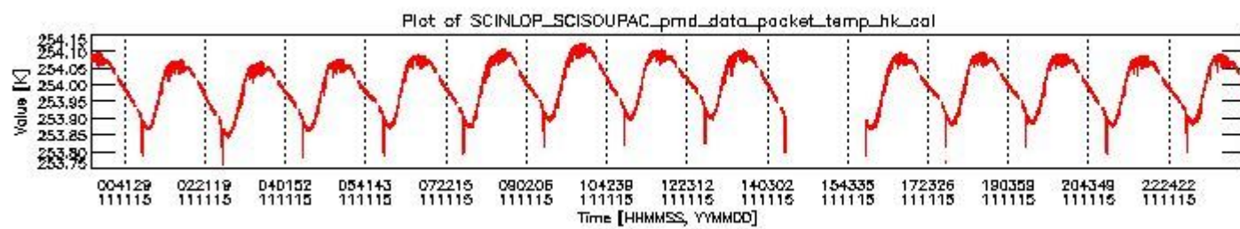
sciamachy_daily_report_level0_KSPT_L0_4504_N_20111115_3.PNG
