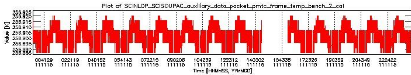
sciamachy_daily_report_level0_KSPT_L0_4504_N_20111115_1.PNG
