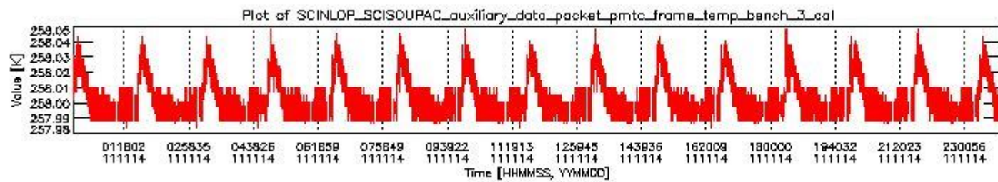
sciamachy_daily_report_level0_KSPT_L0_4504_N_20111114_2.PNG
