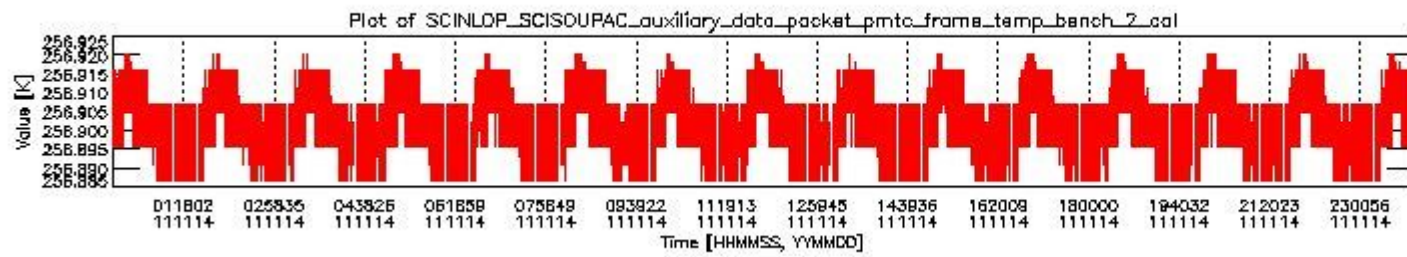
sciamachy_daily_report_level0_KSPT_L0_4504_N_20111114_1.PNG
