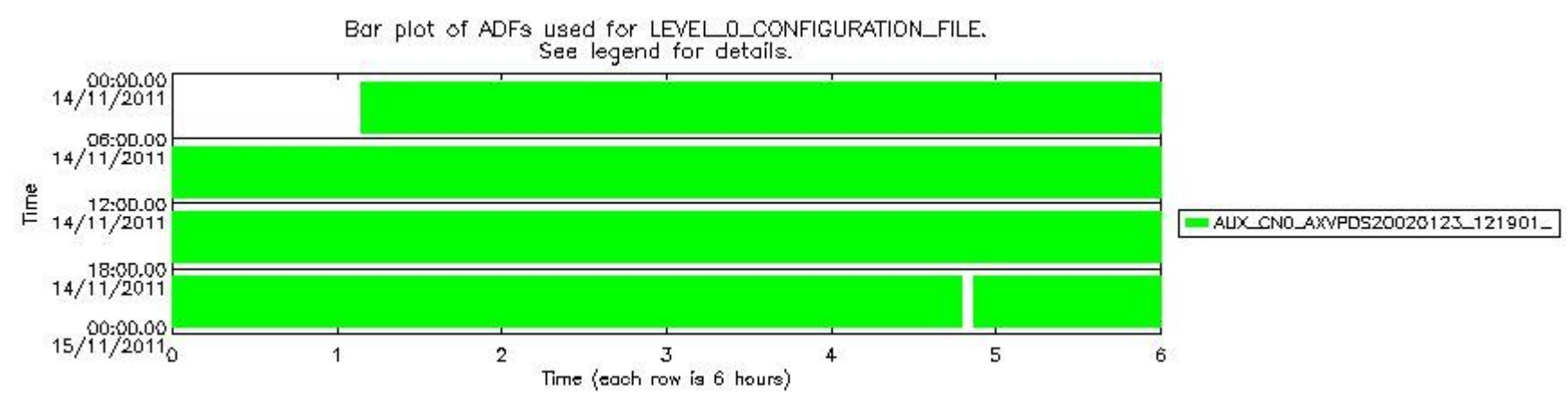
sciamachy_daily_report_level0_KSPT_L0_4504_N_20111114_7.PNG
