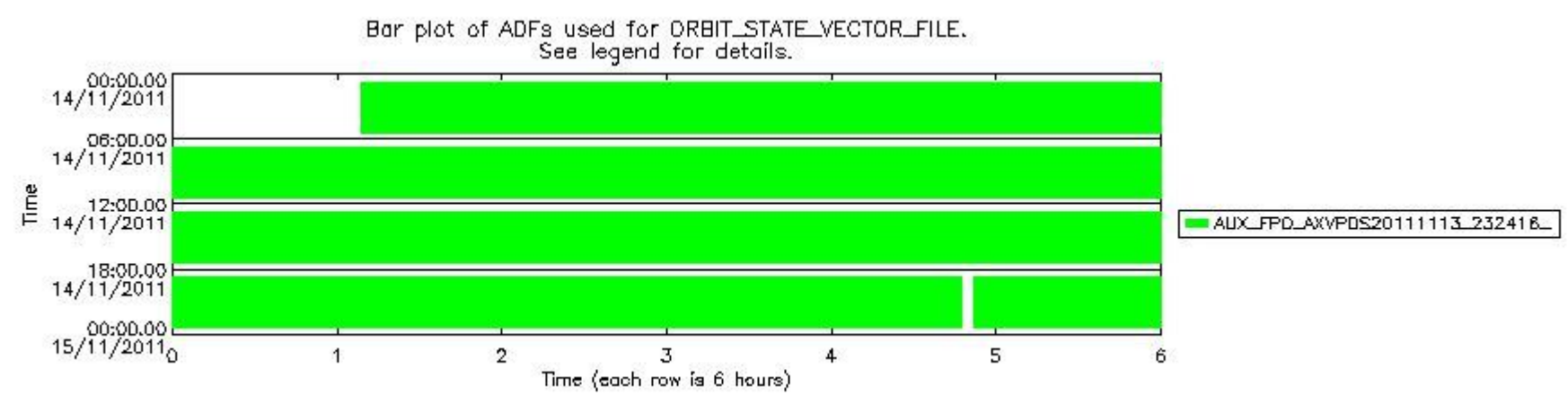
sciamachy_daily_report_level0_KSPT_L0_4504_N_20111114_8.PNG
