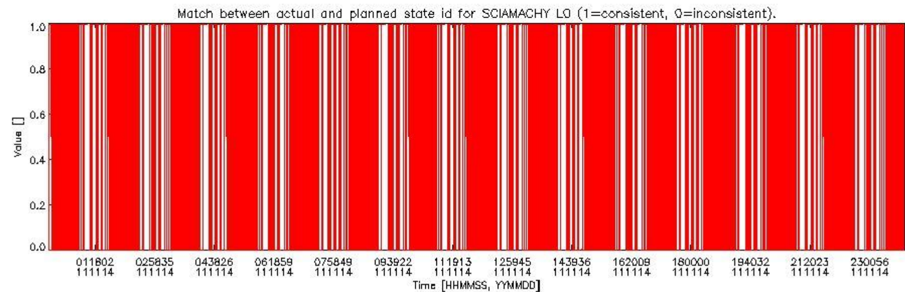
sciamachy_daily_report_level0_KSPT_L0_4504_N_20111114_5.PNG
