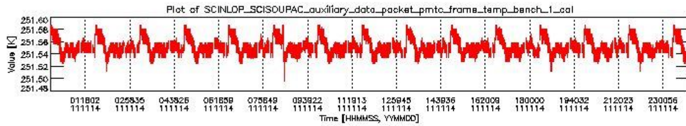
sciamachy_daily_report_level0_KSPT_L0_4504_N_20111114_0.PNG
