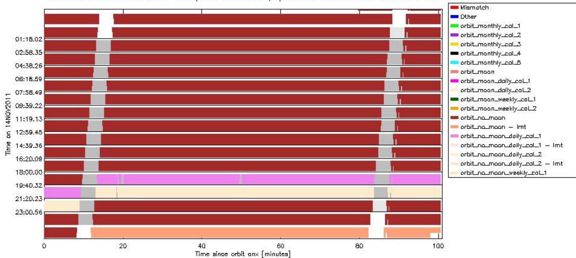
sciamachy_daily_report_level0_KSPT_L0_4504_N_20111114_6.PNG
