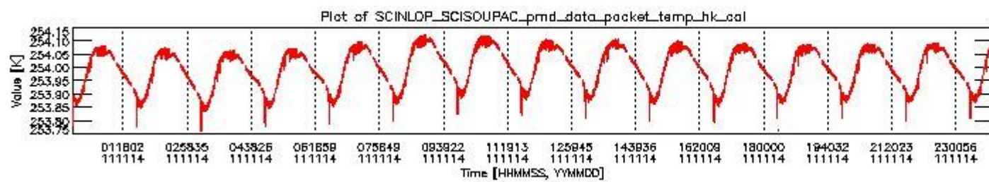
sciamachy_daily_report_level0_KSPT_L0_4504_N_20111114_3.PNG
