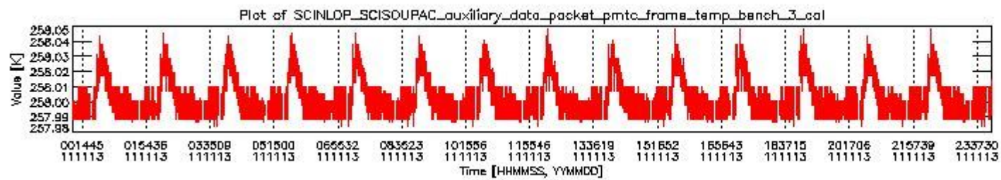
sciamachy_daily_report_level0_KSPT_L0_4504_N_20111113_2.PNG
