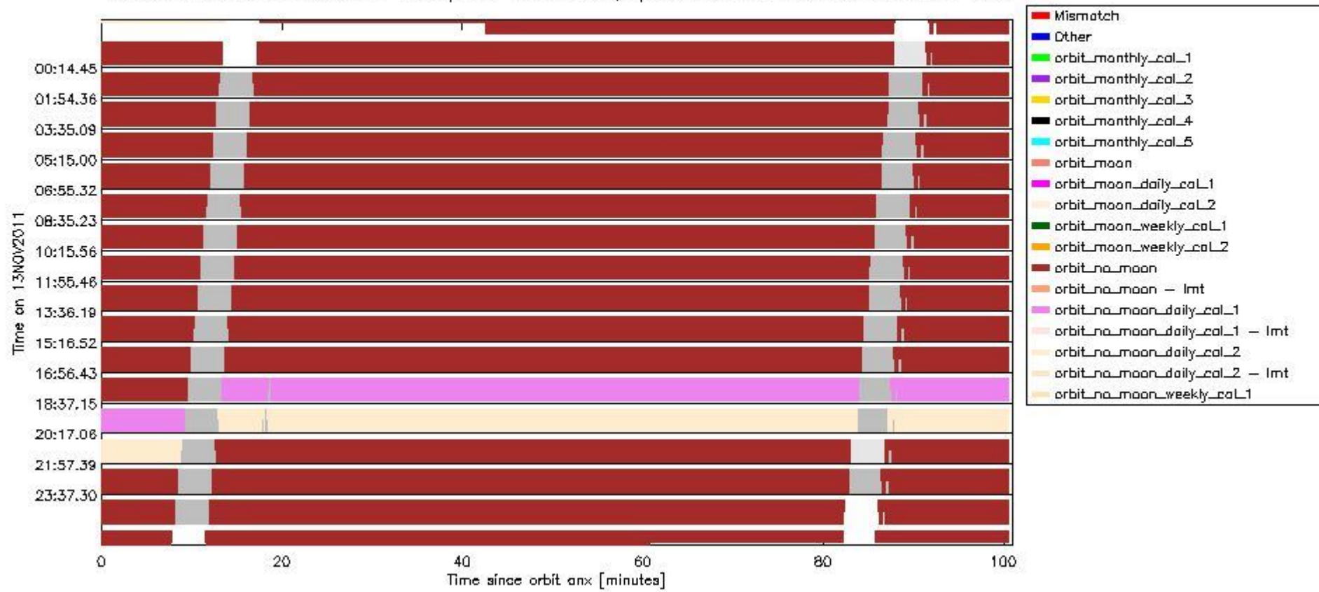
sciamachy_daily_report_level0_KSPT_L0_4504_N_20111113_6.PNG
