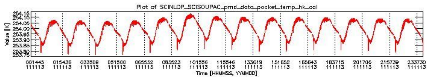
sciamachy_daily_report_level0_KSPT_L0_4504_N_20111113_3.PNG
