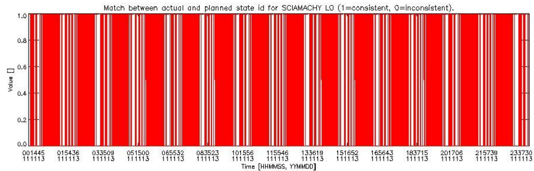
sciamachy_daily_report_level0_KSPT_L0_4504_N_20111113_5.PNG
