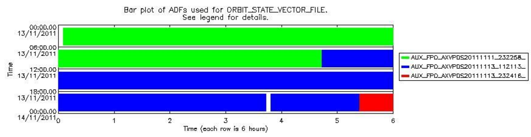
sciamachy_daily_report_level0_KSPT_L0_4504_N_20111113_8.PNG
