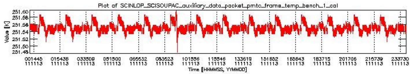
sciamachy_daily_report_level0_KSPT_L0_4504_N_20111113_0.PNG
