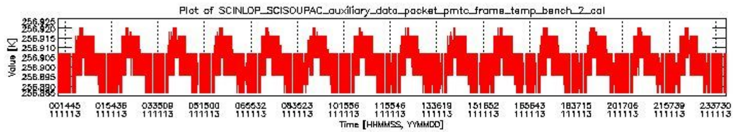
sciamachy_daily_report_level0_KSPT_L0_4504_N_20111113_1.PNG
