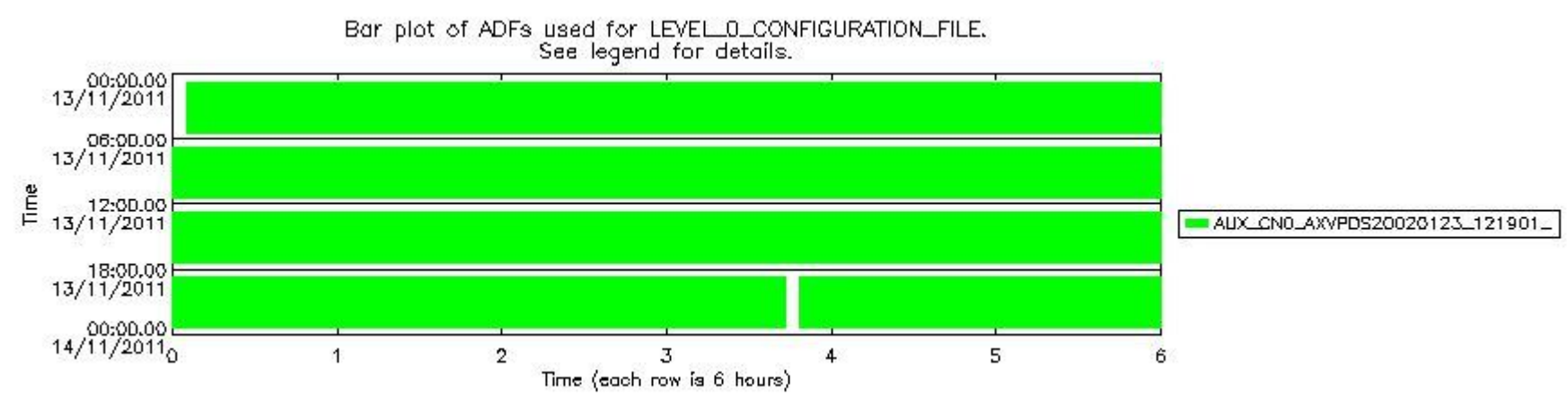
sciamachy_daily_report_level0_KSPT_L0_4504_N_20111113_7.PNG
