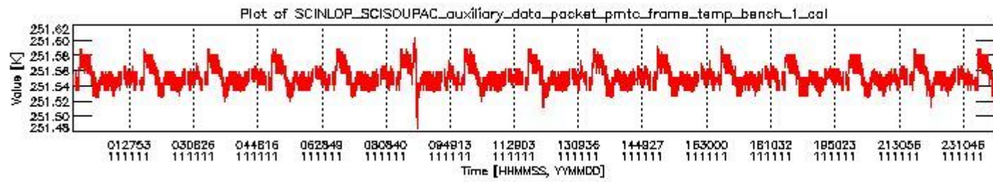
sciamachy_daily_report_level0_KSPT_L0_4504_N_20111111_0.PNG
