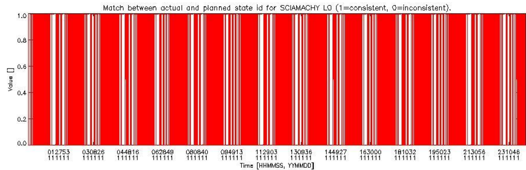
sciamachy_daily_report_level0_KSPT_L0_4504_N_20111111_5.PNG
