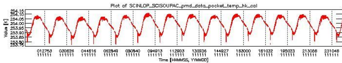
sciamachy_daily_report_level0_KSPT_L0_4504_N_20111111_3.PNG
