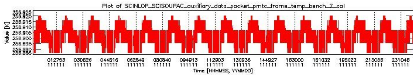
sciamachy_daily_report_level0_KSPT_L0_4504_N_20111111_1.PNG
