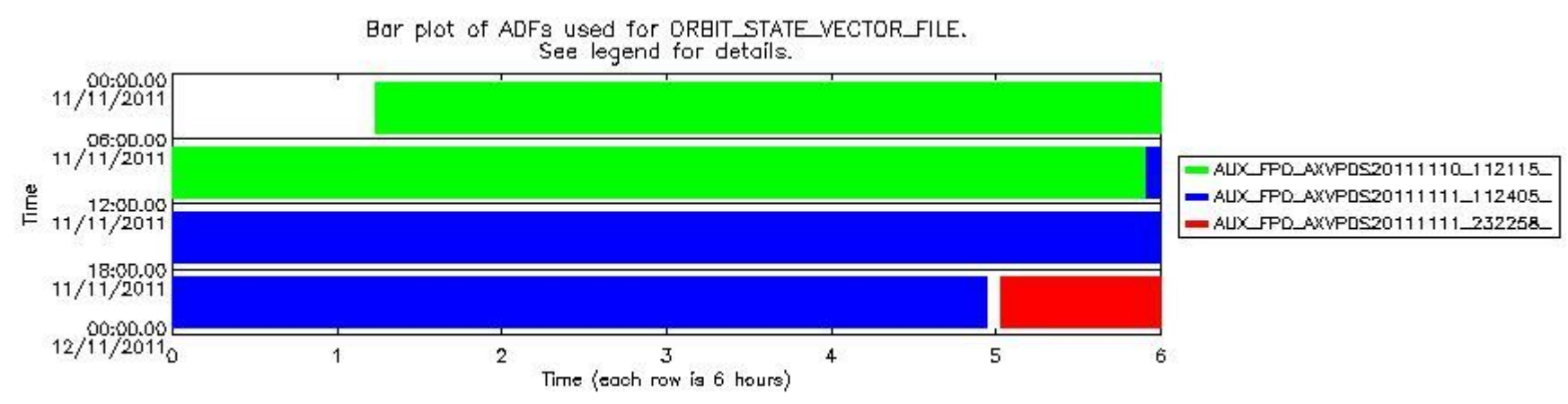
sciamachy_daily_report_level0_KSPT_L0_4504_N_20111111_8.PNG
