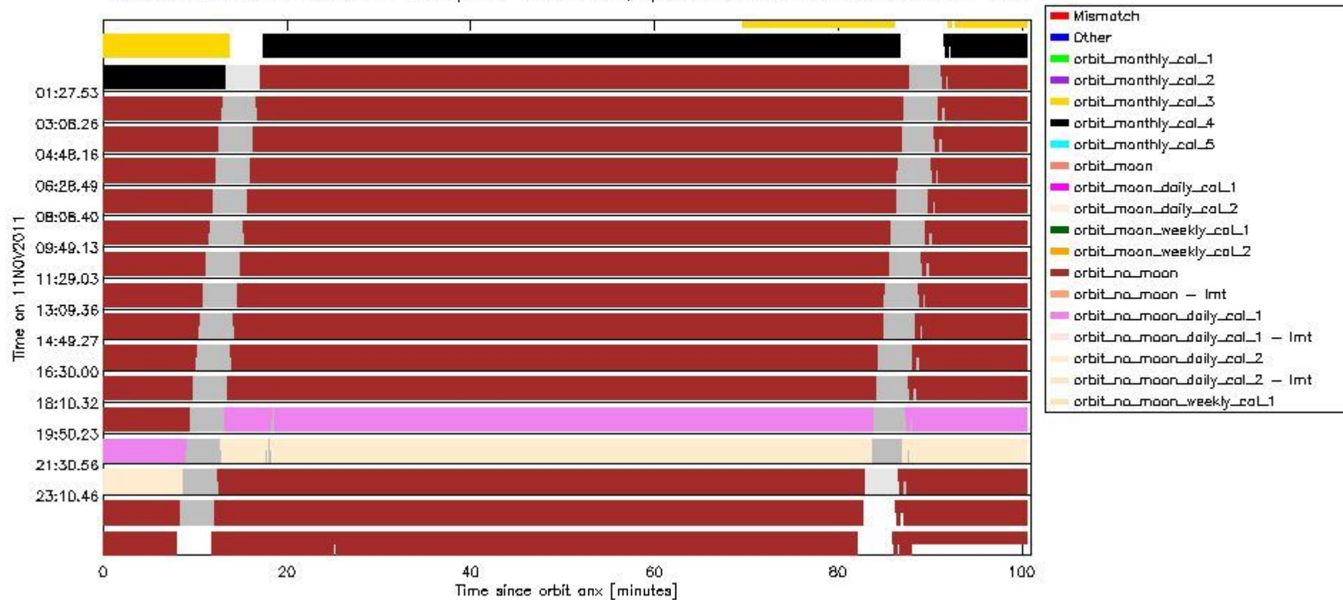
sciamachy_daily_report_level0_KSPT_L0_4504_N_20111111_6.PNG
