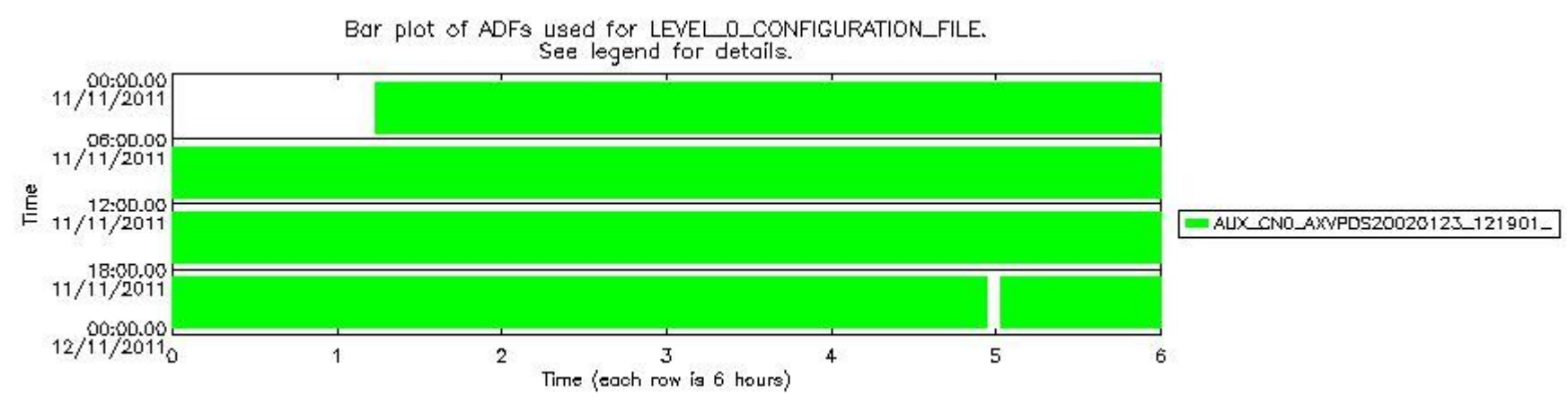
sciamachy_daily_report_level0_KSPT_L0_4504_N_20111111_7.PNG
