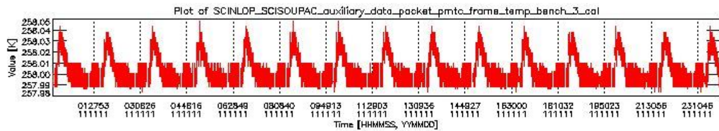
sciamachy_daily_report_level0_KSPT_L0_4504_N_20111111_2.PNG
