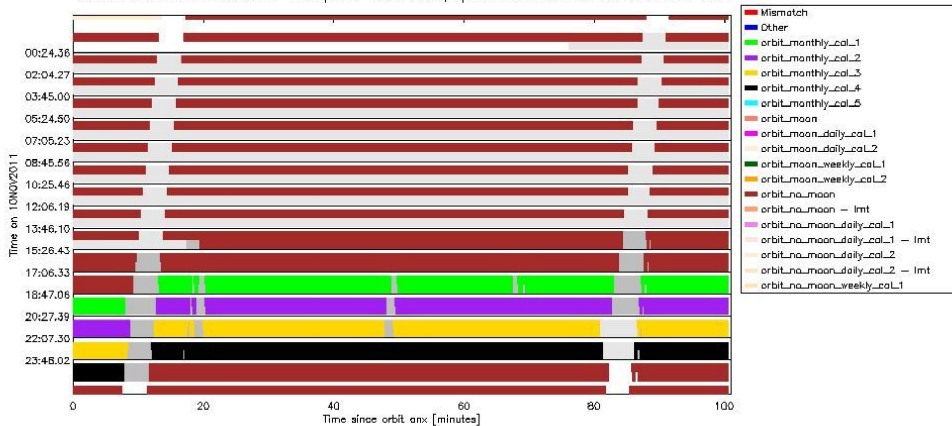
sciamachy_daily_report_level0_KSPT_L0_4504_N_20111110_6.PNG
