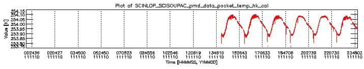
sciamachy_daily_report_level0_KSPT_L0_4504_N_20111110_3.PNG
