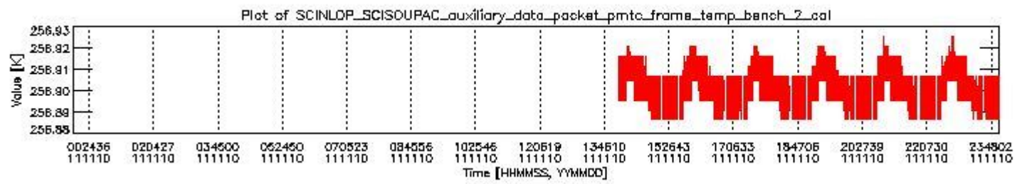
sciamachy_daily_report_level0_KSPT_L0_4504_N_20111110_1.PNG
