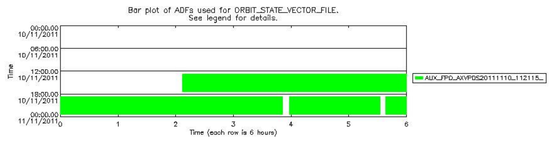
sciamachy_daily_report_level0_KSPT_L0_4504_N_20111110_8.PNG
