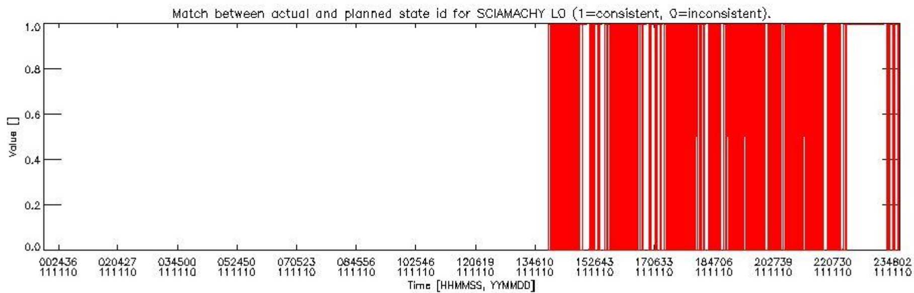
sciamachy_daily_report_level0_KSPT_L0_4504_N_20111110_5.PNG
