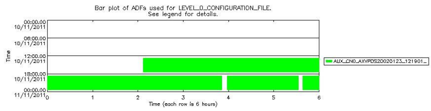
sciamachy_daily_report_level0_KSPT_L0_4504_N_20111110_7.PNG
