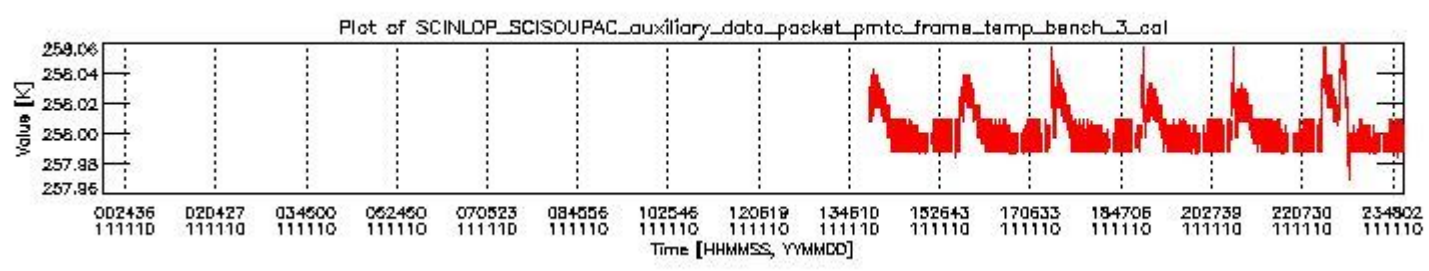
sciamachy_daily_report_level0_KSPT_L0_4504_N_20111110_2.PNG
