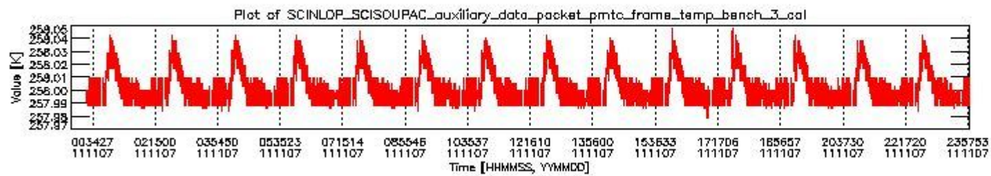
sciamachy_daily_report_level0_KSPT_L0_4504_N_20111107_2.PNG
