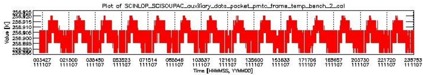
sciamachy_daily_report_level0_KSPT_L0_4504_N_20111107_1.PNG
