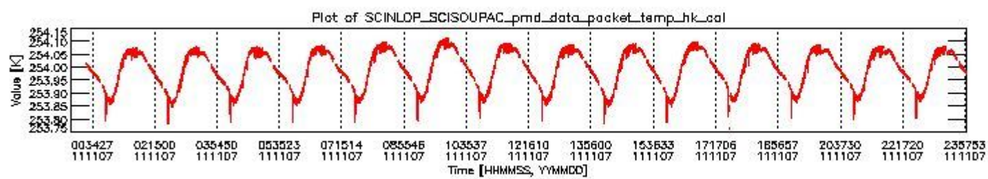
sciamachy_daily_report_level0_KSPT_L0_4504_N_20111107_3.PNG
