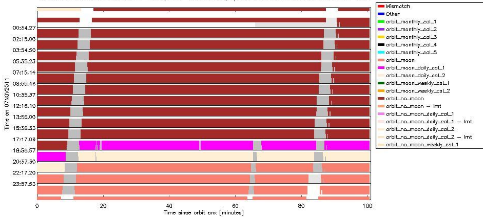
sciamachy_daily_report_level0_KSPT_L0_4504_N_20111107_6.PNG
