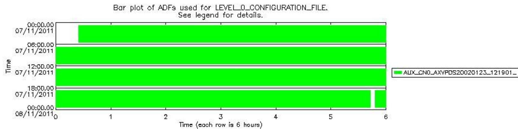
sciamachy_daily_report_level0_KSPT_L0_4504_N_20111107_7.PNG
