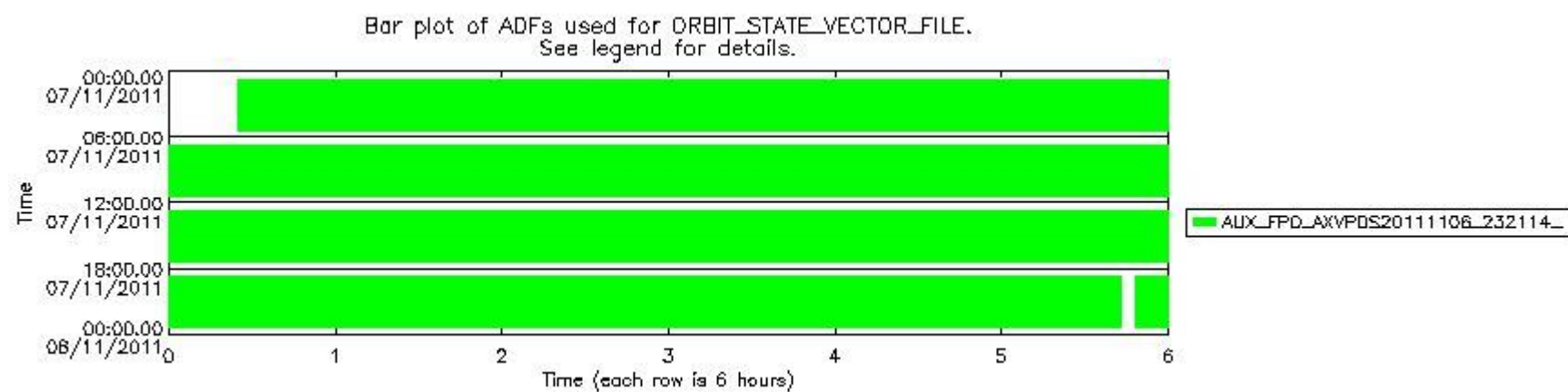
sciamachy_daily_report_level0_KSPT_L0_4504_N_20111107_8.PNG
