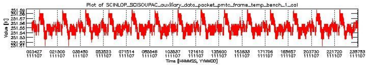
sciamachy_daily_report_level0_KSPT_L0_4504_N_20111107_0.PNG
