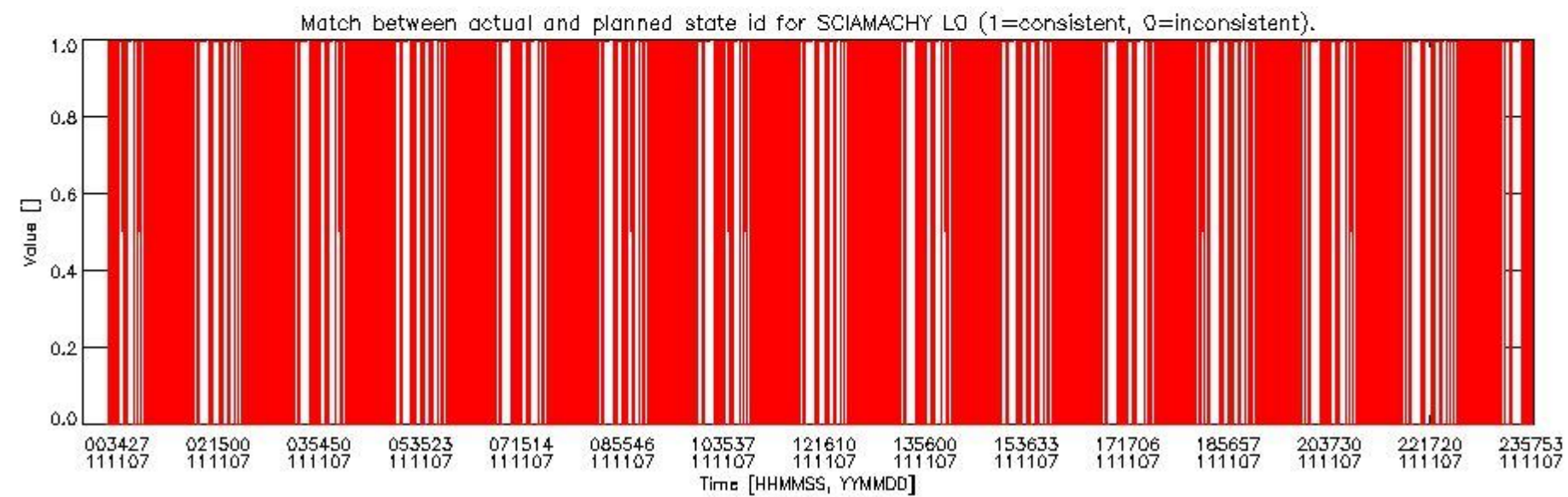
sciamachy_daily_report_level0_KSPT_L0_4504_N_20111107_5.PNG
