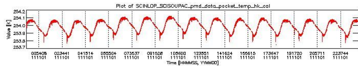
sciamachy_daily_report_level0_KSPT_L0_4504_N_20111101_3.PNG
