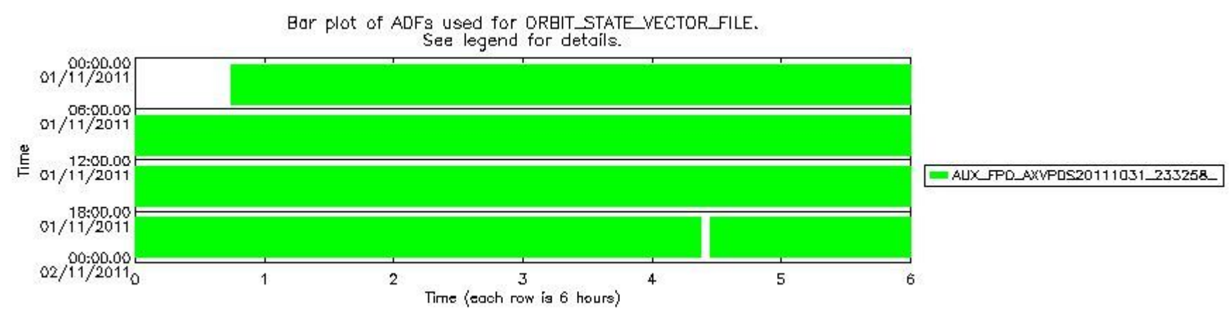
sciamachy_daily_report_level0_KSPT_L0_4504_N_20111101_8.PNG
