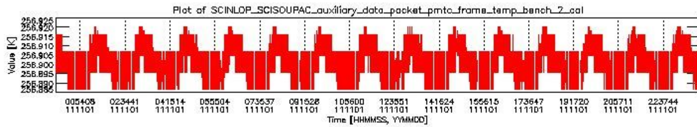
sciamachy_daily_report_level0_KSPT_L0_4504_N_20111101_1.PNG
