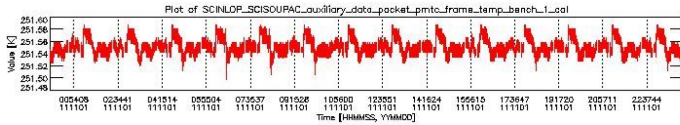
sciamachy_daily_report_level0_KSPT_L0_4504_N_20111101_0.PNG
