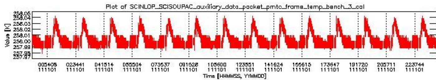
sciamachy_daily_report_level0_KSPT_L0_4504_N_20111101_2.PNG
