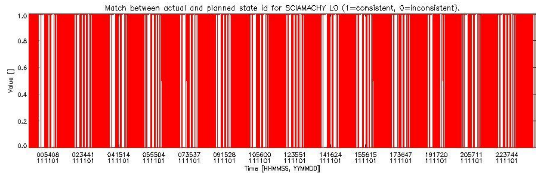
sciamachy_daily_report_level0_KSPT_L0_4504_N_20111101_5.PNG
