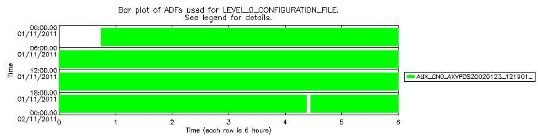
sciamachy_daily_report_level0_KSPT_L0_4504_N_20111101_7.PNG
