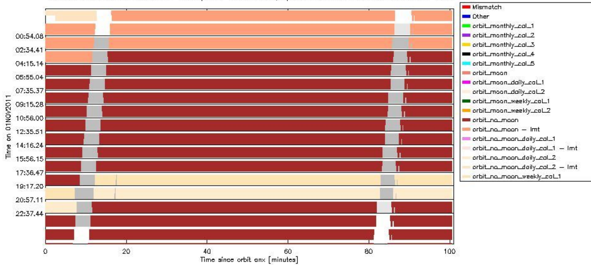
sciamachy_daily_report_level0_KSPT_L0_4504_N_20111101_6.PNG
