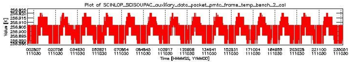
sciamachy_daily_report_level0_KSPT_L0_4504_N_20111030_1.PNG
