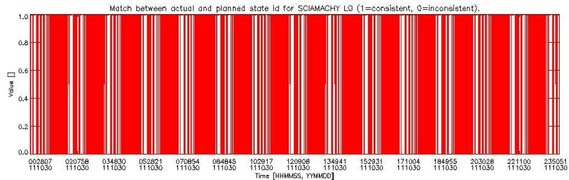
sciamachy_daily_report_level0_KSPT_L0_4504_N_20111030_5.PNG
