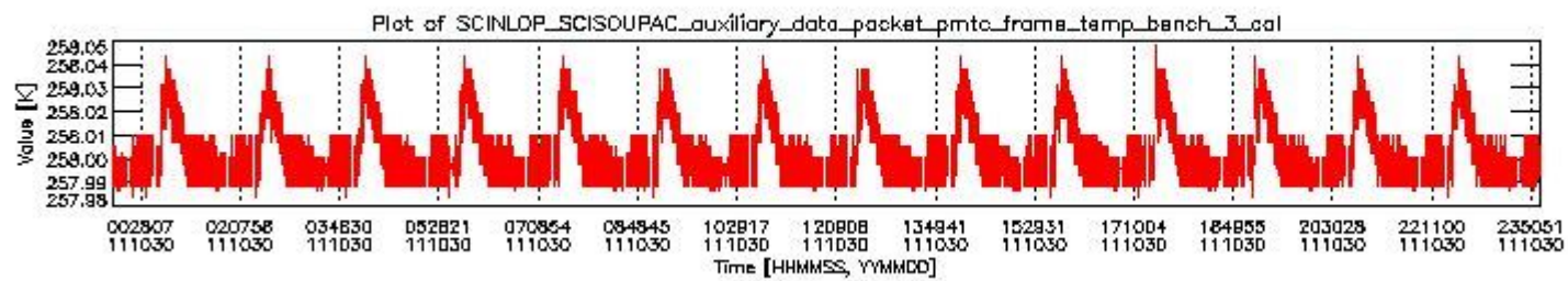
sciamachy_daily_report_level0_KSPT_L0_4504_N_20111030_2.PNG
