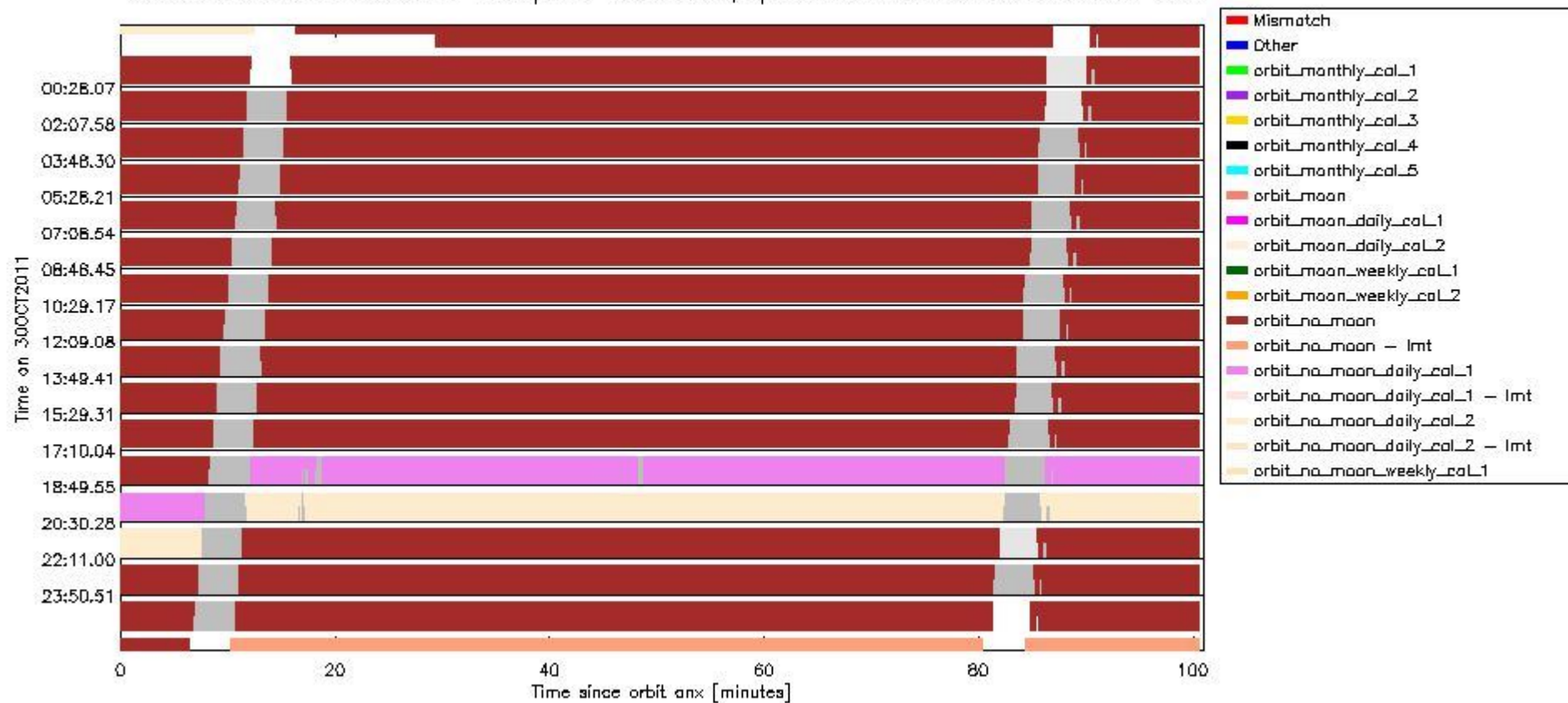
sciamachy_daily_report_level0_KSPT_L0_4504_N_20111030_6.PNG
