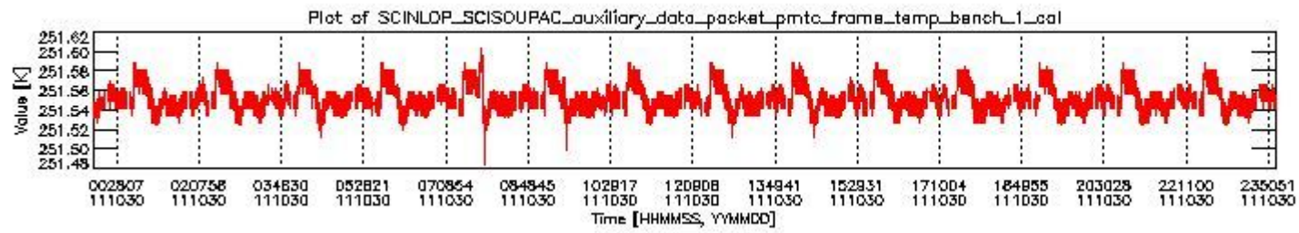
sciamachy_daily_report_level0_KSPT_L0_4504_N_20111030_0.PNG
