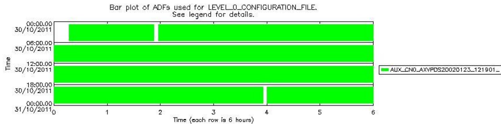
sciamachy_daily_report_level0_KSPT_L0_4504_N_20111030_7.PNG
