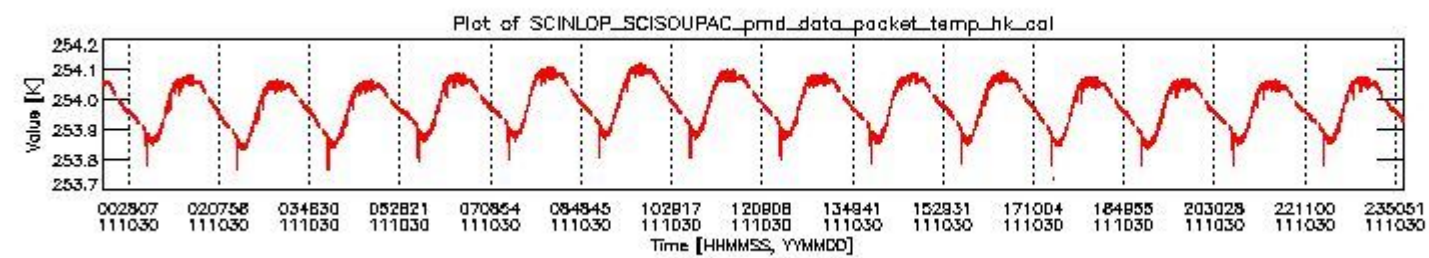
sciamachy_daily_report_level0_KSPT_L0_4504_N_20111030_3.PNG
