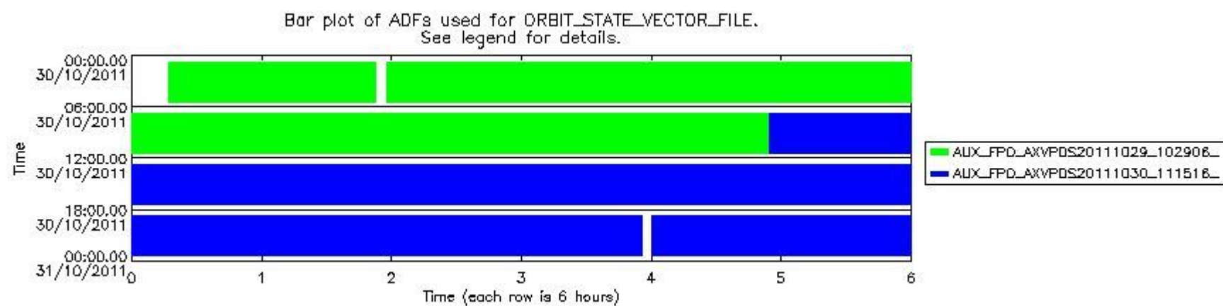
sciamachy_daily_report_level0_KSPT_L0_4504_N_20111030_8.PNG
