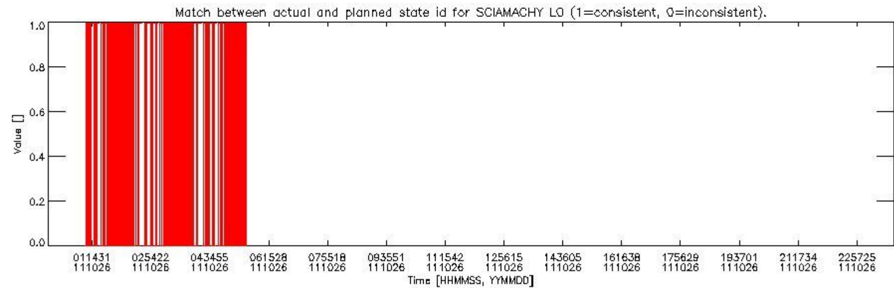
sciamachy_daily_report_level0_KSPT_L0_4504_N_20111026_5.PNG
