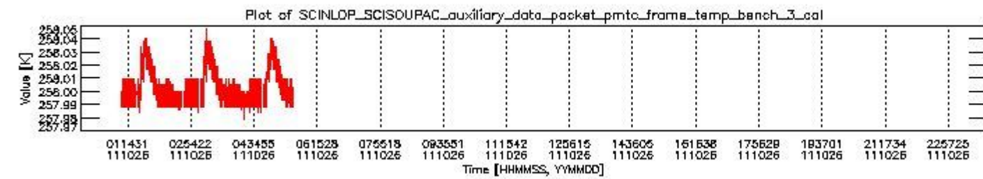
sciamachy_daily_report_level0_KSPT_L0_4504_N_20111026_2.PNG
