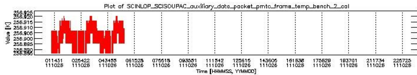
sciamachy_daily_report_level0_KSPT_L0_4504_N_20111026_1.PNG
