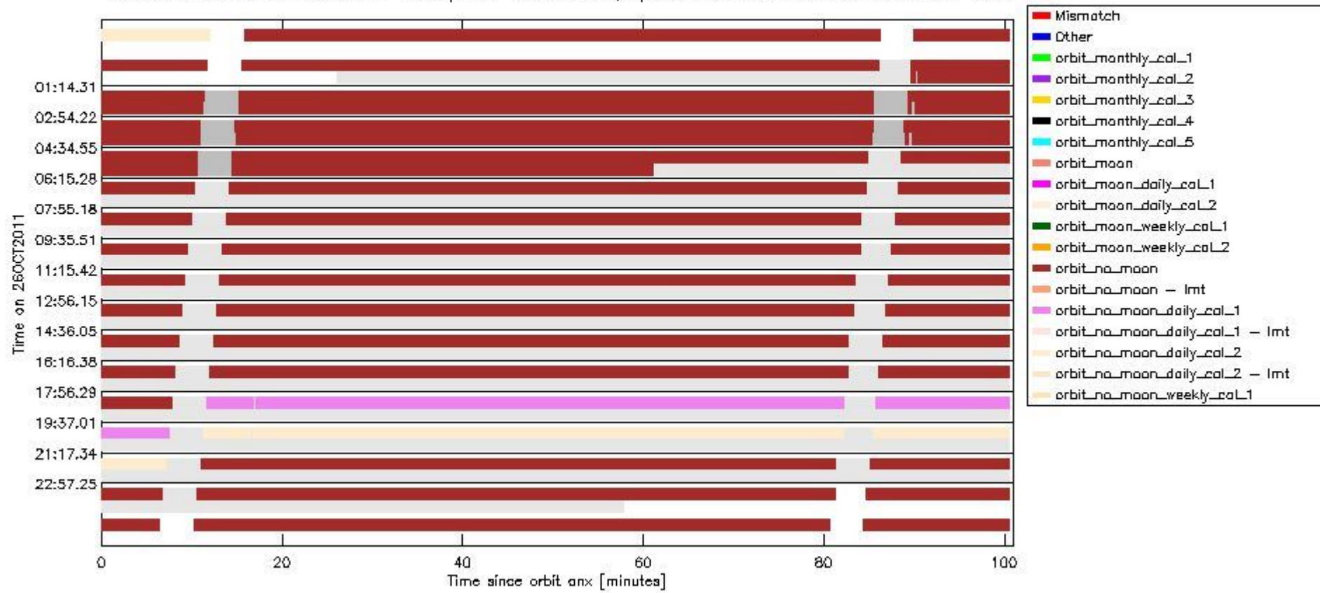
sciamachy_daily_report_level0_KSPT_L0_4504_N_20111026_6.PNG
