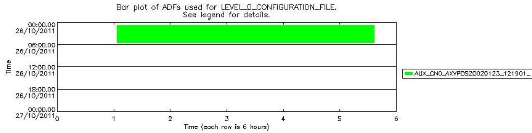
sciamachy_daily_report_level0_KSPT_L0_4504_N_20111026_7.PNG
