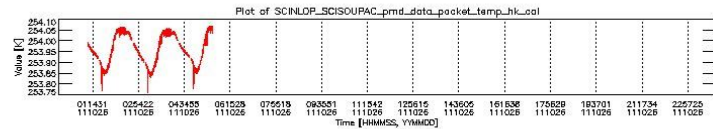
sciamachy_daily_report_level0_KSPT_L0_4504_N_20111026_3.PNG
