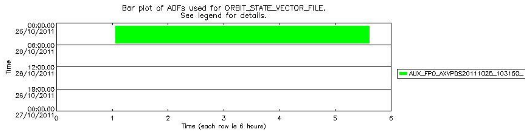
sciamachy_daily_report_level0_KSPT_L0_4504_N_20111026_8.PNG
