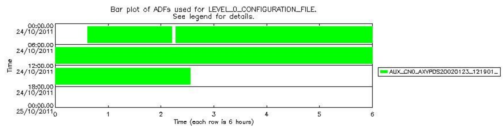
sciamachy_daily_report_level0_KSPT_L0_4504_N_20111024_7.PNG
