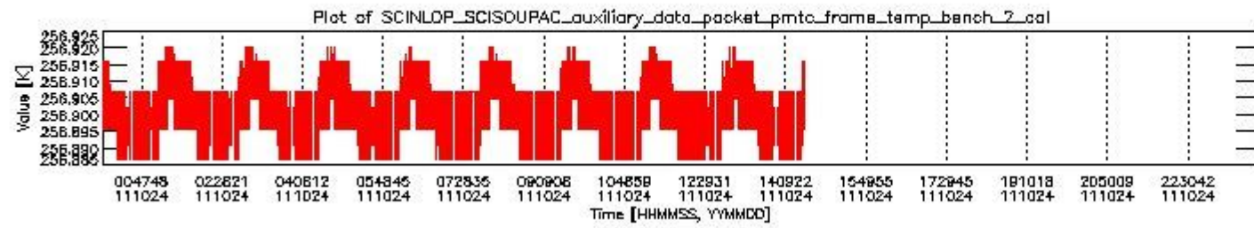
sciamachy_daily_report_level0_KSPT_L0_4504_N_20111024_1.PNG
