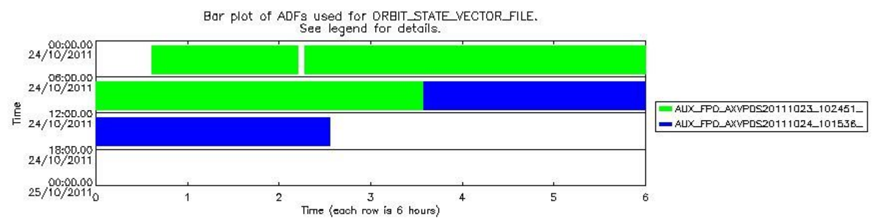
sciamachy_daily_report_level0_KSPT_L0_4504_N_20111024_8.PNG
