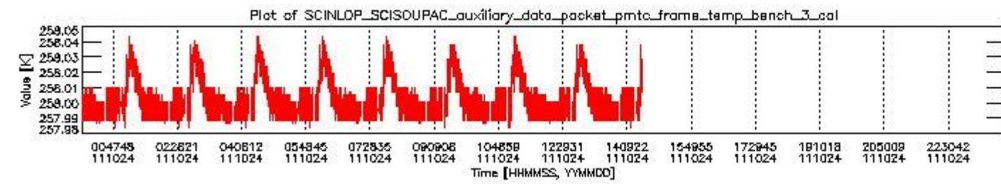
sciamachy_daily_report_level0_KSPT_L0_4504_N_20111024_2.PNG
