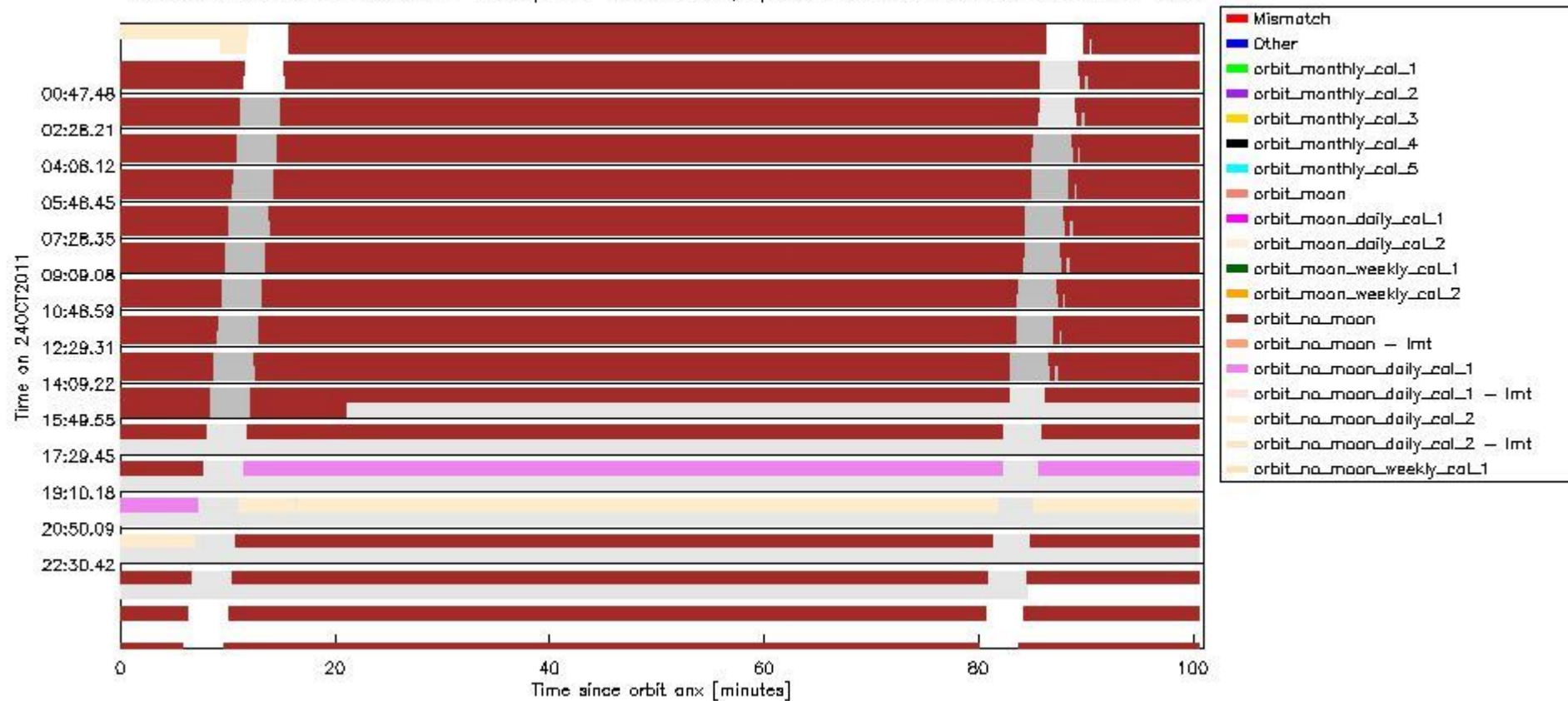
sciamachy_daily_report_level0_KSPT_L0_4504_N_20111024_6.PNG
