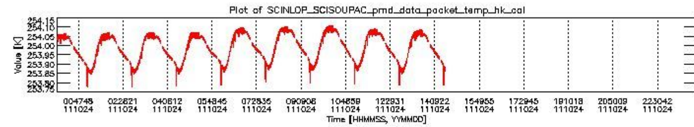
sciamachy_daily_report_level0_KSPT_L0_4504_N_20111024_3.PNG
