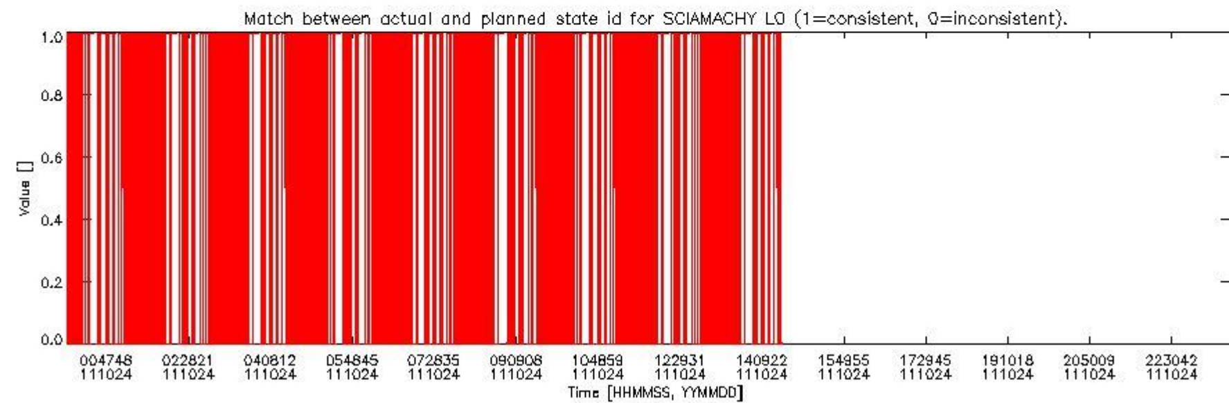
sciamachy_daily_report_level0_KSPT_L0_4504_N_20111024_5.PNG
