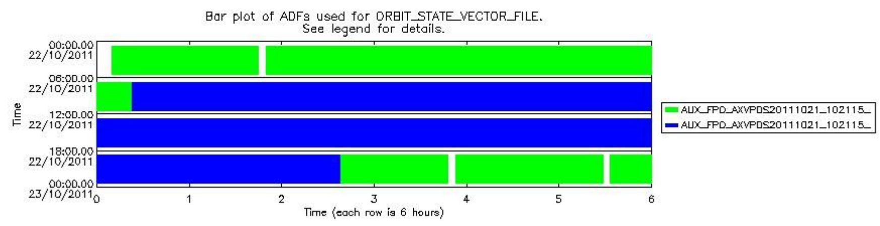
sciamachy_daily_report_level0_KSPT_L0_4504_N_20111022_8.PNG
