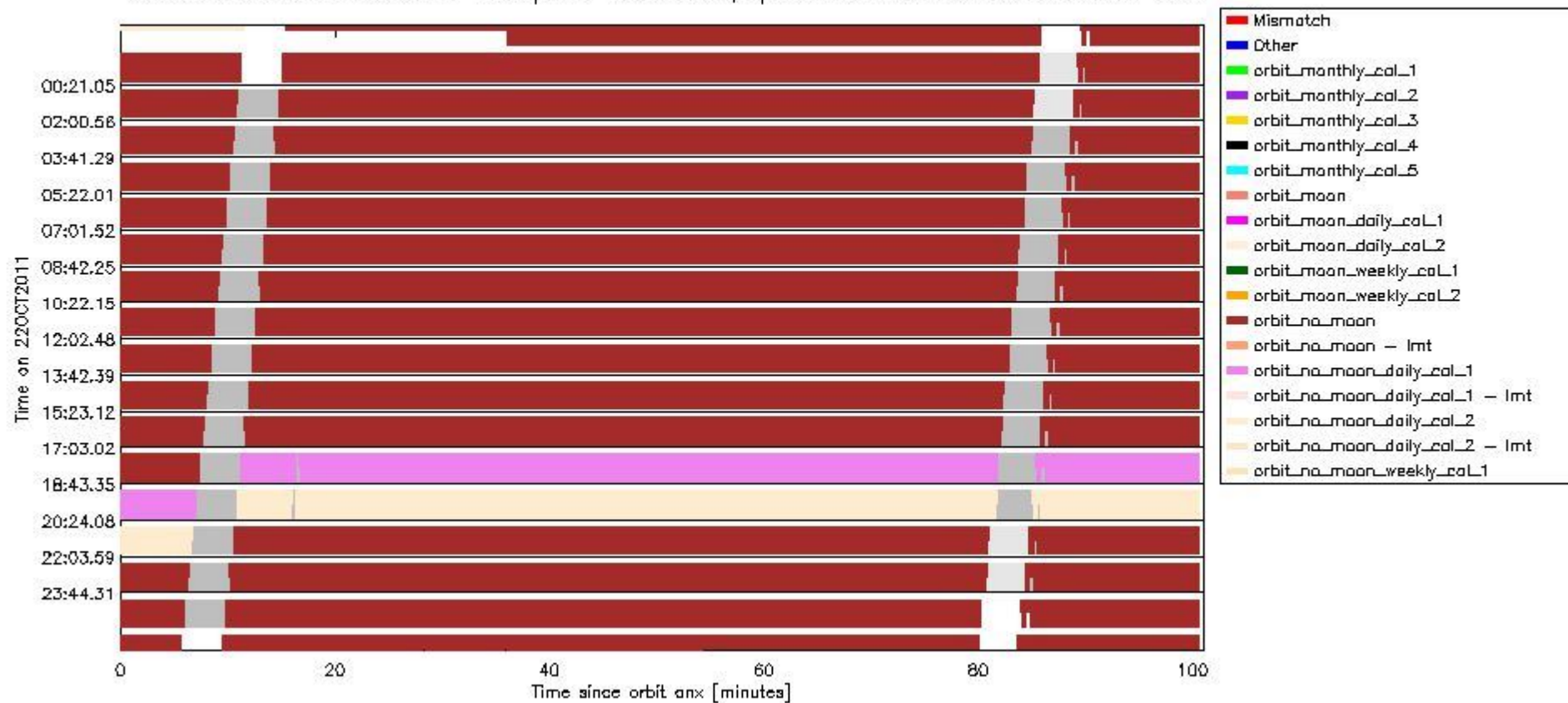
sciamachy_daily_report_level0_KSPT_L0_4504_N_20111022_6.PNG
