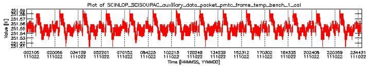
sciamachy_daily_report_level0_KSPT_L0_4504_N_2011022_0.PNG
