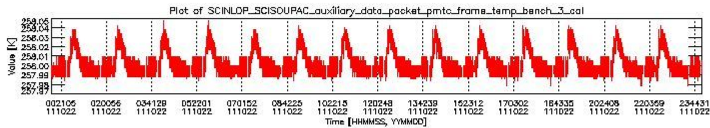
sciamachy_daily_report_level0_KSPT_L0_4504_N_2011022_2.PNG
