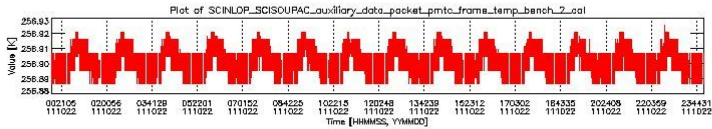
sciamachy_daily_report_level0_KSPT_L0_4504_N_2011022_1.PNG
