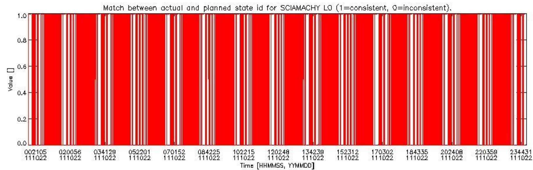
sciamachy_daily_report_level0_KSPT_L0_4504_N_20111022_5.PNG
