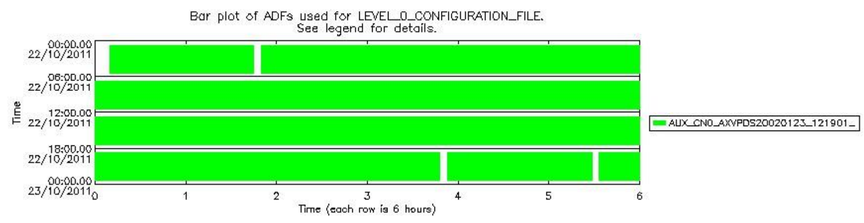
sciamachy_daily_report_level0_KSPT_L0_4504_N_20111022_7.PNG
