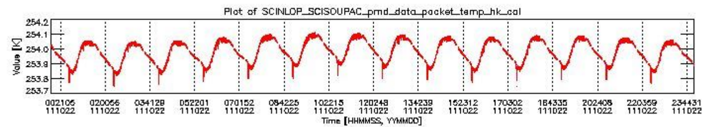
sciamachy_daily_report_level0_KSPT_L0_4504_N_2011022_3.PNG
