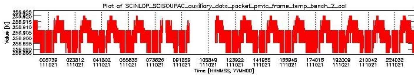
sciamachy_daily_report_level0_KSPT_L0_4504_N_20111021_1.PNG
