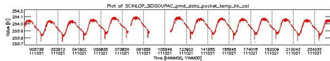
sciamachy_daily_report_level0_KSPT_L0_4504_N_20111021_3.PNG
