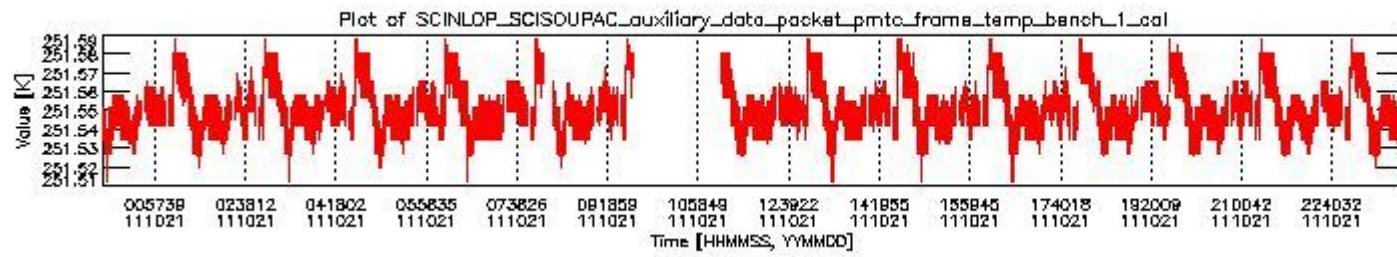
sciamachy_daily_report_level0_KSPT_L0_4504_N_20111021_0.PNG
