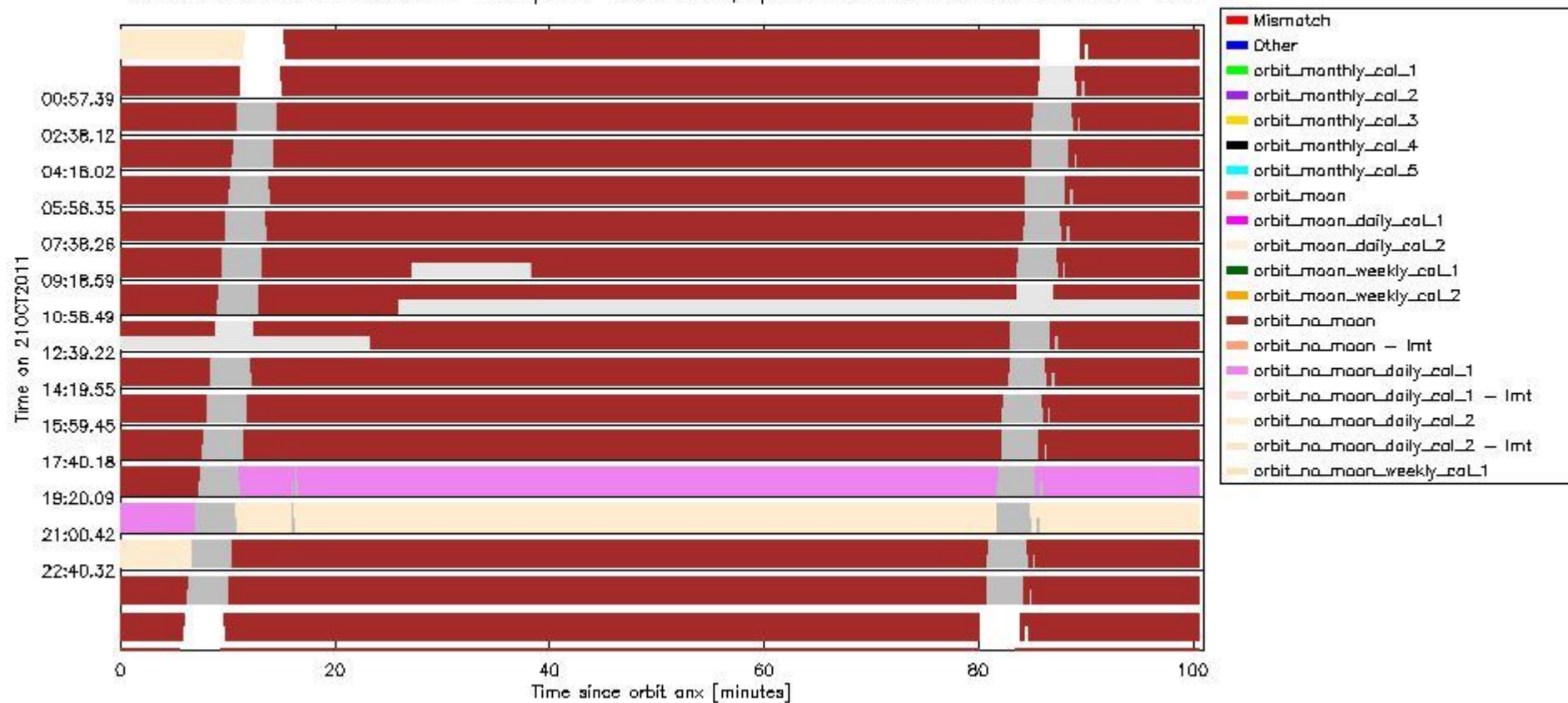
sciamachy_daily_report_level0_KSPT_L0_4504_N_20111021_6.PNG
