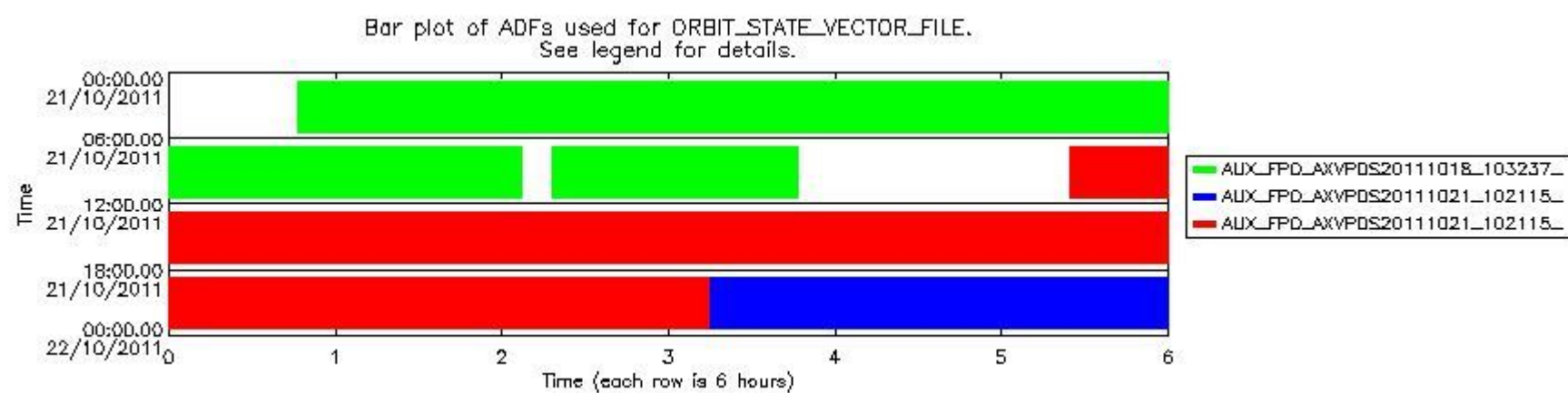
sciamachy_daily_report_level0_KSPT_L0_4504_N_20111021_8.PNG
