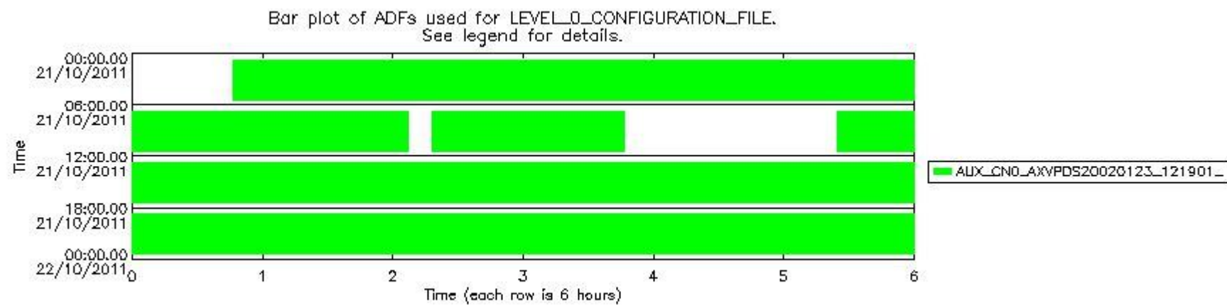
sciamachy_daily_report_level0_KSPT_L0_4504_N_20111021_7.PNG
