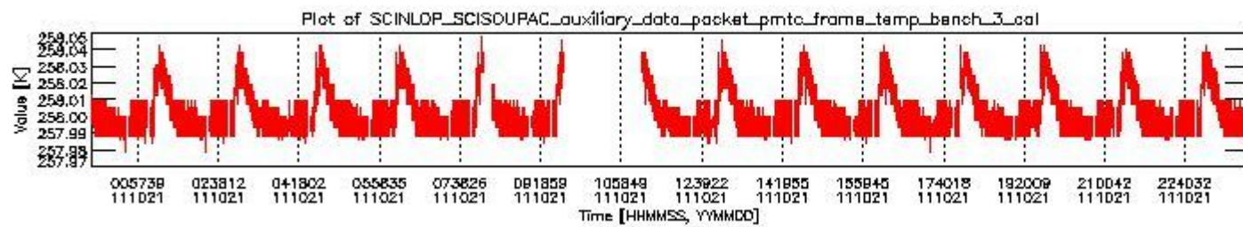
sciamachy_daily_report_level0_KSPT_L0_4504_N_20111021_2.PNG
