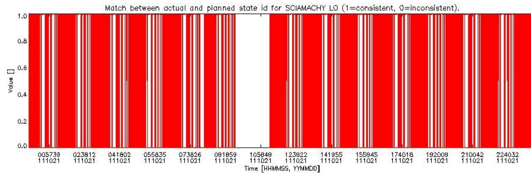
sciamachy_daily_report_level0_KSPT_L0_4504_N_20111021_5.PNG
