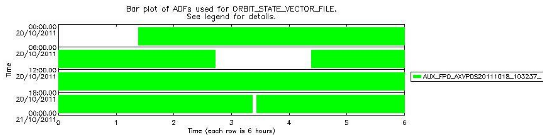
sciamachy_daily_report_level0_KSPT_L0_4504_N_20111020_8.PNG
