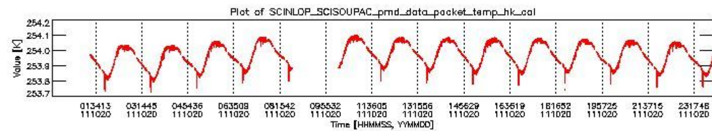
sciamachy_daily_report_level0_KSPT_L0_4504_N_20111020_3.PNG
