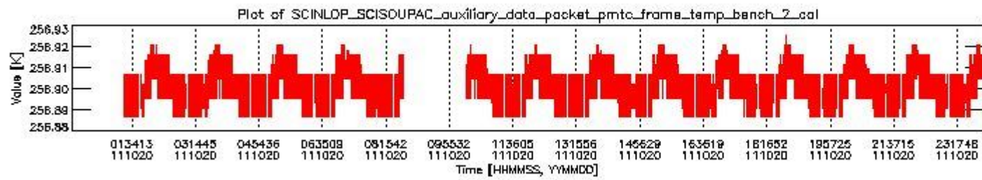
sciamachy_daily_report_level0_KSPT_L0_4504_N_20111020_1.PNG
