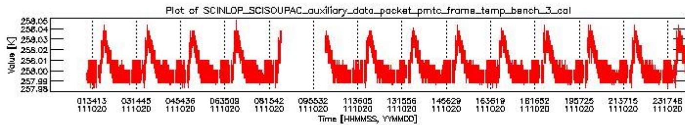
sciamachy_daily_report_level0_KSPT_L0_4504_N_20111020_2.PNG
