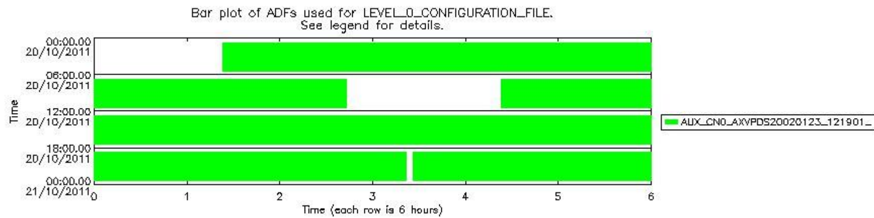
sciamachy_daily_report_level0_KSPT_L0_4504_N_20111020_7.PNG
