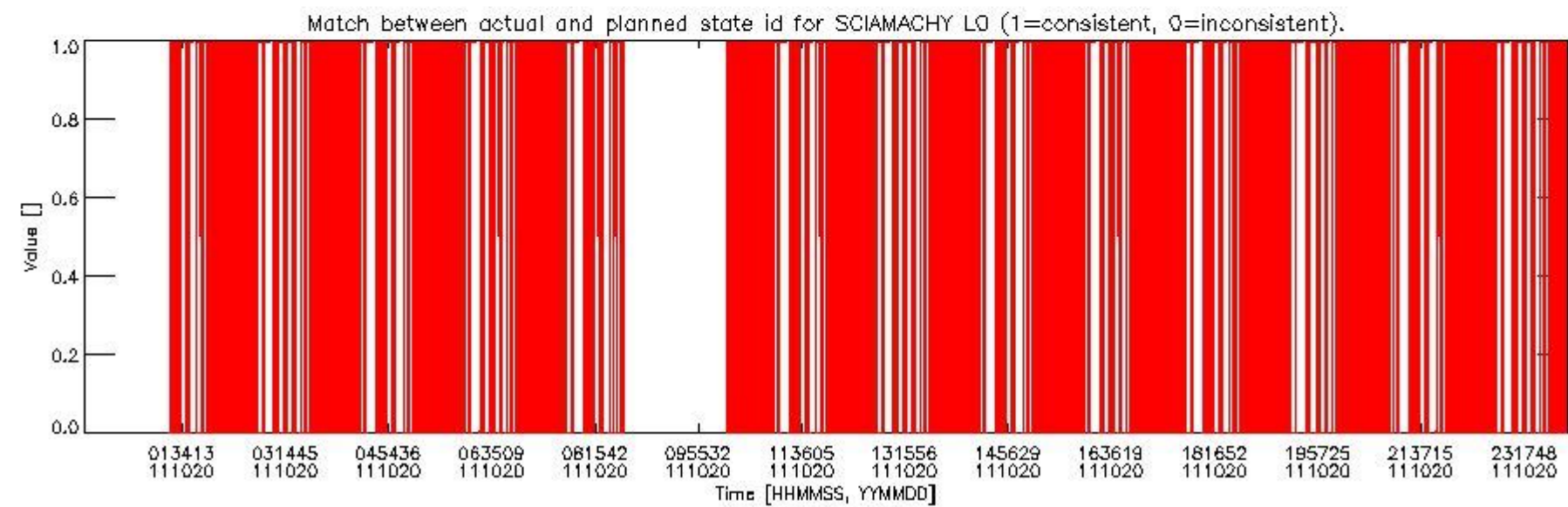
sciamachy_daily_report_level0_KSPT_L0_4504_N_20111020_5.PNG
