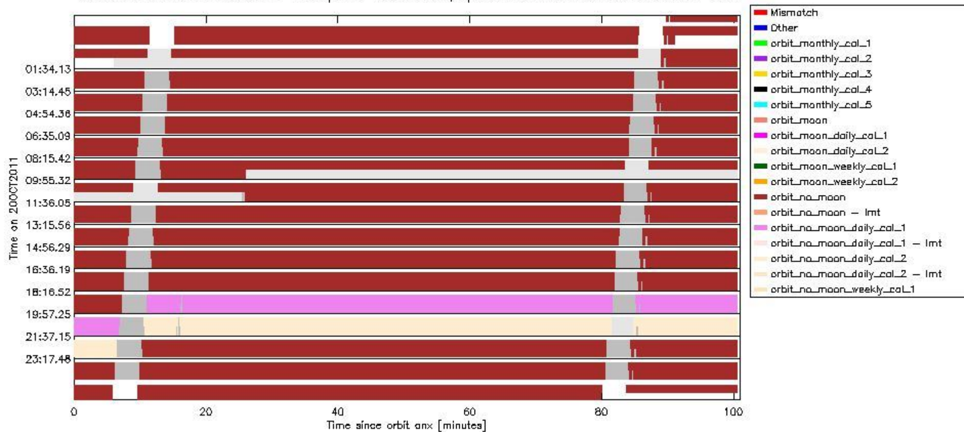
sciamachy_daily_report_level0_KSPT_L0_4504_N_20111020_6.PNG
