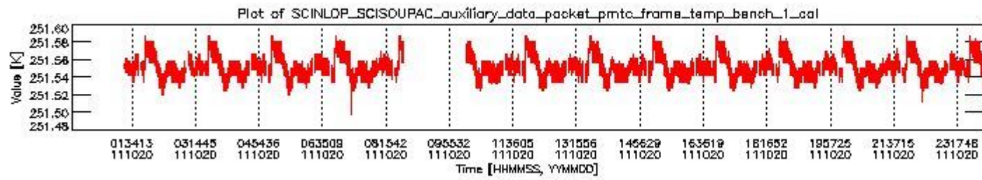
sciamachy_daily_report_level0_KSPT_L0_4504_N_20111020_0.PNG
