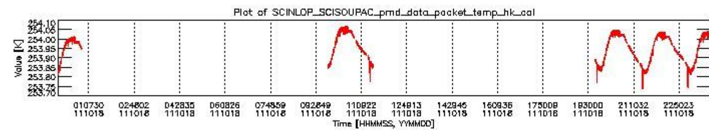
sciamachy_daily_report_level0_KSPT_L0_4504_N_20111018_3.PNG
