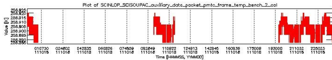
sciamachy_daily_report_level0_KSPT_L0_4504_N_20111018_1.PNG
