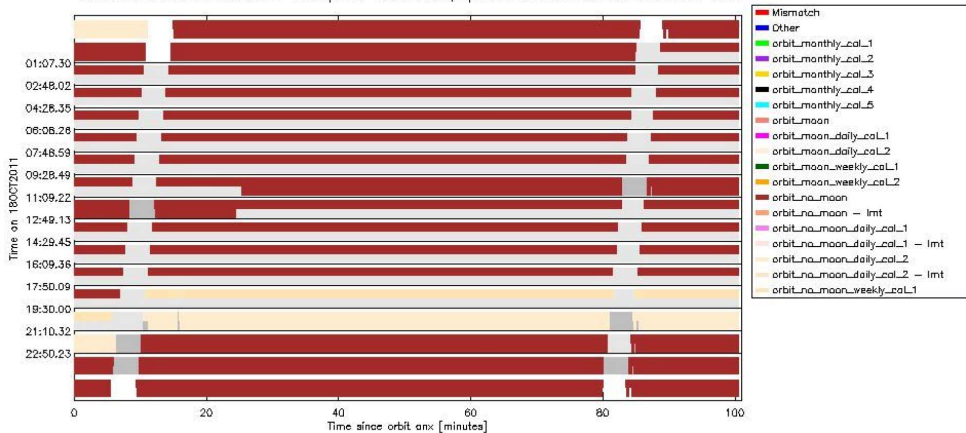
sciamachy_daily_report_level0_KSPT_L0_4504_N_20111018_6.PNG
