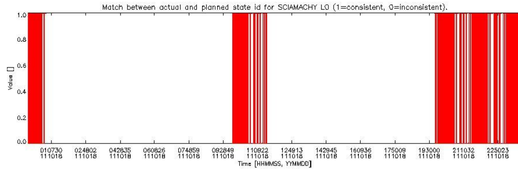
sciamachy_daily_report_level0_KSPT_L0_4504_N_20111018_5.PNG
