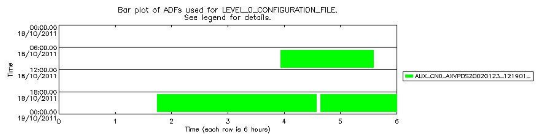
sciamachy_daily_report_level0_KSPT_L0_4504_N_20111018_7.PNG
