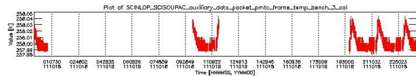
sciamachy_daily_report_level0_KSPT_L0_4504_N_20111018_2.PNG
