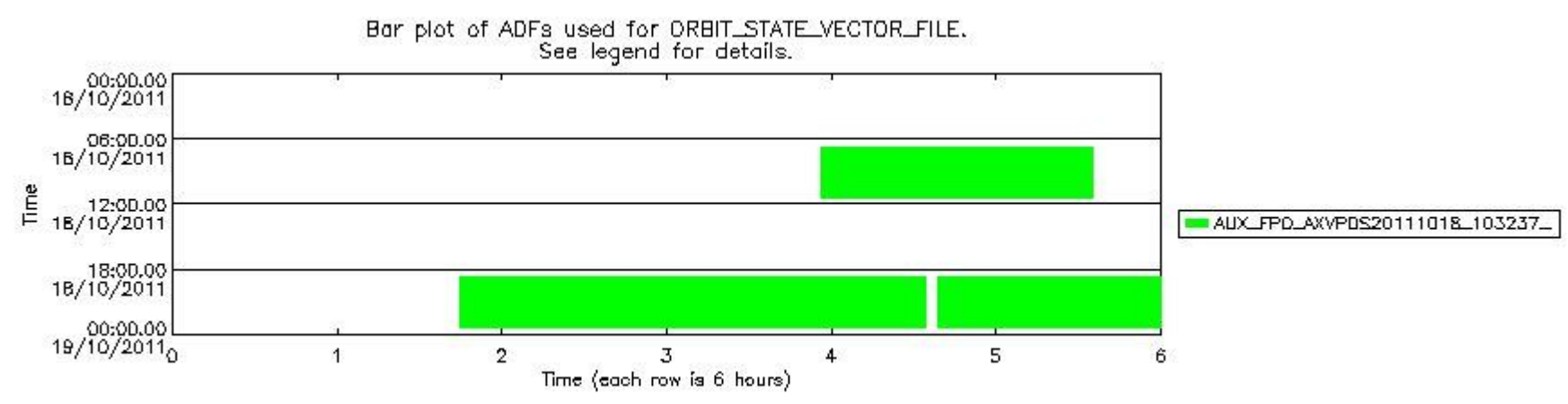
sciamachy_daily_report_level0_KSPT_L0_4504_N_20111018_8.PNG
