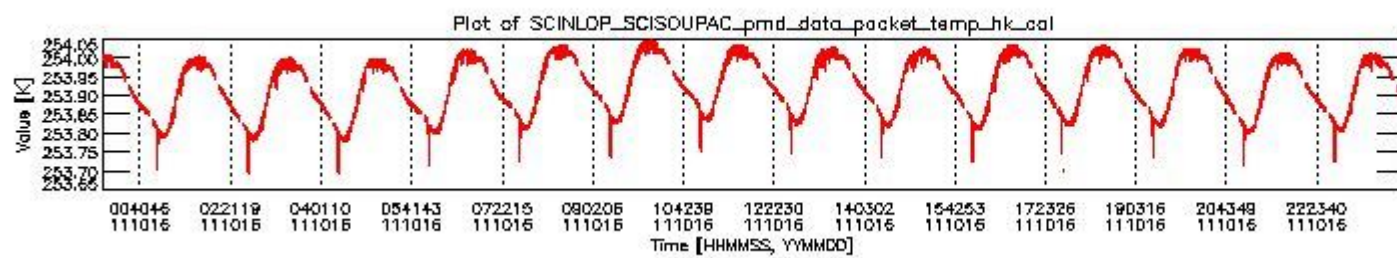
sciamachy_daily_report_level0_KSPT_L0_4504_N_20111016_3.PNG
