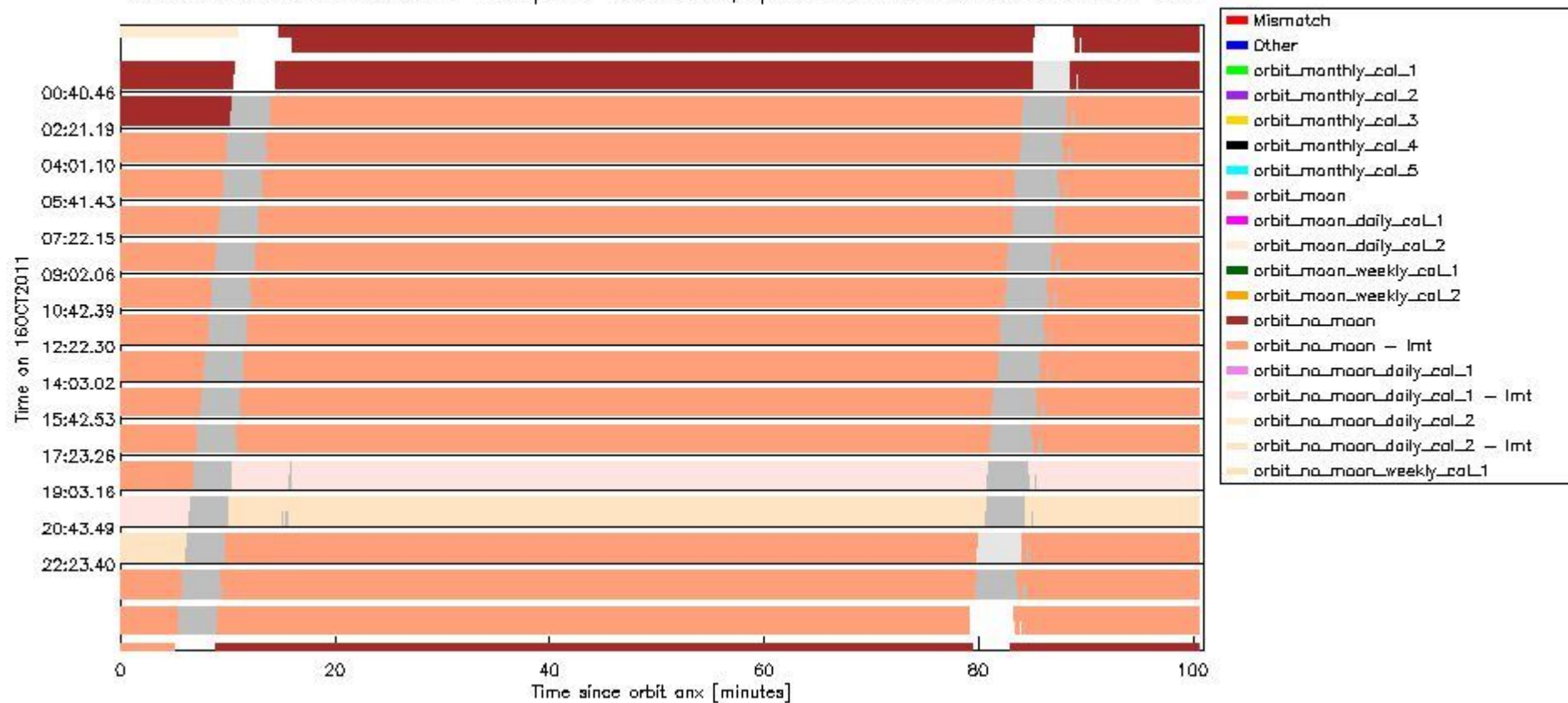
sciamachy_daily_report_level0_KSPT_L0_4504_N_20111016_6.PNG
