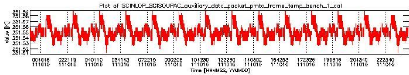
sciamachy_daily_report_level0_KSPT_L0_4504_N_20111016_0.PNG
