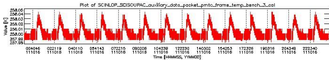
sciamachy_daily_report_level0_KSPT_L0_4504_N_20111016_2.PNG
