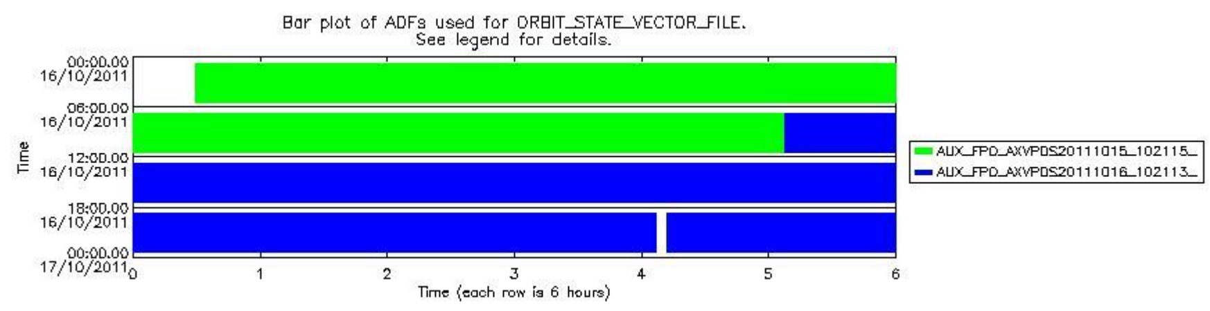
sciamachy_daily_report_level0_KSPT_L0_4504_N_20111016_8.PNG
