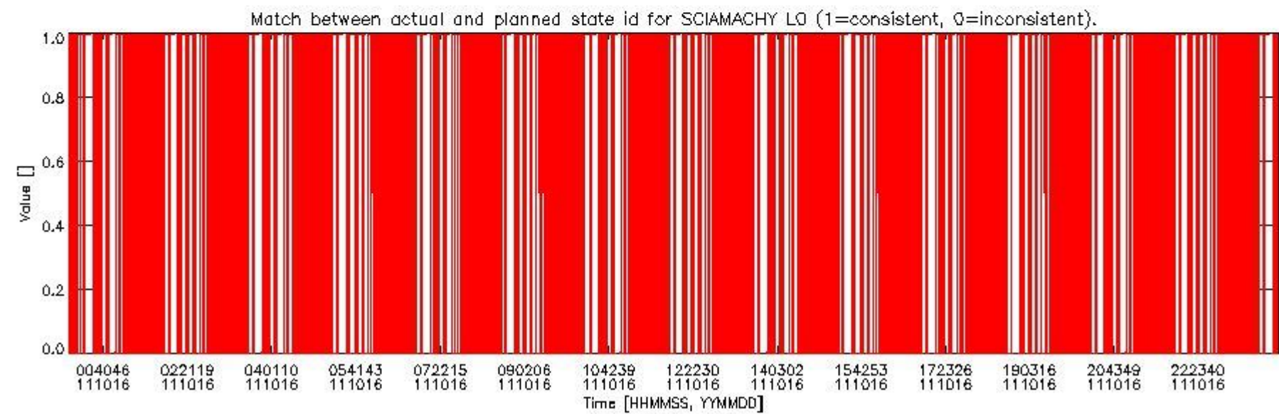
sciamachy_daily_report_level0_KSPT_L0_4504_N_20111016_5.PNG
