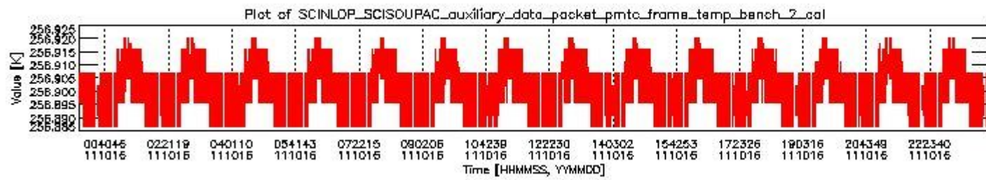
sciamachy_daily_report_level0_KSPT_L0_4504_N_20111016_1.PNG
