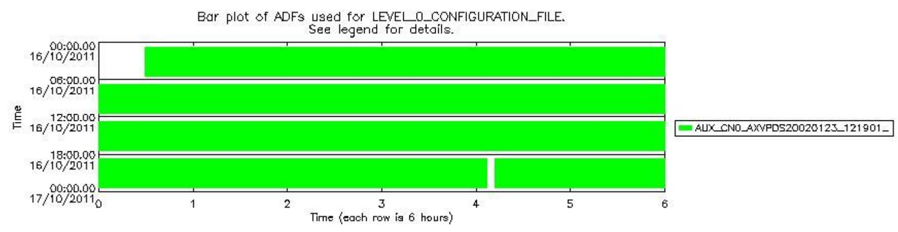
sciamachy_daily_report_level0_KSPT_L0_4504_N_20111016_7.PNG
