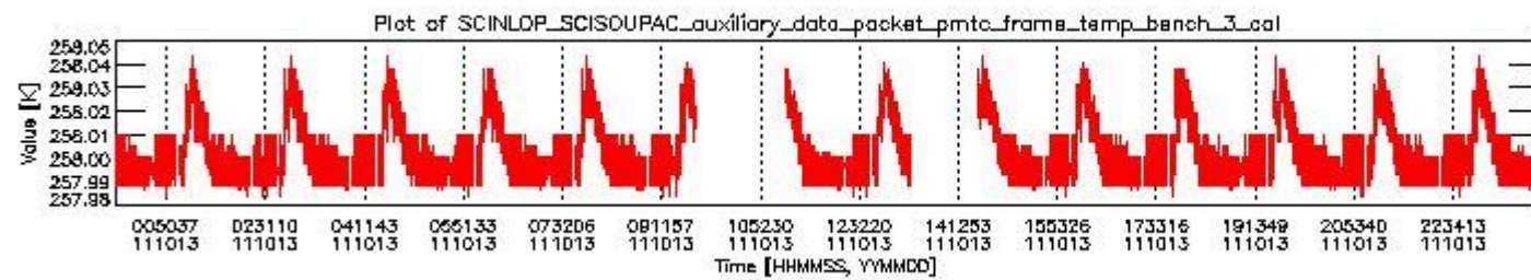
sciamachy_daily_report_level0_KSPT_L0_4504_N_20111013_2.PNG
