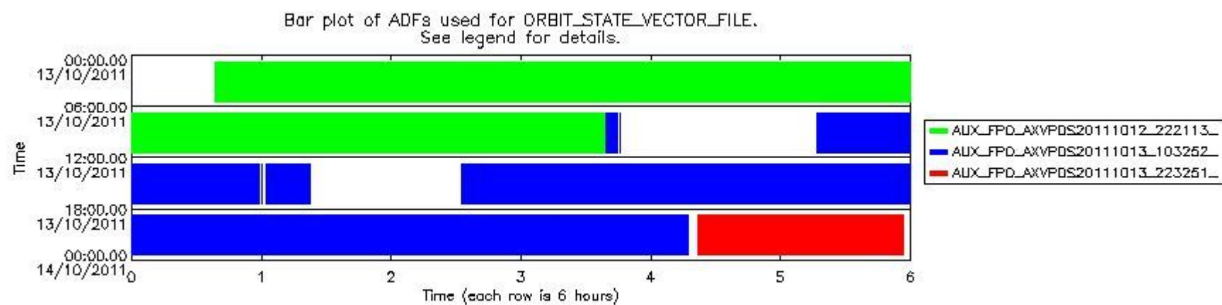
sciamachy_daily_report_level0_KSPT_L0_4504_N_20111013_8.PNG
