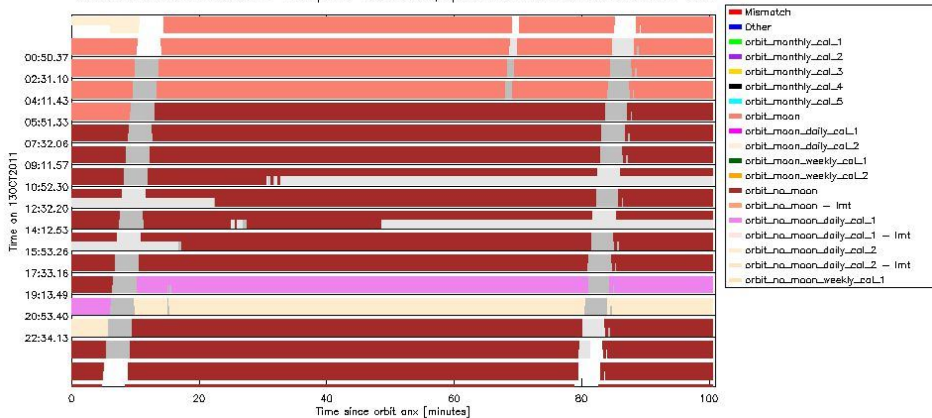
sciamachy_daily_report_level0_KSPT_L0_4504_N_20111013_6.PNG
