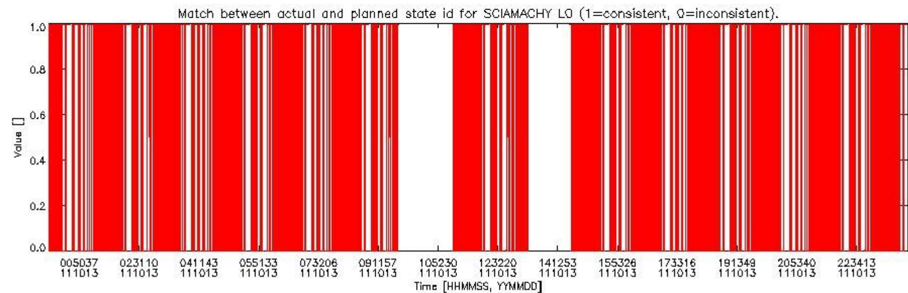
sciamachy_daily_report_level0_KSPT_L0_4504_N_20111013_5.PNG
