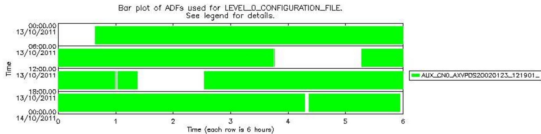
sciamachy_daily_report_level0_KSPT_L0_4504_N_20111013_7.PNG
