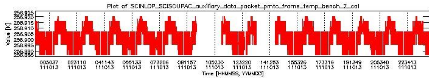
sciamachy_daily_report_level0_KSPT_L0_4504_N_20111013_1.PNG
