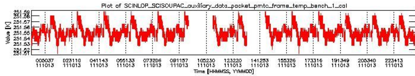
sciamachy_daily_report_level0_KSPT_L0_4504_N_20111013_0.PNG
