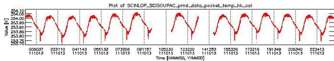
sciamachy_daily_report_level0_KSPT_L0_4504_N_20111013_3.PNG
