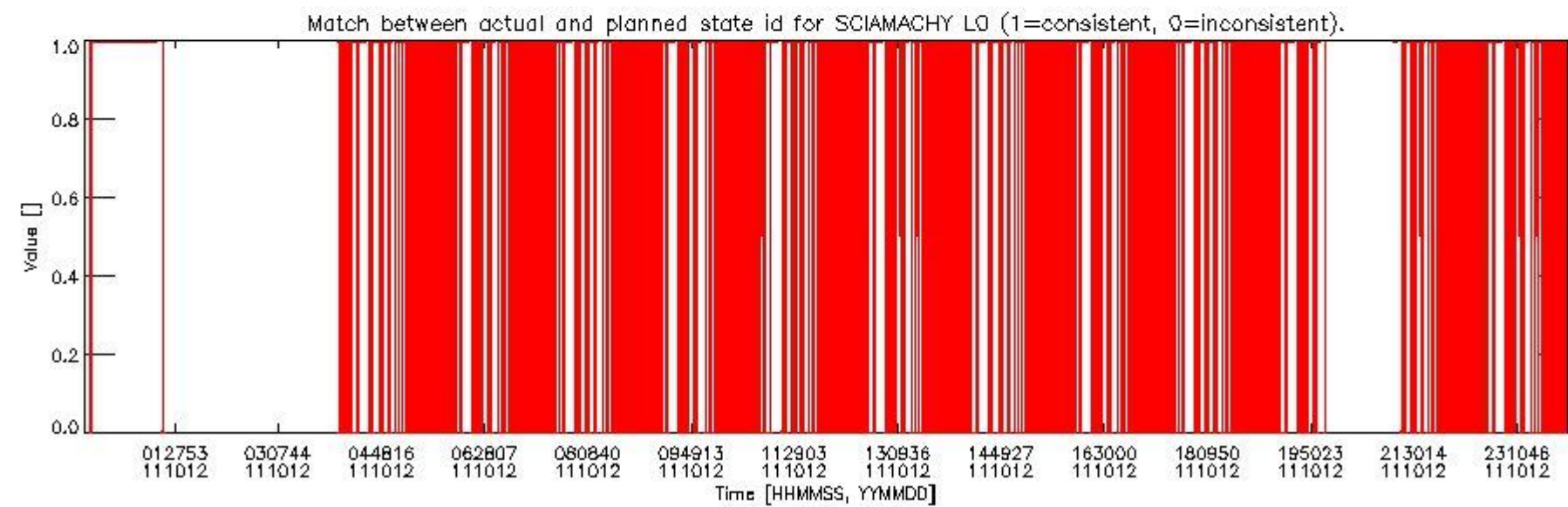
sciamachy_daily_report_level0_KSPT_L0_4504_N_20111012_5.PNG
