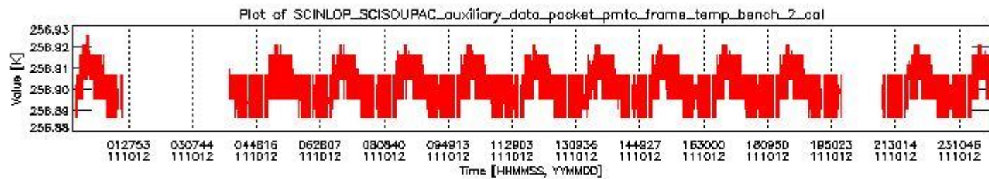
sciamachy_daily_report_level0_KSPT_L0_4504_N_20111012_1.PNG
