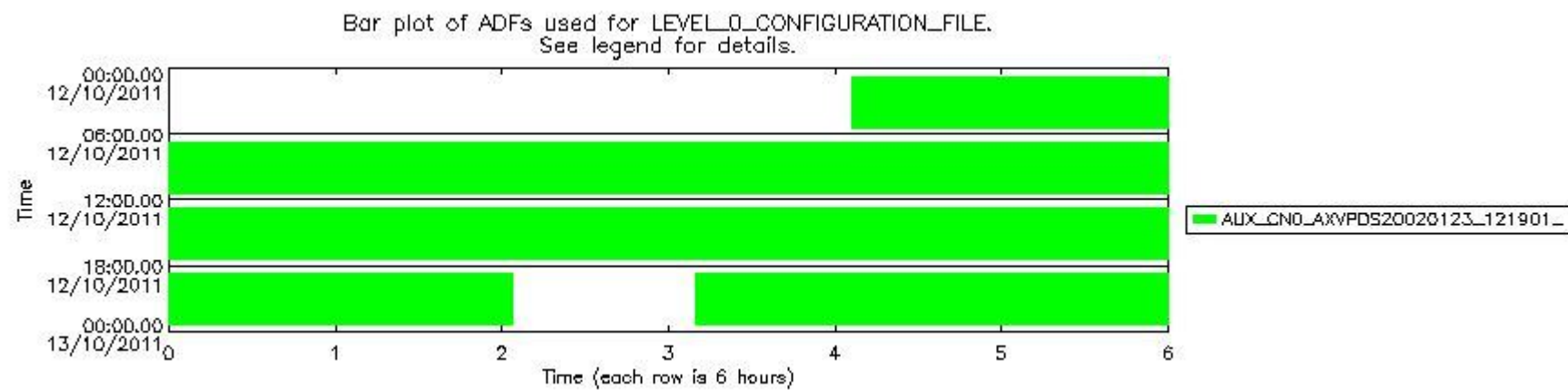
sciamachy_daily_report_level0_KSPT_L0_4504_N_20111012_7.PNG
