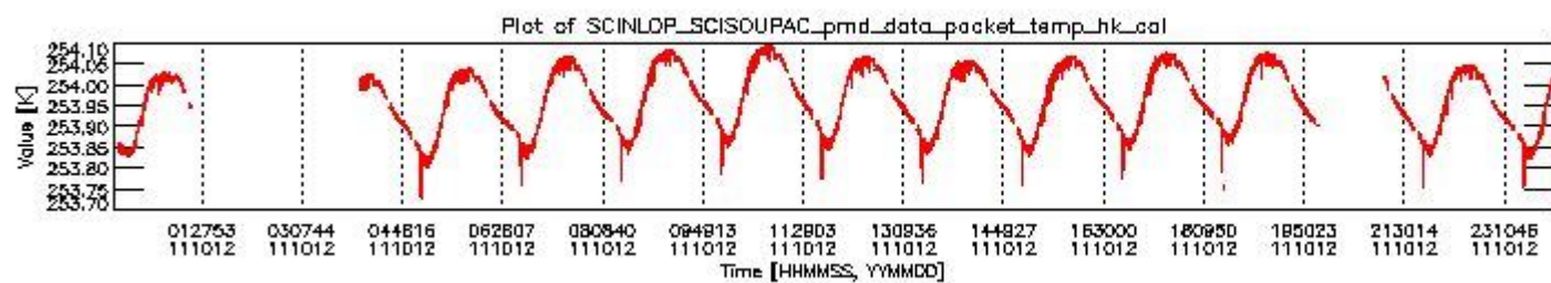
sciamachy_daily_report_level0_KSPT_L0_4504_N_20111012_3.PNG
