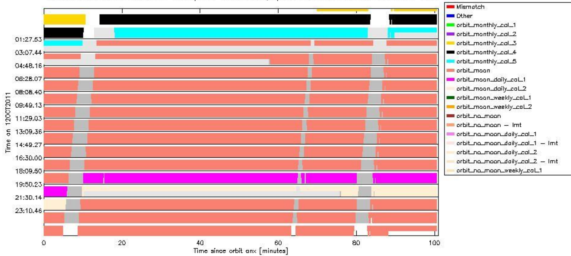
sciamachy_daily_report_level0_KSPT_L0_4504_N_20111012_6.PNG
