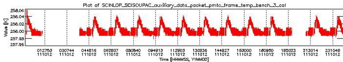
sciamachy_daily_report_level0_KSPT_L0_4504_N_20111012_2.PNG
