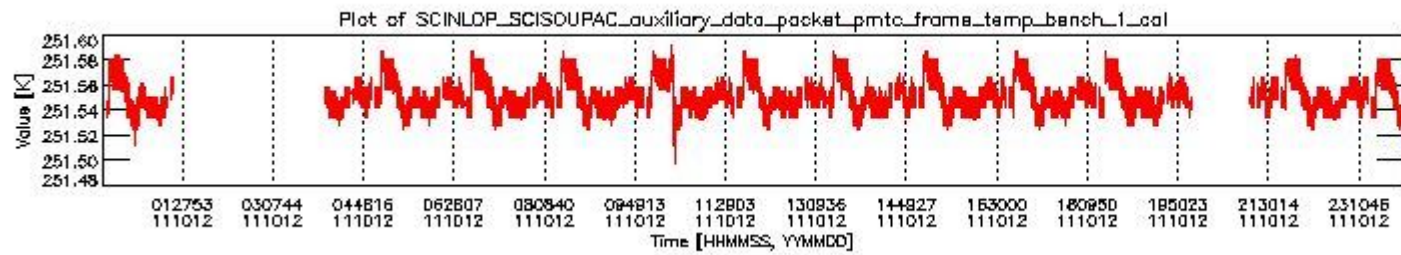
sciamachy_daily_report_level0_KSPT_L0_4504_N_20111012_0.PNG
