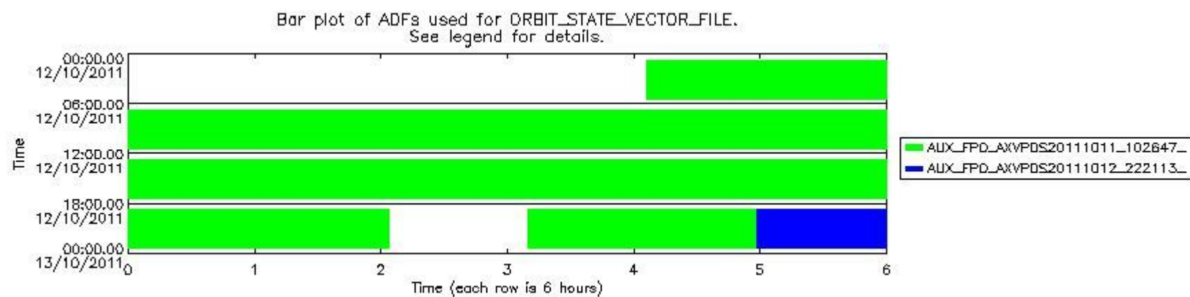
sciamachy_daily_report_level0_KSPT_L0_4504_N_20111012_8.PNG
