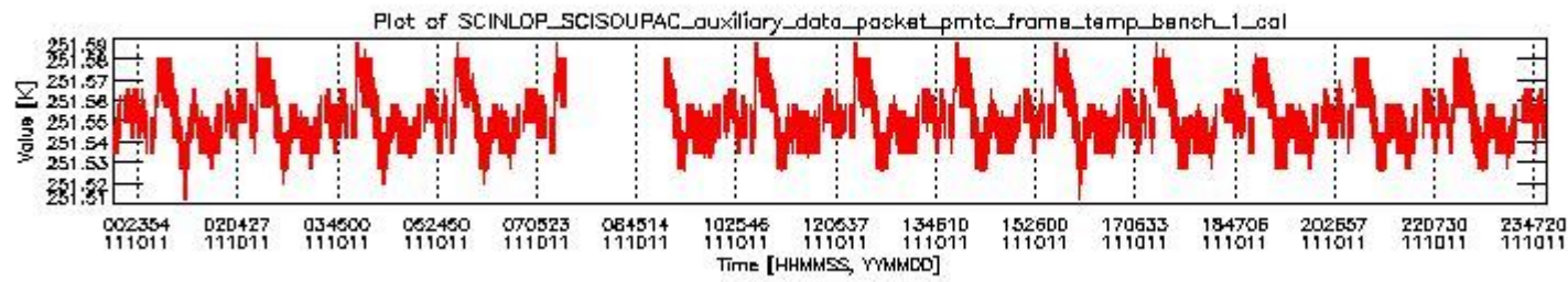
sciamachy_daily_report_level0_KSPT_L0_4504_N_20111011_0.PNG
