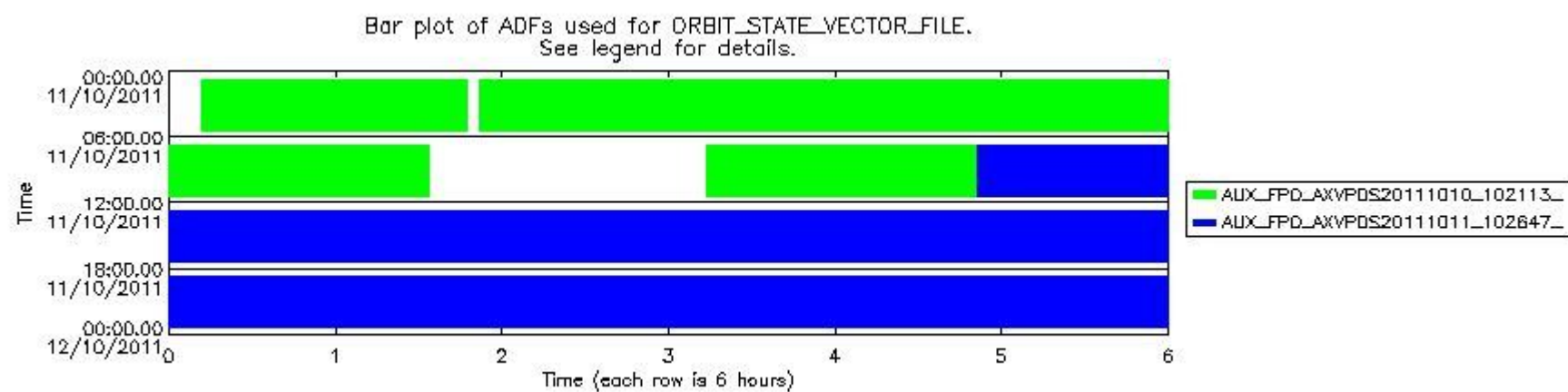
sciamachy_daily_report_level0_KSPT_L0_4504_N_20111011_8.PNG
