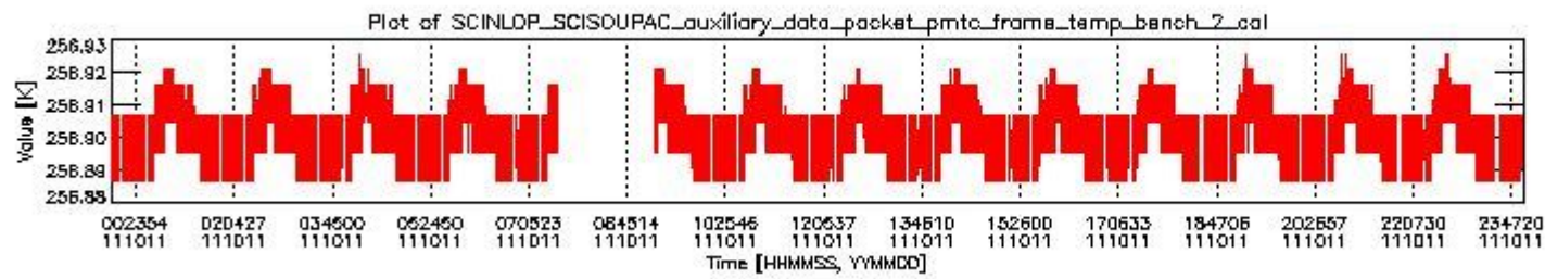
sciamachy_daily_report_level0_KSPT_L0_4504_N_20111011_1.PNG
