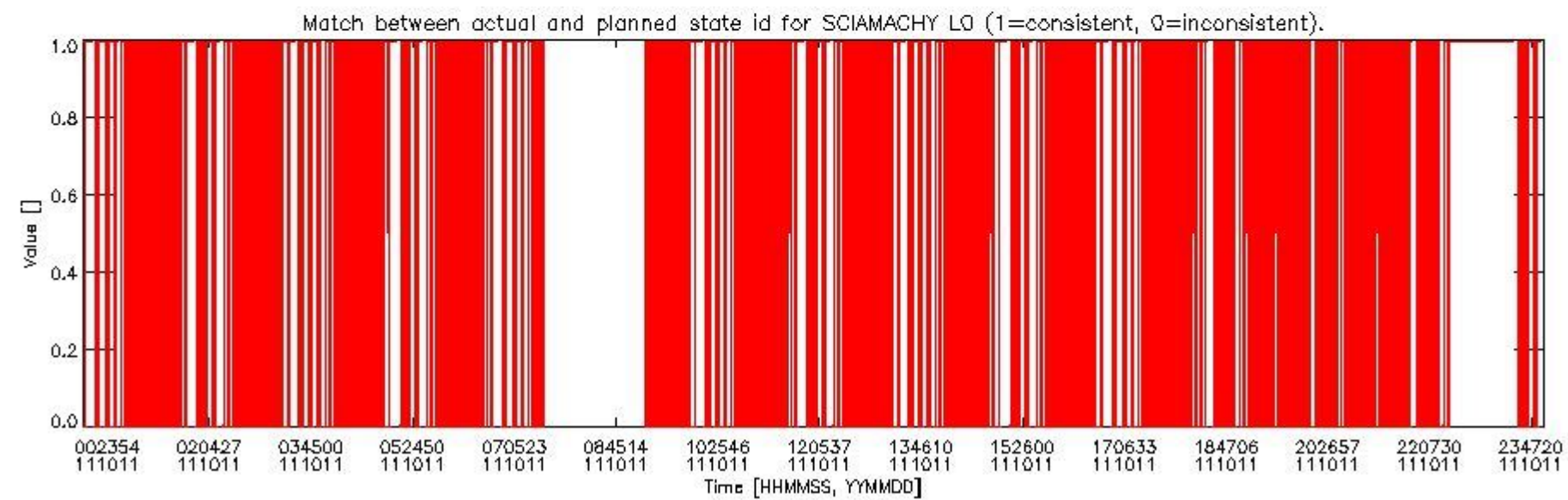
sciamachy_daily_report_level0_KSPT_L0_4504_N_20111011_5.PNG
