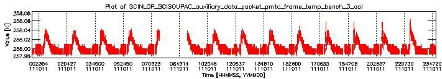
sciamachy_daily_report_level0_KSPT_L0_4504_N_20111011_2.PNG
