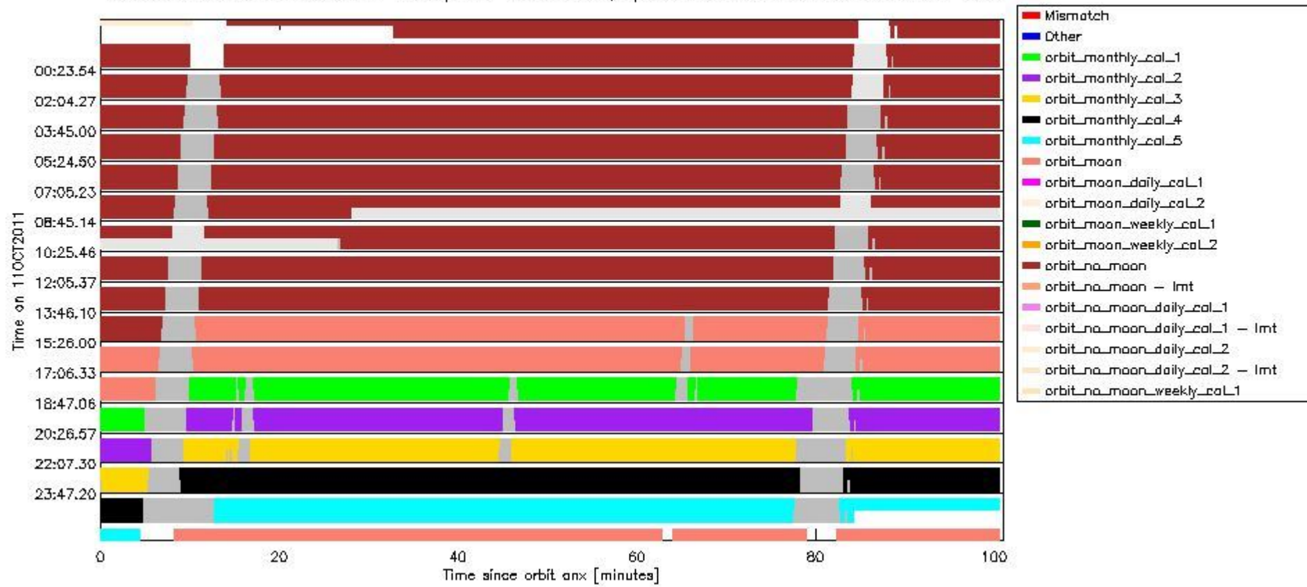
sciamachy_daily_report_level0_KSPT_L0_4504_N_20111011_6.PNG
