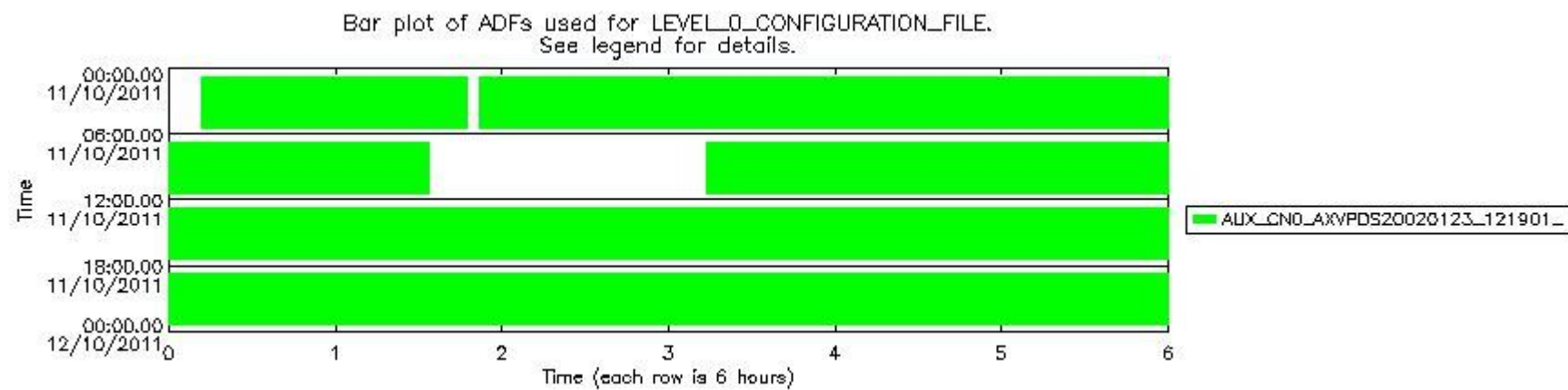
sciamachy_daily_report_level0_KSPT_L0_4504_N_20111011_7.PNG
