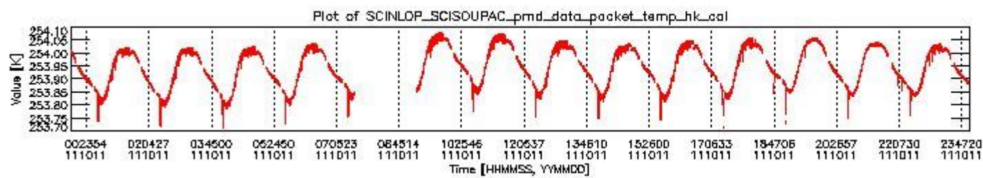
sciamachy_daily_report_level0_KSPT_L0_4504_N_20111011_3.PNG
