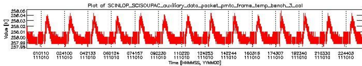
sciamachy_daily_report_level0_KSPT_L0_4504_N_20111010_2.PNG
