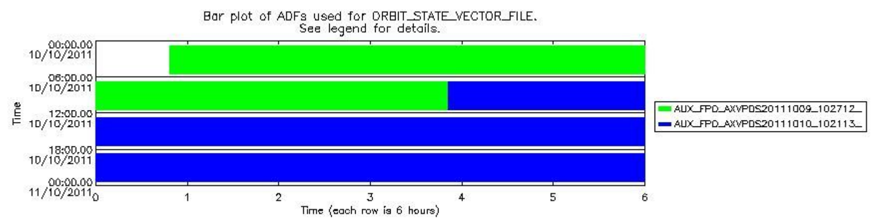
sciamachy_daily_report_level0_KSPT_L0_4504_N_20111010_8.PNG
