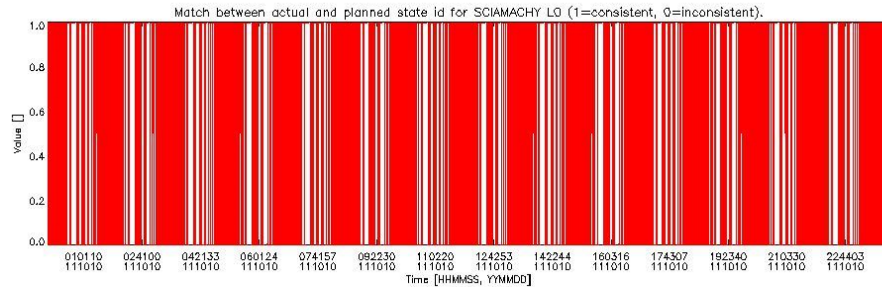
sciamachy_daily_report_level0_KSPT_L0_4504_N_20111010_5.PNG
