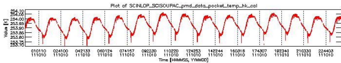
sciamachy_daily_report_level0_KSPT_L0_4504_N_20111010_3.PNG
