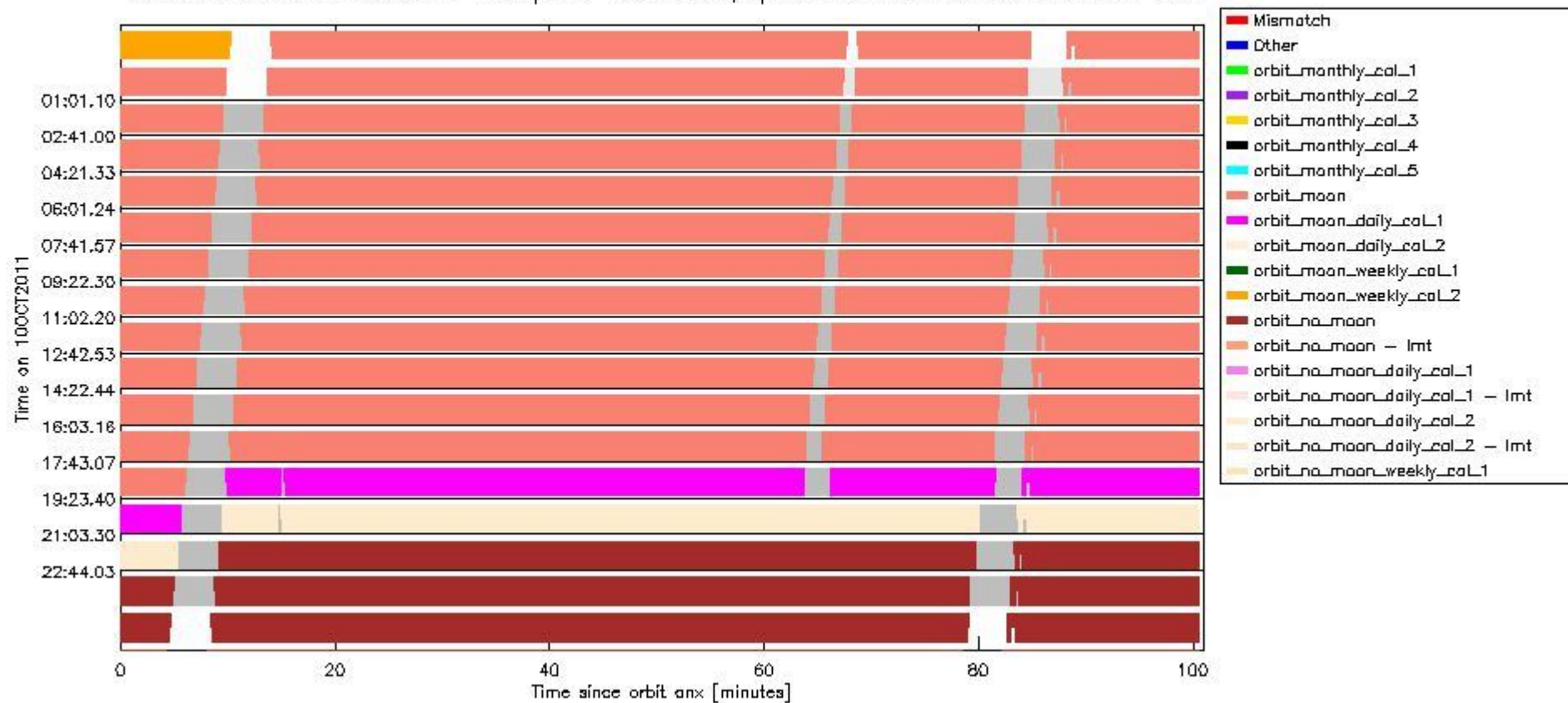
sciamachy_daily_report_level0_KSPT_L0_4504_N_20111010_6.PNG
