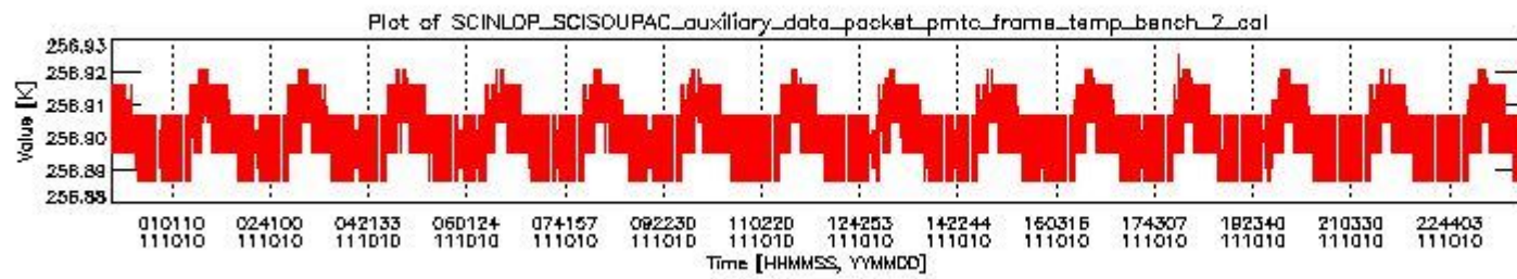
sciamachy_daily_report_level0_KSPT_L0_4504_N_20111010_1.PNG
