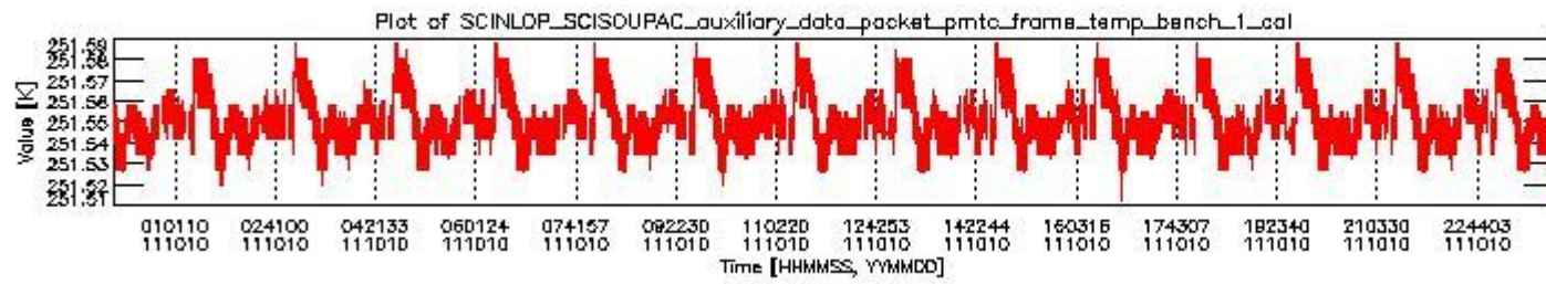
sciamachy_daily_report_level0_KSPT_L0_4504_N_20111010_0.PNG
