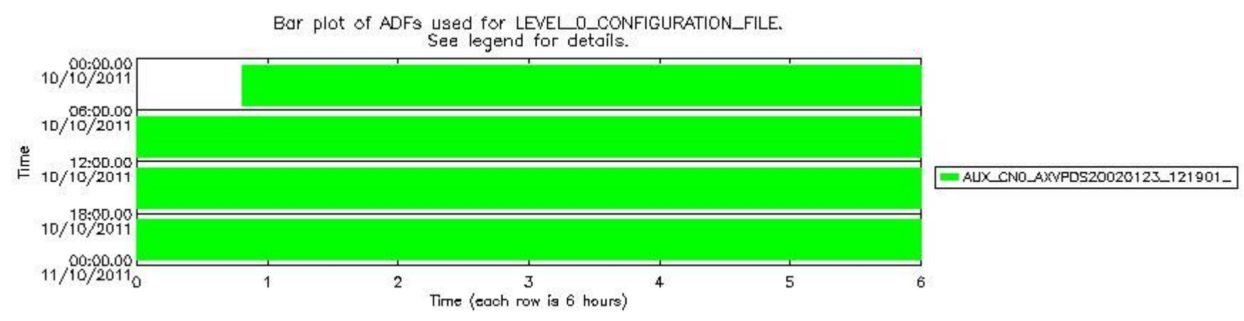
sciamachy_daily_report_level0_KSPT_L0_4504_N_20111010_7.PNG
